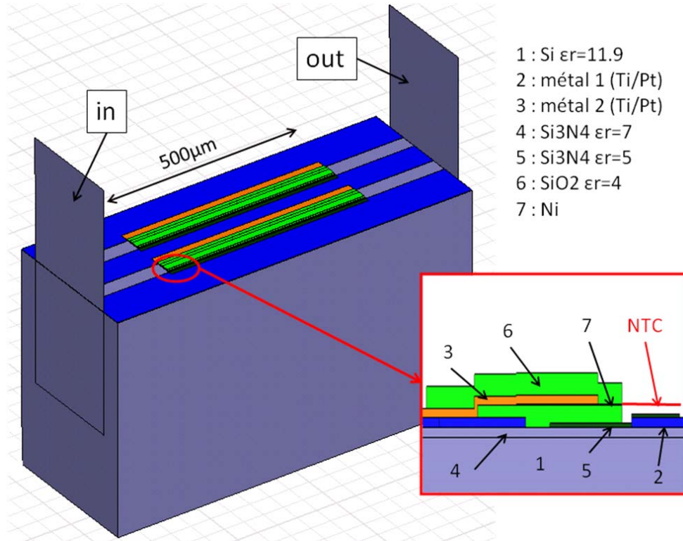
Figure 9 : Schéma de simulation et cross-section de la partie centrale. Le port d'entrée est « in », celui de sortie est « out ». Les différents matériaux utilisés sont ceux décrit dans la cross section, ainsi que l'espace de 2\mu\text{m} entre la couche de Ni et la piste de métallisation de la ligne de transmission.
