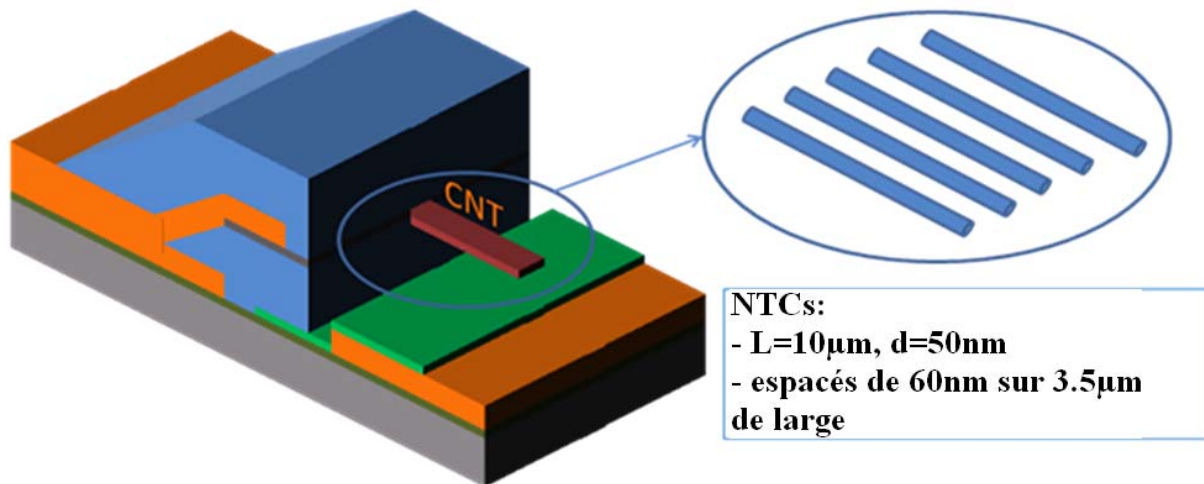
Figure 36 : Schématisation 3D d'une cellule unitaire de 20µm de largeur, elle est constituée de nanotubes espacés de 60 nm sur 3,5µm de large.
