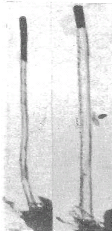
Figure 1 : image obtenue au MET par les russes Radushkevich et Lukyanovich lors de test sur du carbone. On voit clairement des fibres de carbone que l'on peut appeler nanotubes.
