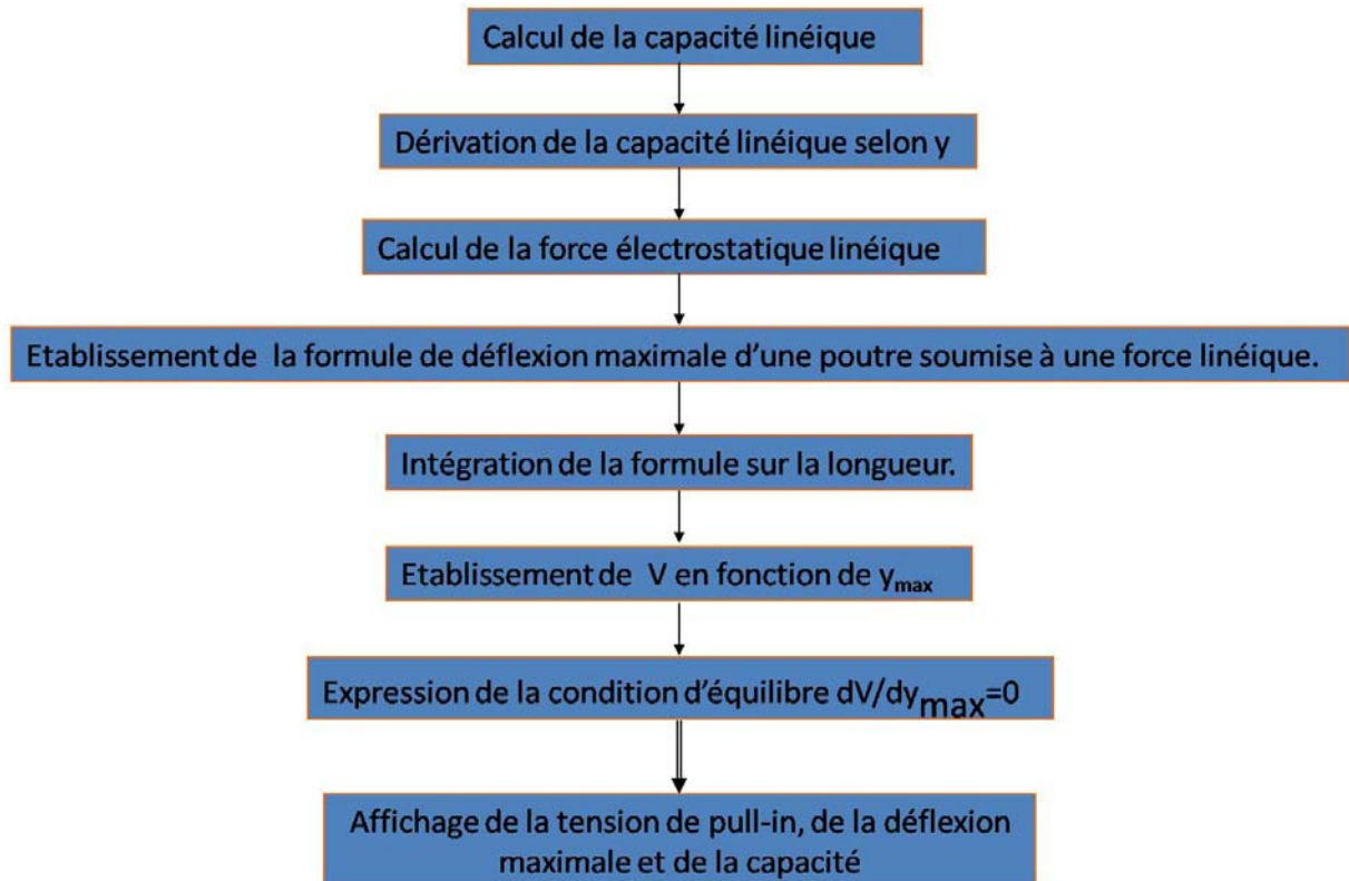
Figure 21 : Fonctionnement simplifié de notre programme pour trouver la déflexion et le pull-in d'un réseau de nanotube soumis à une force électrostatique.
