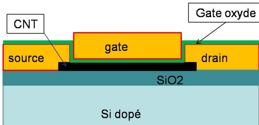
Figure 11 : cross section d'un CNFET, le nanotube, placé entre le drain et la source, joue le rôle du canal de conduction.
