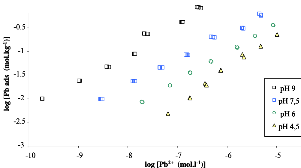
Figure 33 : Titrations par le plomb de la fraction HPOMT à 4 pH différents
