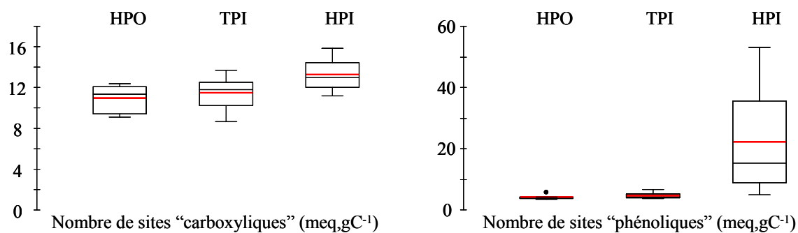
Figure 20 : Nombre de sites « carboxyliques » et « phénoliques » selon le type de fraction
