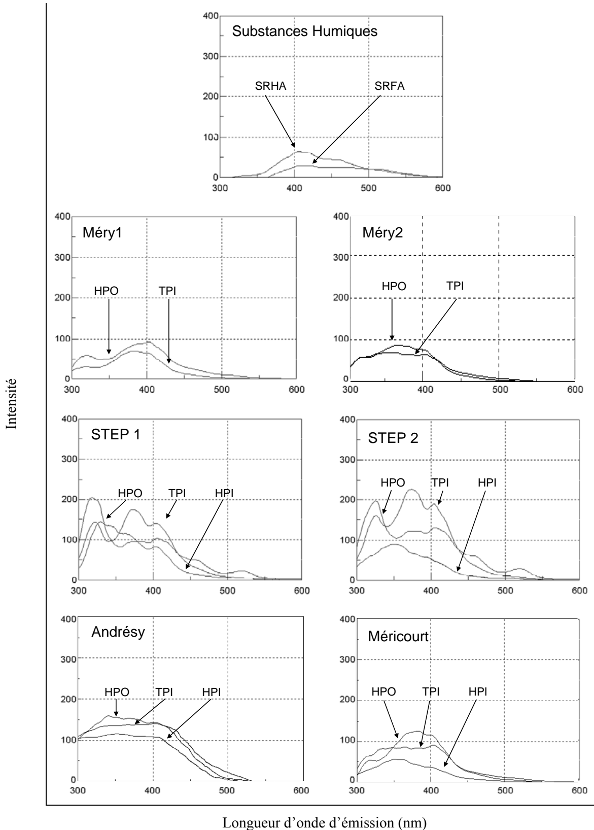
Figure 16 : Spectres de fluorescence synchrone des fractions étudiées ( \Delta\lambda = 40 \text{ nm} )
