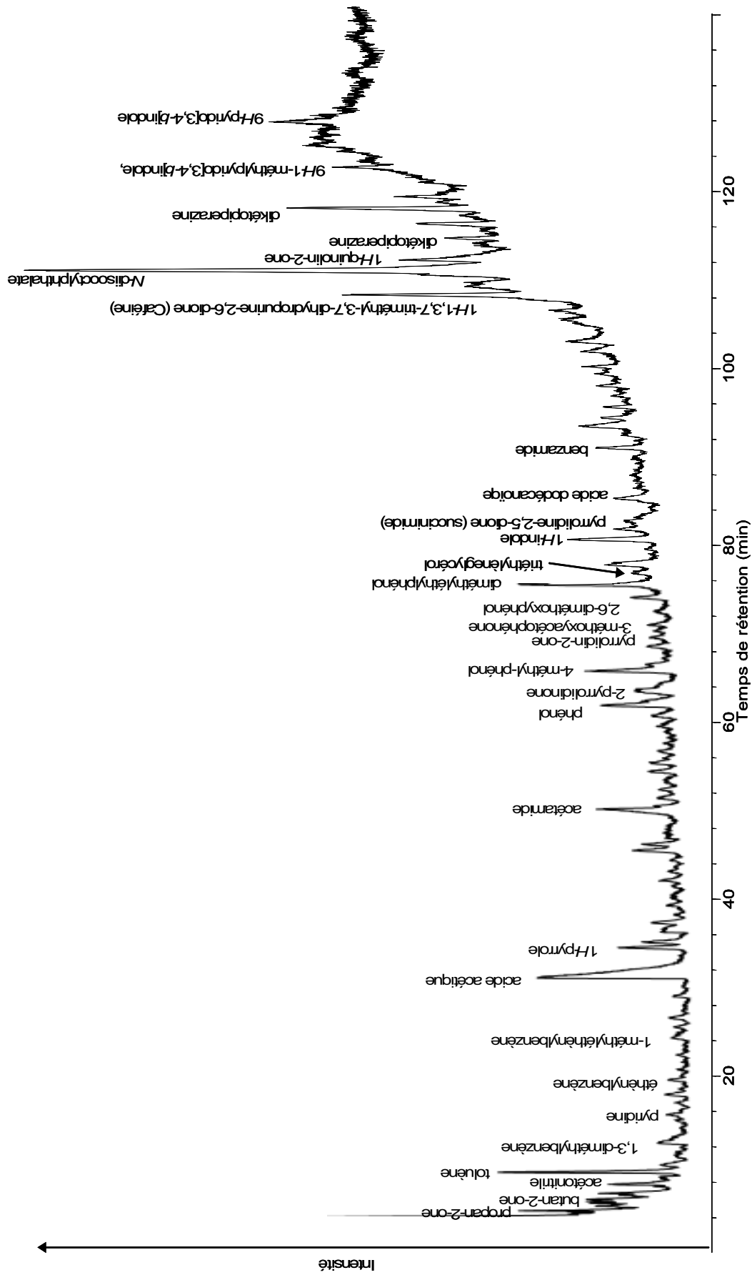
Figure 26 : Pyrogramme de la fraction HPOAI issue des effluents de la STEP Seine-Aval
