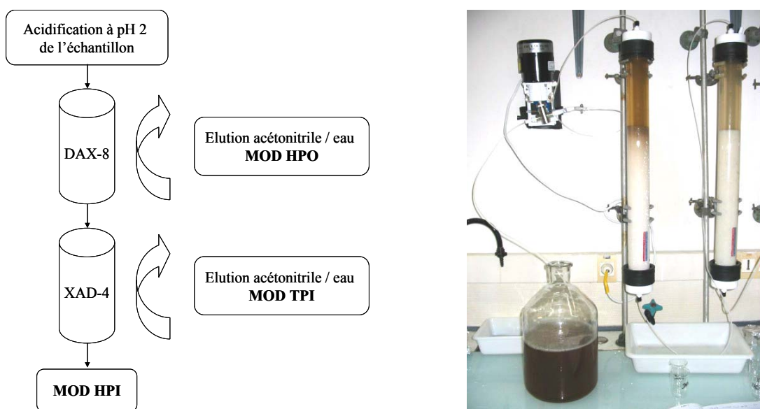
Figure 4 : Protocole de fractionnement sur résines DAX-8 et XAD-4
