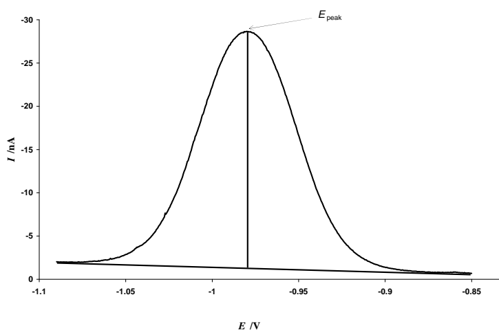
Figure 16 : Représentation d'une DPP réalisée avec une solution de Zn^{2+}
