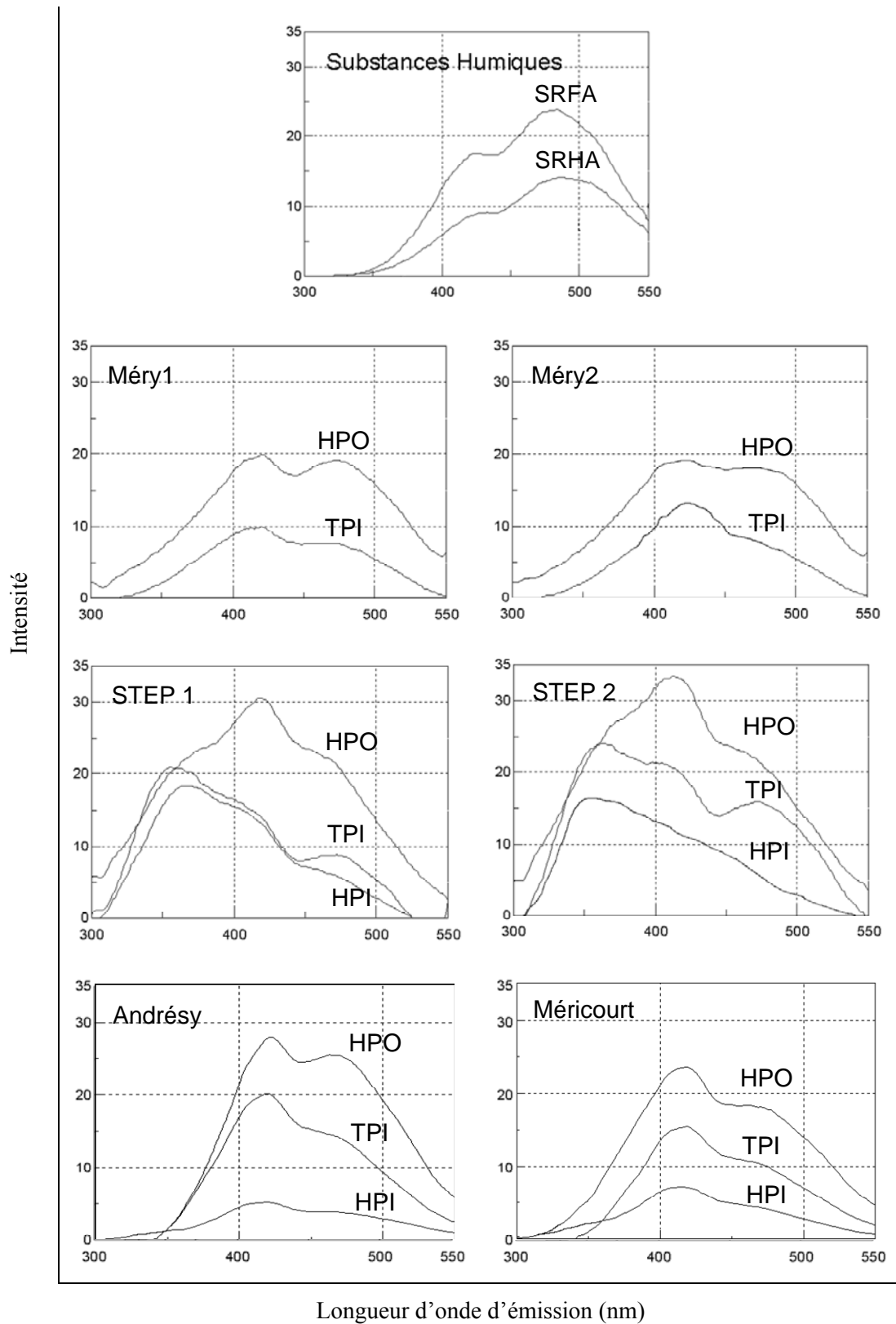
Figure 14 : Spectres de fluorescence d'émission simple ( \lambda_{ex}=280 nm) des fractions isolées (spectres corrigés par soustraction du spectre du solvant, ici l'eau déionisée ultrapure)
