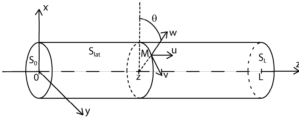
FIG. 2.1 – Schéma de la coque cylindrique et notations.
