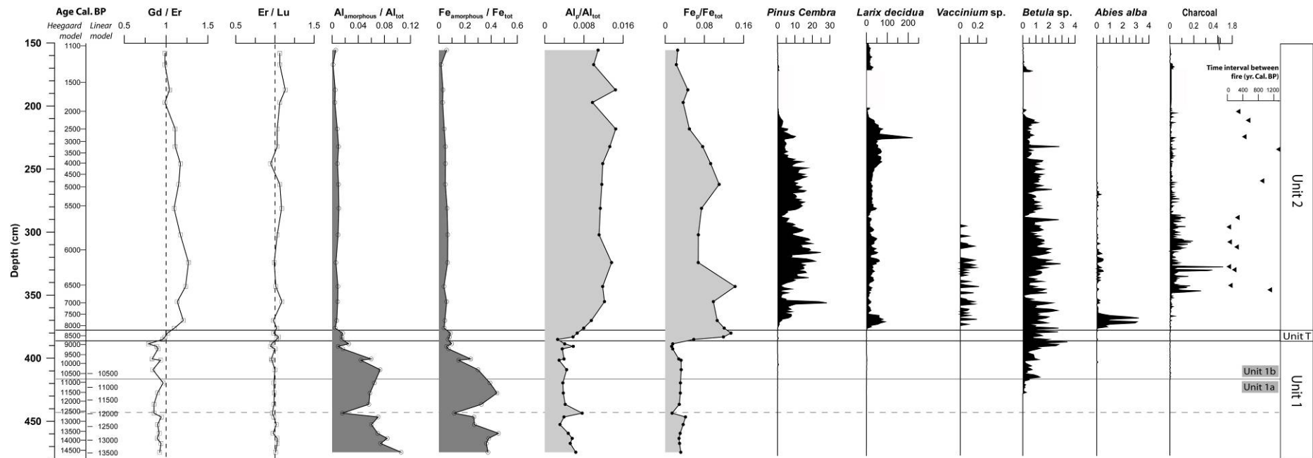
Figure 5.17 Présentation des différents paramètres géochimiques comparés aux influx de macrorestes (nb. cm-2yr.-1) de quelques espèces arboricoles et aux influx de charbons (mm2/cm2/yr). Gr/Er représente le fractionnement entre les REE intermédiaires et les REE lourdes et Er/Lu représente le fractionnement au sein des REE lourdes. Les triangles noirs représentent l'intervalle de temps entre les feux. La méthode statistique de reconstruction des feux est détaillée chapitre 4 (Mourier et al., submitted)
