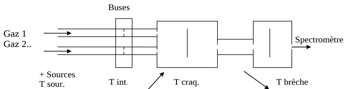
Figure I-12: réacteur possible à réaliser
