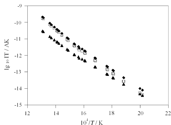
FIGURE 5. Effusion, diffusion and total contribution of \text{Cs}^+ measured ion when vaporizing \text{CsOH(s,l)} in a Pt–Rh effusion cell. \blacktriangle : \text{Cs}^+ diffusion. \square : \text{Cs}^+ effusion. \blacklozenge : \text{Cs}^+ effusion + diffusion (hypothetical).
