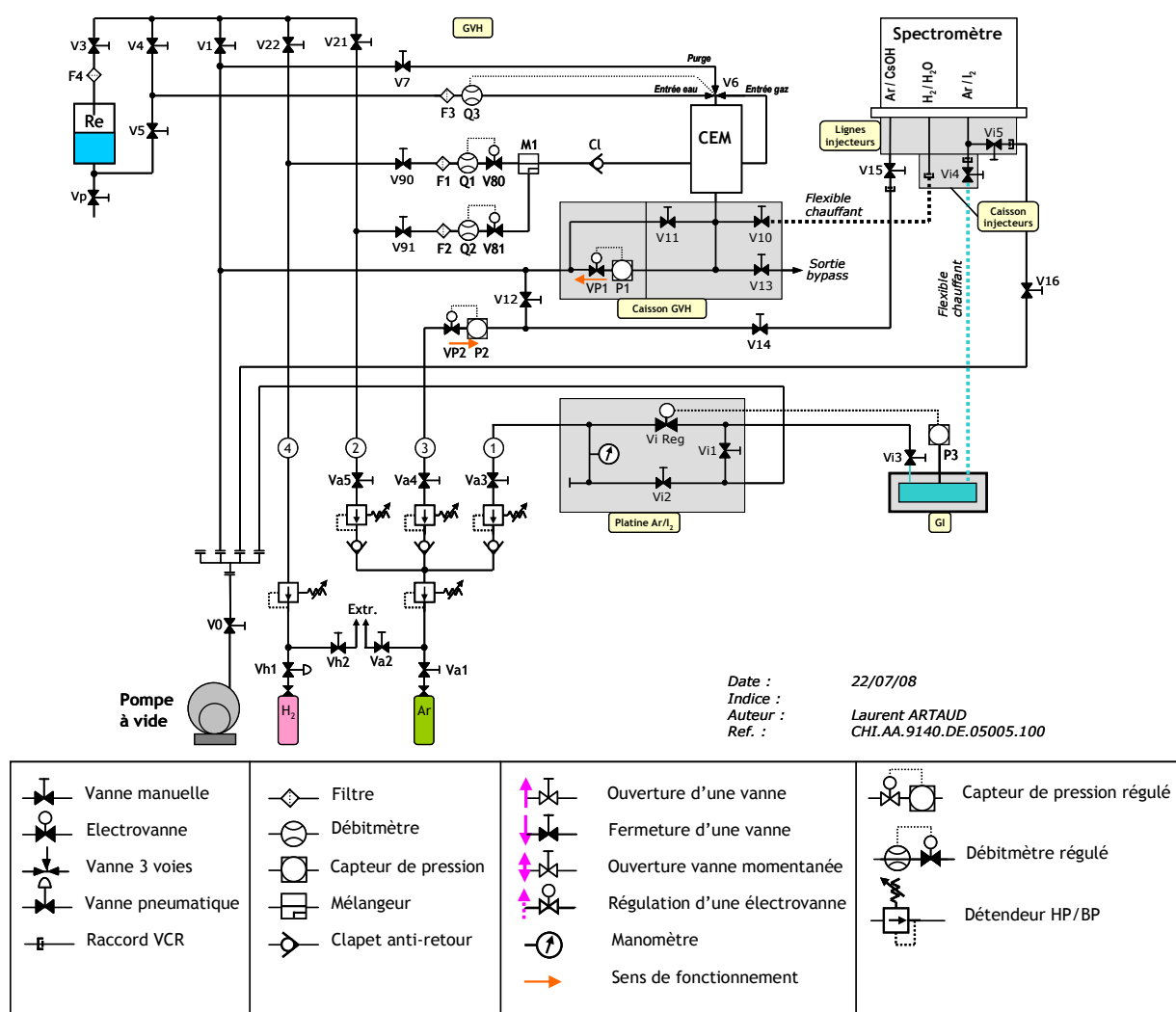
Figure I-A1: schéma de principe du circuit Bronkhorst pour l'injection des gaz \text{H}_2/\text{H}_2\text{O}/\text{Ar} .
