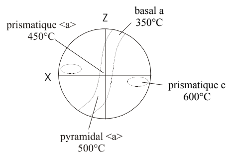
Figure 84. Différents systèmes de glissement du quartz mesurés au moyen des orientations préférentielles d'axes c (= [0001]) (projection stéréographique de Schmidt, hémisphère inférieur).
