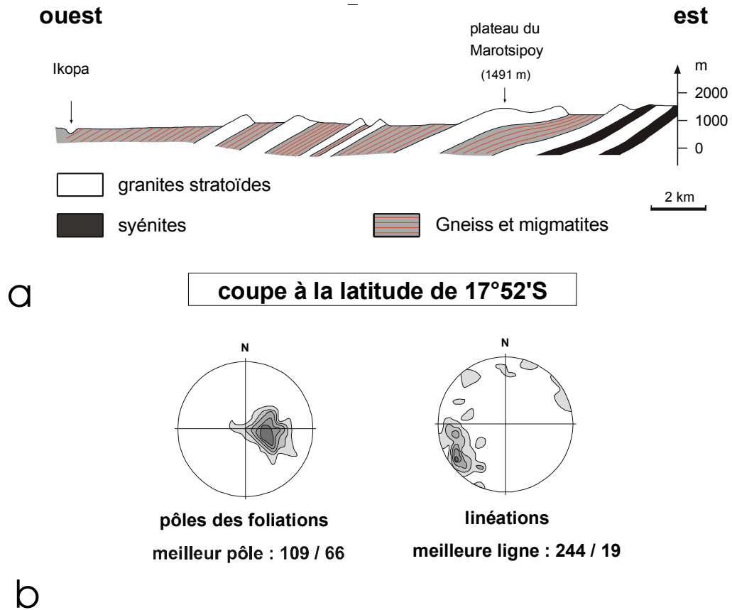
Figure 5. La série stratoïde au nord d'Antananarivo : a- coupe générale ; b- diagramme de projections (hémisphère inférieure) des pôles des foliations et des linéations magnétiques (d'après Nédélec et al., 1994).
