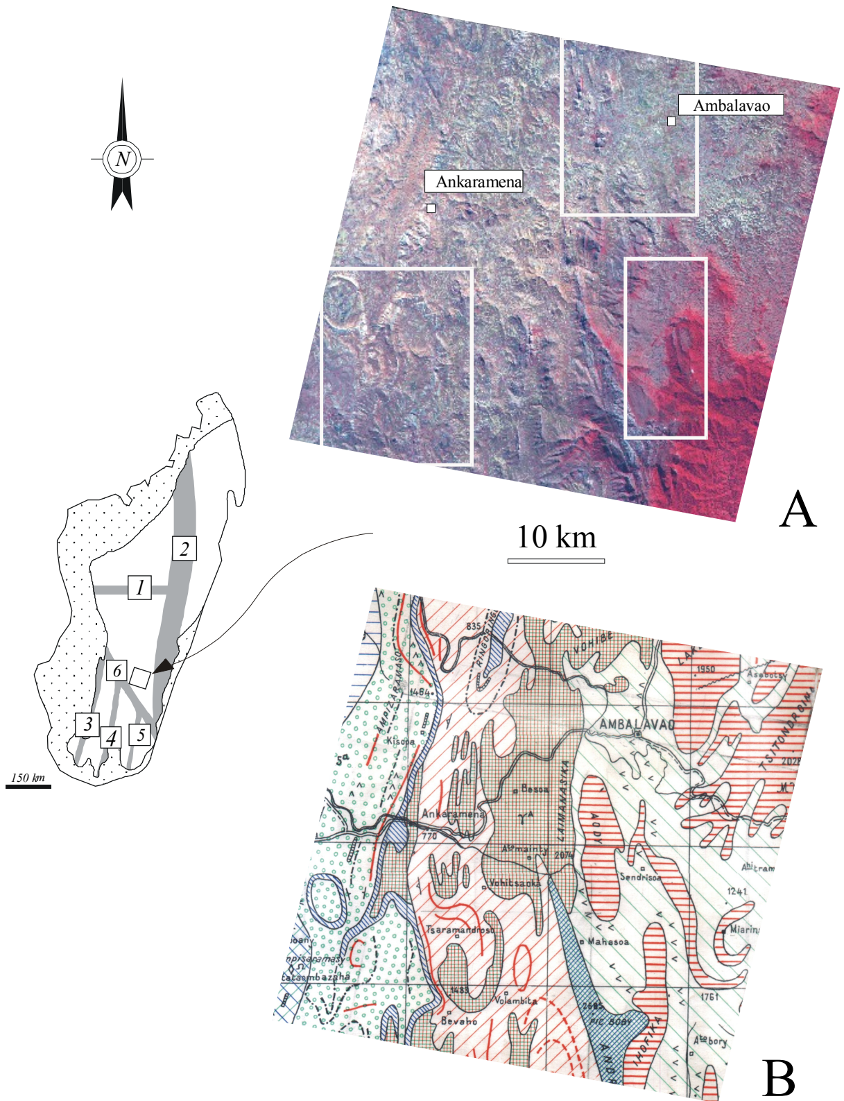
Figure 24. A- Situation de l'image brute SPOT multispectrale 169-394 du 30 janvier par rapport aux principales structures cisailantes panafricaines. Cisaillements de : 1- Antananarivo ; 2- Angavo ; 3- Ampanihy ; 4- Ampandrandava ; 5- Tranomaro ; 6- Bongolava-Ranotsara. On voit déjà apparaître distinctement les séries quartzitiques (à l'ouest en blanc) la chaîne de l'Andringitra (au sud-est en bleu foncé) et la partie terminale de la forêt orientale (en rouge). En encadré, les secteurs-clés étudiés dans ce chapitre. B- même secteur d'après la carte géologique (feuille de Fianarantsoa au 1/500000 ème ).
