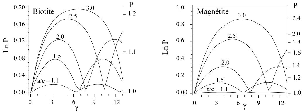
Figure 22. Simulation numérique de l'intensité de la fabrique magnétique (P ou lnP) d'une population de marqueurs magnétiques (biotite et magnétite) d'anisotropie intrinsèque de forme a/c. a- L'anisotropie magnétocristalline des cristaux de biotite ne dépasse pas 1,3 quel que soit le rapport de forme des grains considérés. b- L'anisotropie magnétocristalline des grains de magnétite est directement liée au rapport a/c. (in Hrouda, 1993).
