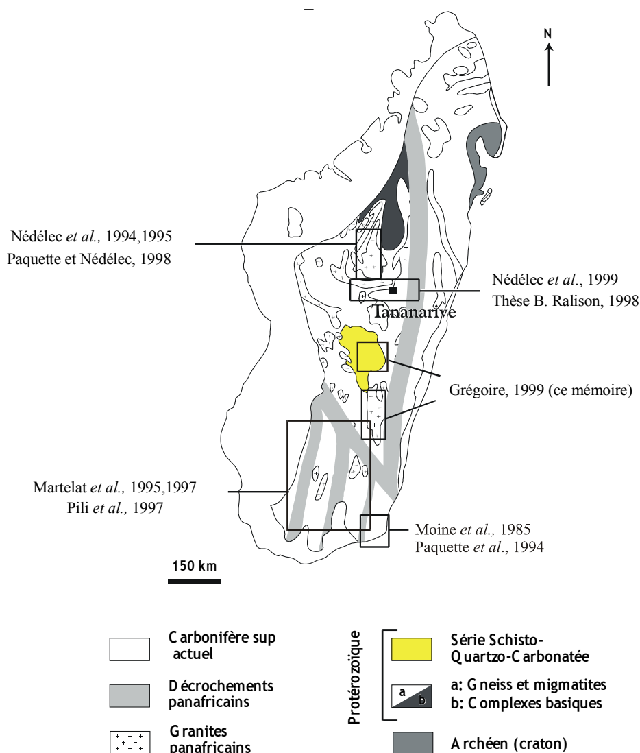
Figure 10. Situation des secteurs d'étude par rapport aux grandes structures panafricaines Les secteurs récemment étudiés par les équipes françaises (Toulouse, Lyon, Clermont-Ferrand) sont aussi indiqués.
