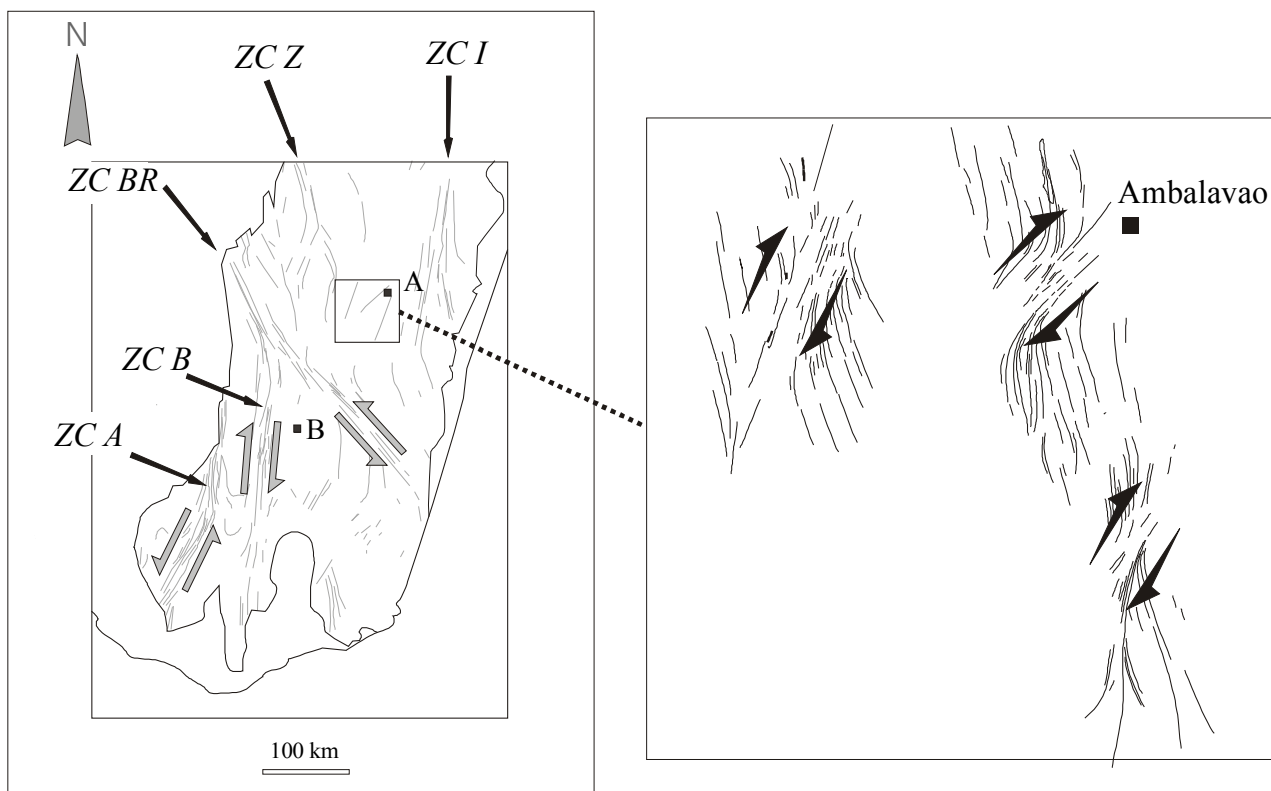
Figure 43. Situation des cisaillements détectés dans la région d'Ambalavao par rapport au cadre structural général du proposé par Martelat (1998). On a reporté les zones de cisaillement (ZC) de : I : Ifanadiana ; Z : Zazafotsy ; BR : Bongolava-Ranotsara ; B : Beraketa ; A : Ampanihy. Le secteur d'Ambalavao est caractérisé par des zones de cisaillement kilométriques synchrones du champ de déformation D2.
