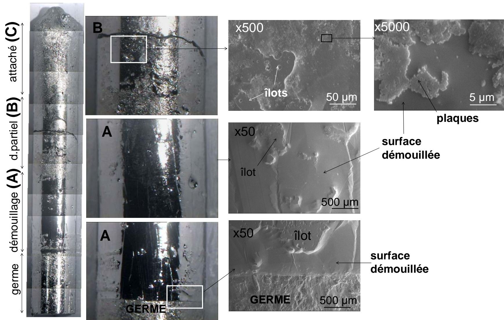
Figure III-3-4. Photographie du lingot GaSb sous air (M15) séparé en quatre zones: le germe, une zone de démoillage stable avec une surface lisse, du démoillage partiel avec une surface rugueuse/lisse et la présence de plaques (contamination), et enfin une zone de croissance attachée.
