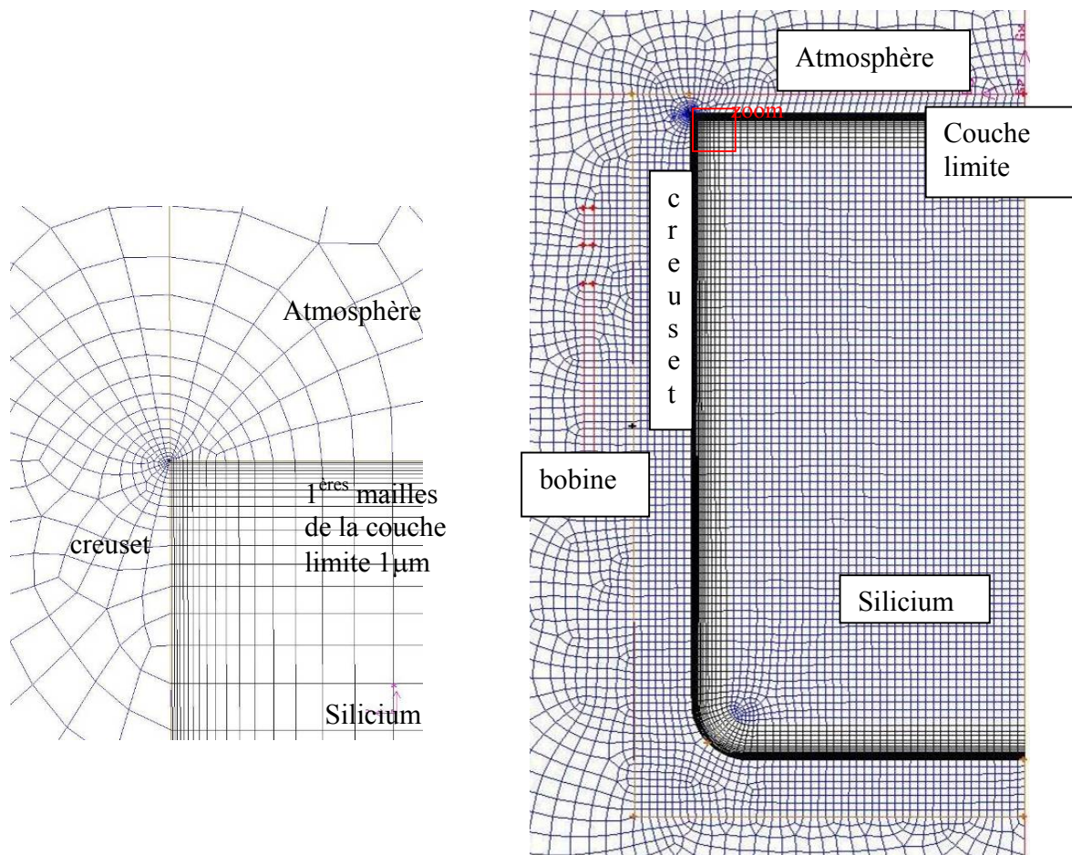
Figure V-13. maillage de la structure utilisé pour les simulations.
