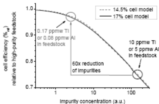
Figure III-5. Effet d'une contamination en aluminium et en titane sur le rendement des cellules photovoltaïques [26].
