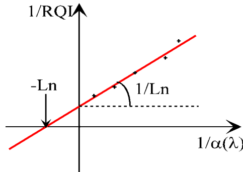
Figure C-4. Détermination graphique de la longueur de diffusion.
