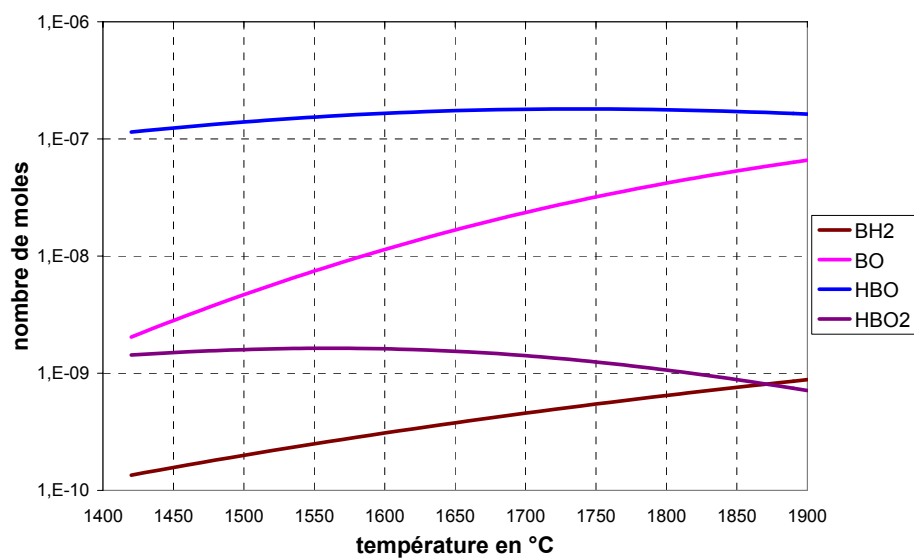
Figure IV-20. Calcul thermodynamique de la forme chimique du bore ( 700 Si + 1 Ar + 0.0085 O_2 + 0.025 H_2 + 0.007 B ).
