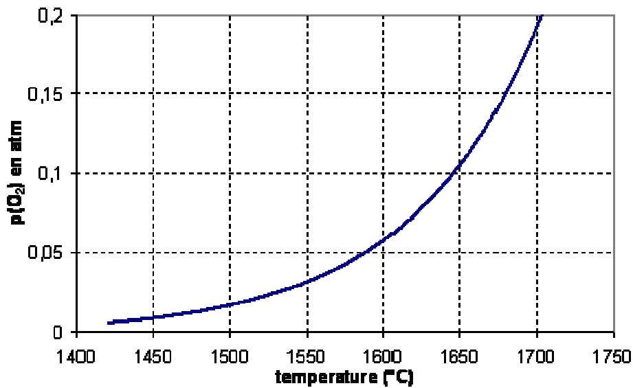
Figure IV-19. Seuil d'apparition de la couche de SiO_2 en fonction de la température ( 700 Si + 1 Ar + <A> O_2 ).
