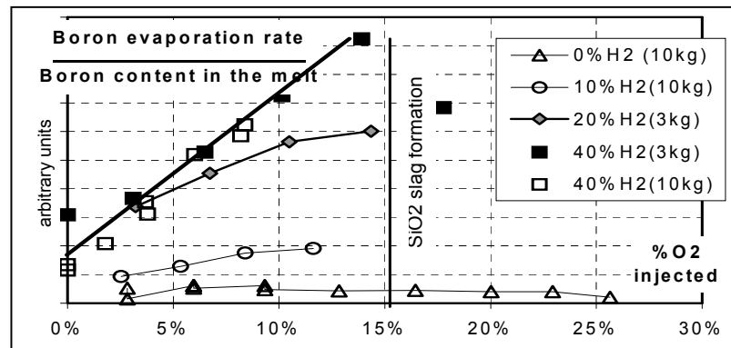
Figure IV-28. H 2 /O 2 effet sur l'évaporation du bore [81].
