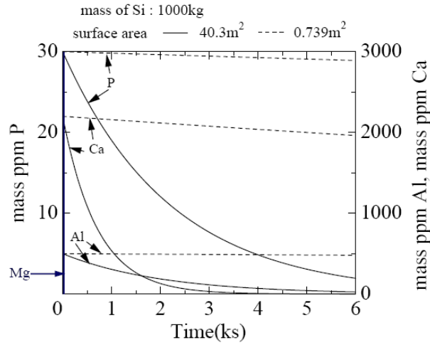
Figure IV-3. Relation entre le temps de traitement sous vide et la concentration en phosphore, aluminium et calcium pour un silicium calculé à 1823K [49].
