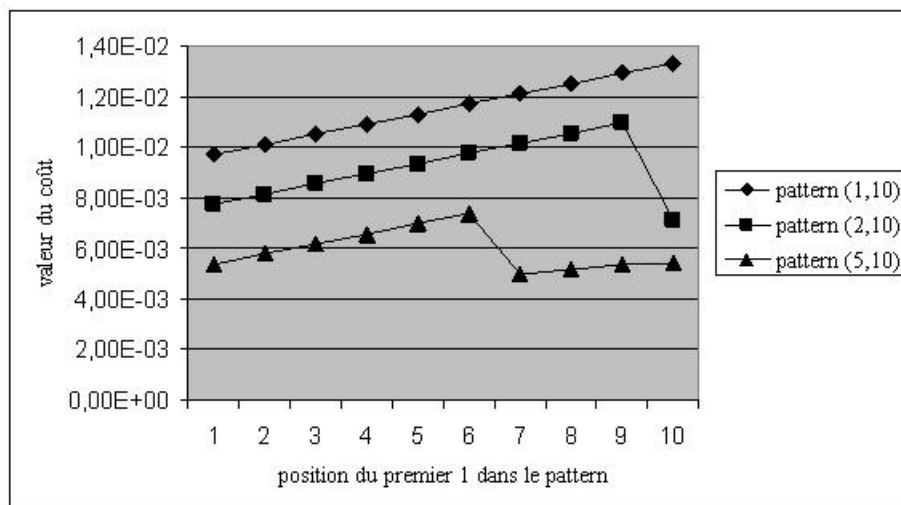
FIGURE 4.5 – Coûts obtenus pour les pattern (1, 10) , (2, 10) et (5, 10) en fonction de la synchronisation de demande de changement de consigne par rapport au premier échantillon accepté de la suite \Pi . Les pattern (m, 10) considérés comprennent tous une suite de 10 - m 1 consécutifs.
