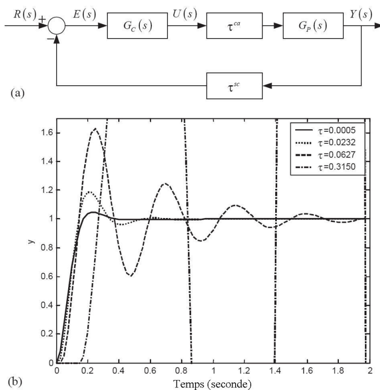
FIGURE 1.9 – La dégradation de performance induit par le délai. (a) la boucle de contrôle avec délai. (b) les réponse y à un échelon ( y_{référence} = 1 ) avec différents délais, où \tau_{cc} = \tau_{ca} = \frac{\tau}{2} .
