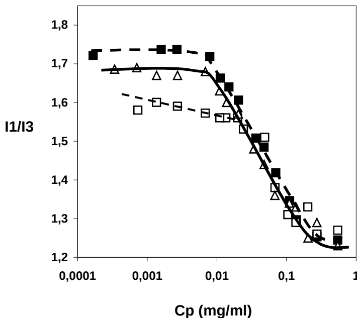
Figure III.1.5 : Tracé de I1/I3 en fonction du log de la concentration en PAA_{135}\text{-}b\text{-}PS_{17}
