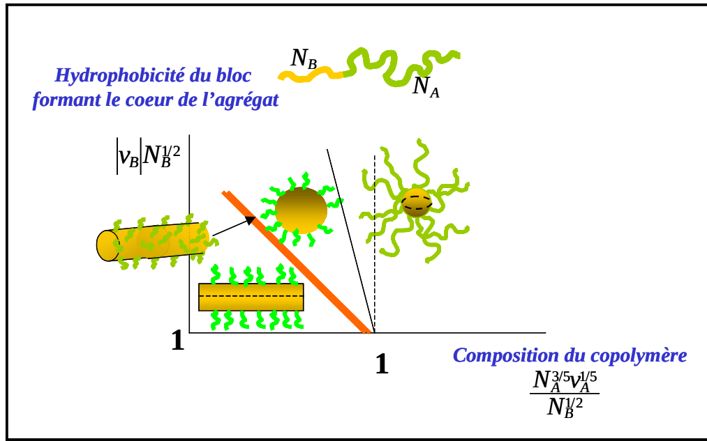
Figure III.1.2 : Diagramme de phase d'agrégats de copolymères di-blocs
