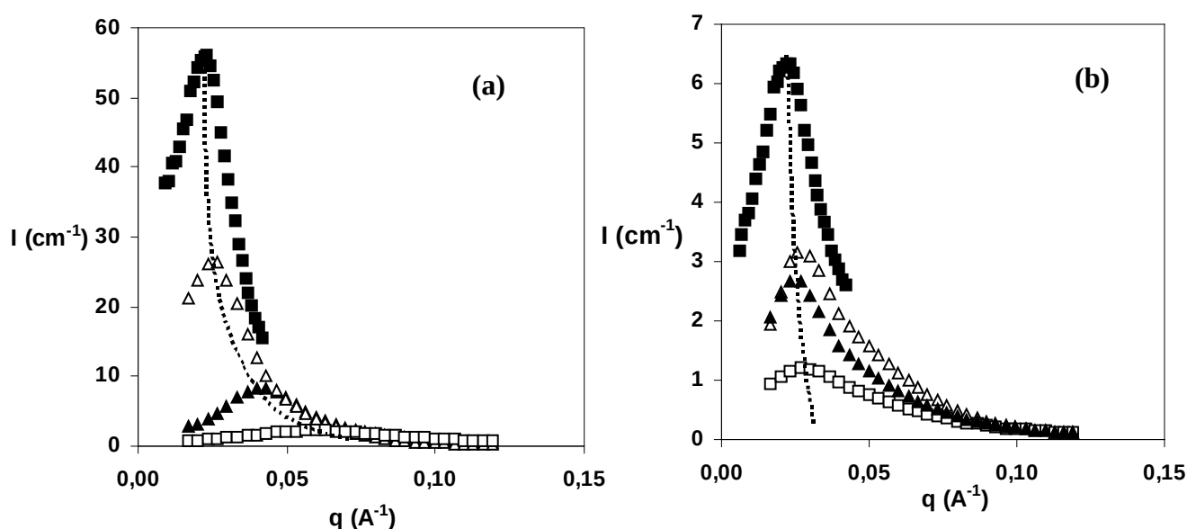
Figure IV.2.1 : Diffusion de neutrons aux petits angles de solutions de a) PAA 75 - b -(PAA 72 - grad -PS 35 ) et b) PAA 106 - b -(PAA 37 - grad -PS 10 ) (sans sel) à C_p=100\text{mg/mL} : ■ pH=3,5, △ pH=4,5, ▲ pH=5,5 et □ pH=7
