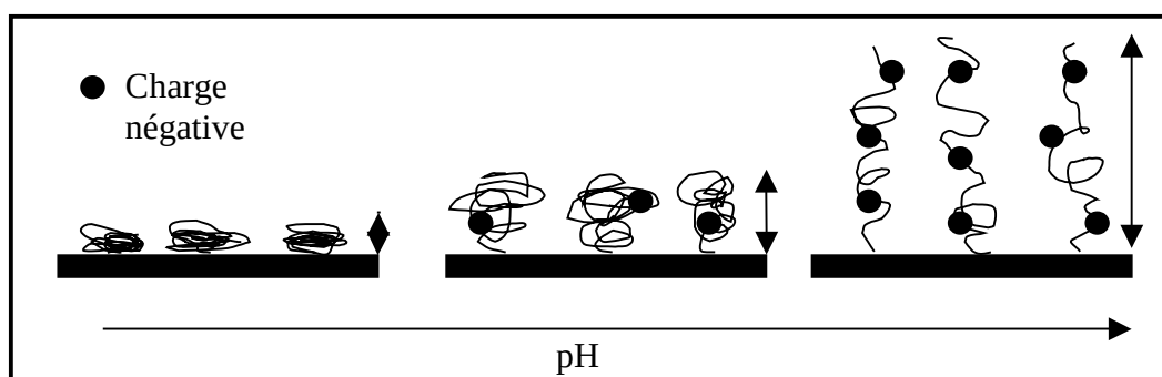
Schéma I.2.1 : Schématisation de l'influence du pH sur la couche de PAA greffé
