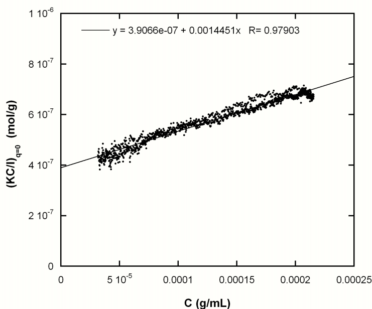
Figure III.3.2 : Traitement Zimm-Debye
