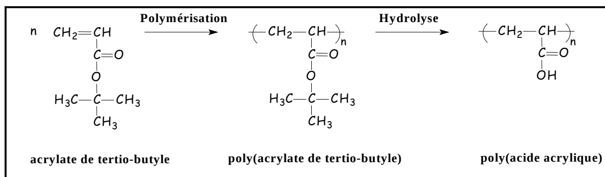
Schéma II.3.1 : Voie « indirecte » de synthèse du poly(acide acrylique) par post-modification du poly(acrylate de tertio -butyle)
