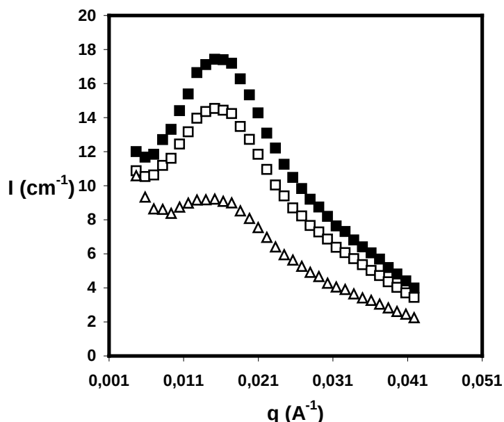
Figure III.2.3 : Diffusion de neutrons aux petits angles de solution de PAA 135 -b-PS 17 à 100 mg/mL (sans sel): \blacksquare pH=9, \square pH=6 et \triangle pH=4
