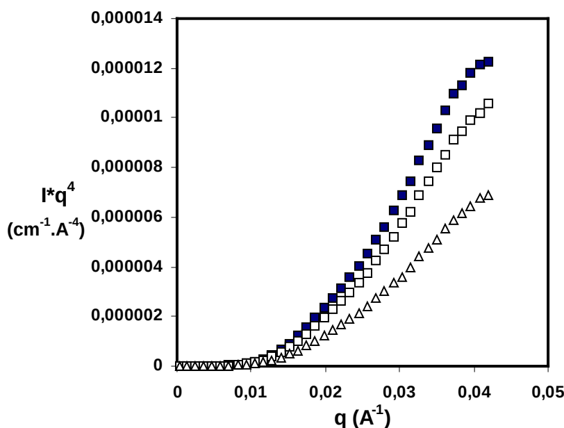
Figure III.2.4 : Tracé I \cdot q^4 en fonction du vecteur de diffusion q pour une solution de PAA_{135} - b - PS_{17} à 100 mg/mL (sans sel): ■ pH=9, □ pH=6 et △ pH=4
