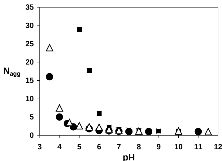
Figure IV.3.2 : Nombre d'agrégation en fonction du pH pour des solutions de PAA 75 -b-(PAA 72 -grad-PS 35 ) en présence de 0,15 mol/L de NaCl et à ■ C_p = 5 \text{ mg/mL} , \triangle C_p = 0,1 \text{ mg/mL} et \bullet C_p = 0,05 \text{ mg/mL}
