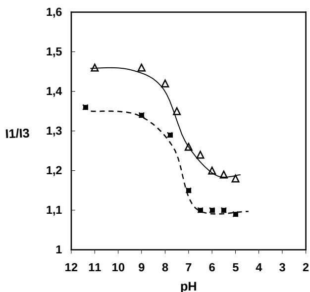
Figure IV.2.1 : Tracé de I_1/I_3 en fonction du pH pour une concentration en ■ PAA_{75}-b-(PAA_{72}-grad-PS_{35}) et △ PAA_{106}-b-(PAA_{37}-grad-PS_{10}) de 1 mg/mL (sans sel)
