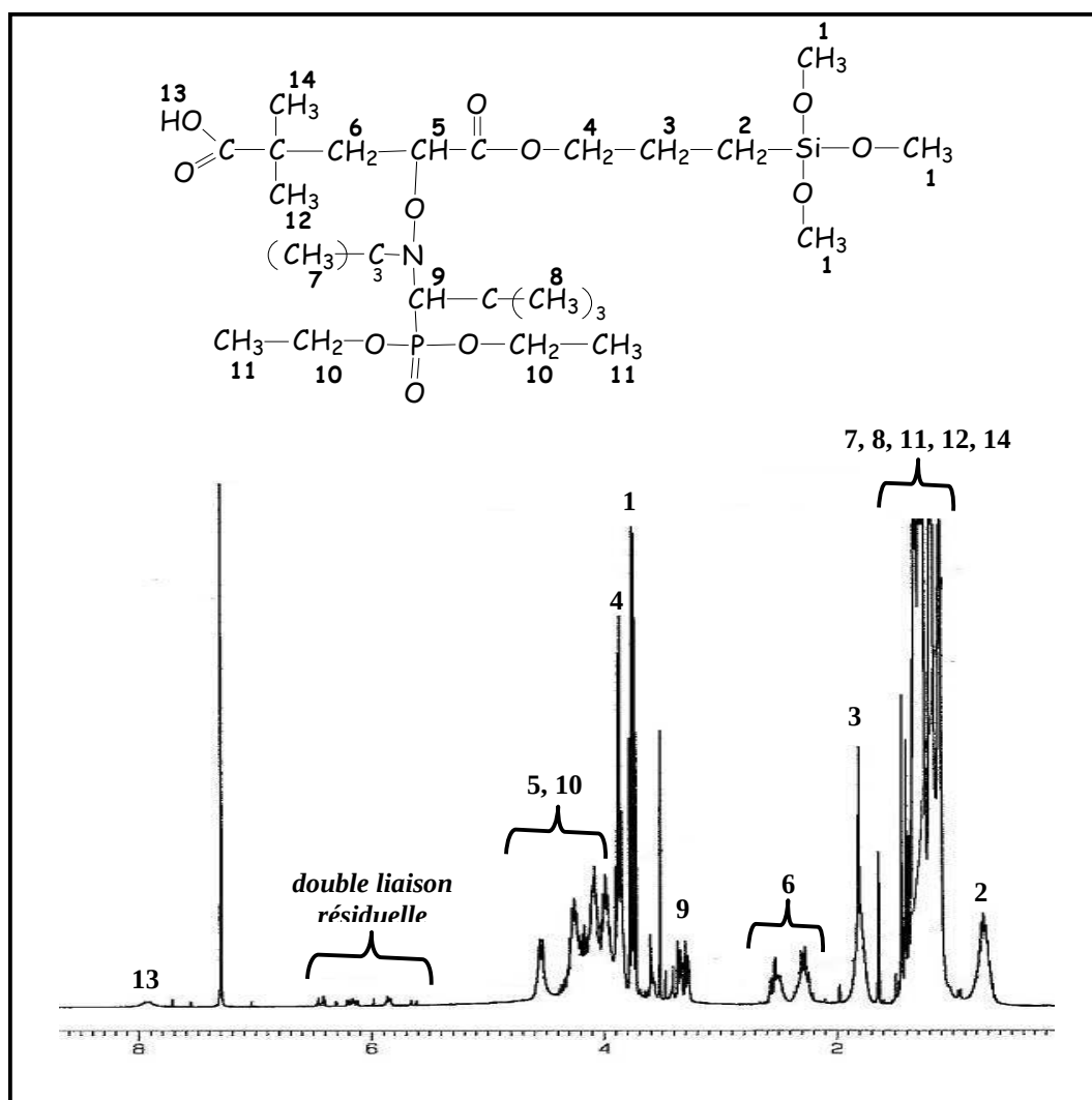
Figure II.2.4 : RMN ^1\text{H} après réaction entre la MAMA et la TMSPA
