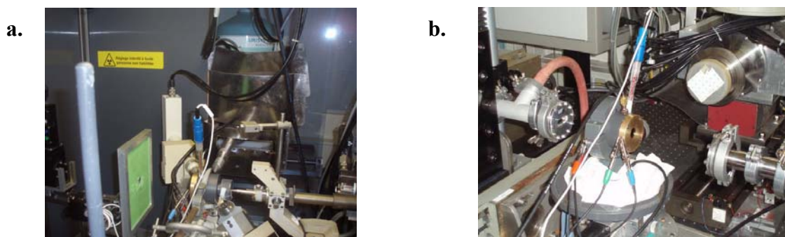
Figure 2.23 : Montage de la cellule sur : a. l'anode tournante du Laboratoire Pierre Süe ; b. la ligne FAME, ESRF.
