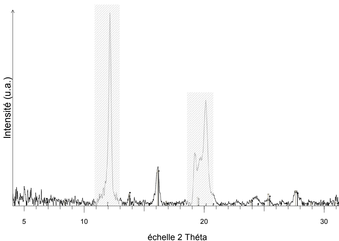
Figure 4.48 : Diffractogramme de l'échantillon R'L3 ( \text{Fe}(\text{OH})_2 + \epsilon \text{Fe}_3\text{O}_4 ) ré-oxydé à pH = 9. Comparaison avec les fiches JCPDF de la maghémite (en noir, PDF n°39-1346) et de la magnétite (en gris, PDF n°19-0629). Les zones grisées correspondent au graphite ( \lambda = 0,070932 \text{ nm} ).
