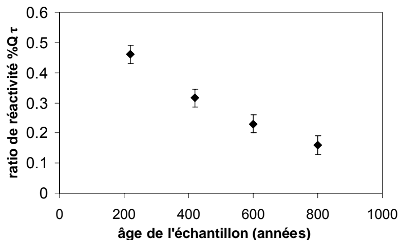
Figure 1.10 : Variation du coefficient de réactivité en réduction \%Q_\tau avec l'âge des échantillons étudiés : Aqueduc de Marly 220 ans, Clef de Voûte 420 ans, Cathédrale de Rouen 600 ans et Palais des Papes d'Avignon 800 ans [27].
