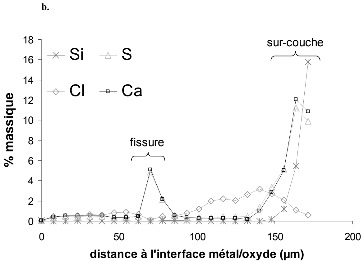
Figure 3.17 : a. Profil du fer et de l'oxygène et b. Profil du calcium, du soufre, du chlore et du silicium mesurés en MEB-EDS sur l'échantillon Am XXX N 100 en fonction de la distance par rapport à l'interface métal/produits de corrosion.
