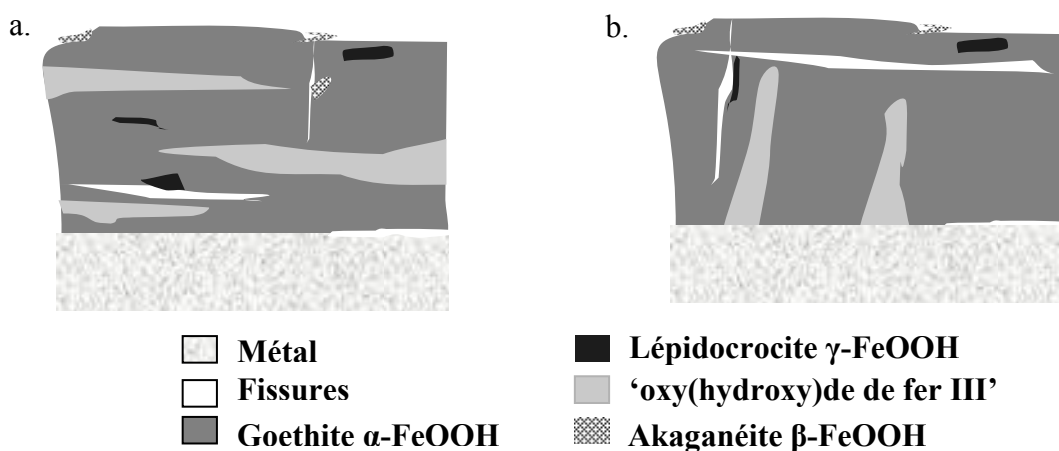
Figure 3.42 : Modélisation schématique de la morphologie de la couche de produits de corrosion développée sur le chaînage de la cathédrale d'Amiens. a. Dans le cas de marbrures de ferrihydrite/feroxyhyte et/ou maghémite non connectées au métal. b. Dans le cas de marbrures connectées au métal.
