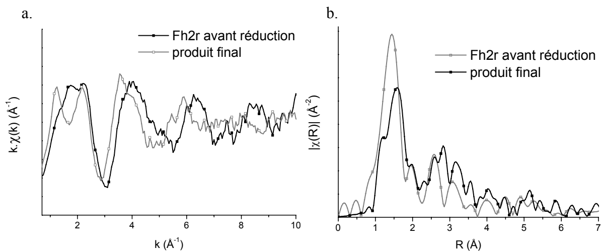
Figure 4.28 : a. Spectres EXAFS au seuil du fer et b. Transformées de Fourier d'un échantillon de ferrihydrite 2 raies avant et après réduction ( expérience RF1 ).
