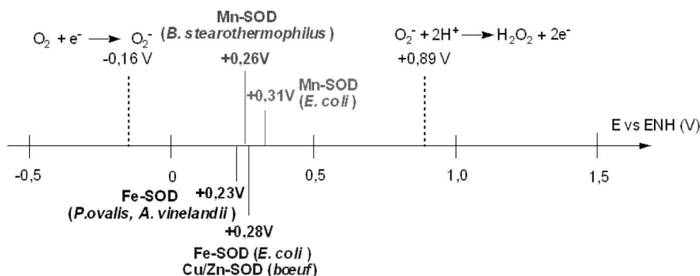
FIG. 4.1 – Potentiels redox des couples métalliques dans les SOD, comparés avec les potentiels redox d'oxydation et de réduction du superoxyde à pH=7, d'après Cabelli et al. [252] .
