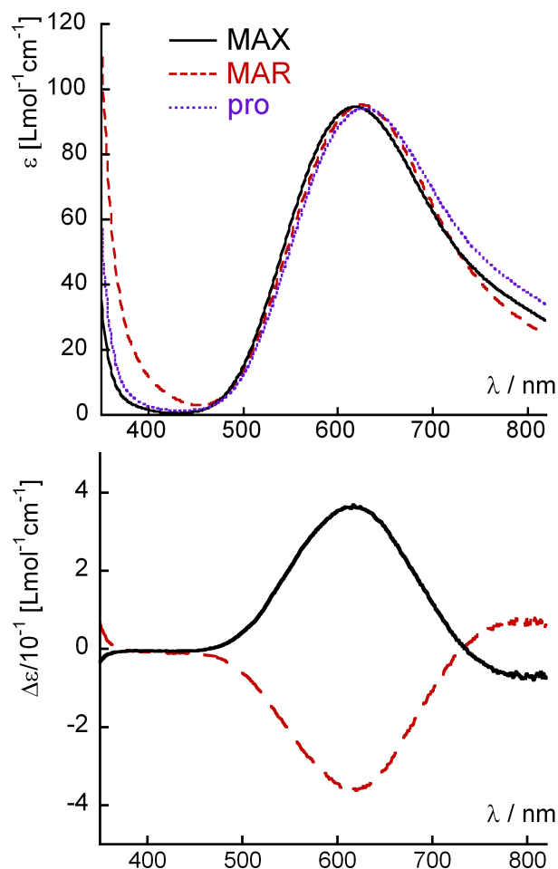
FIG. 3.15 – Spectres d'absorption dans le visible et de dichroïsme circulaire (pour les glycoligands) de solutions des complexes de \text{Cu(II)} de \text{MAXP}_3 , \text{MARP}_3 et \text{proP}_3 . Concentration : 10^{-2} \text{ mol L}^{-1} .
