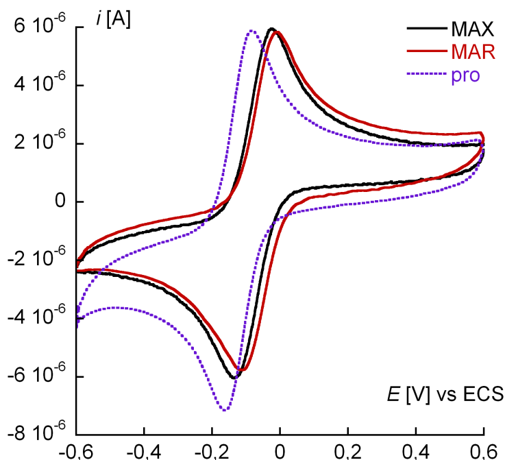
FIG. 3.13 – Voltammogrammes cycliques des solutions de complexes de Cu(II) de \text{MAXP}_3 , \text{MARP}_3 ou \text{proP}_3 . Solvant Ethanol/Acétone 2 : 1. Électrolyte support : \text{LiClO}_4 3,3 \times 10^{-2} mol \text{L}^{-1} . Concentrations de travail : [\text{Cu}(\text{MARP}_3)(\text{EtOH})](\text{PF}_6)_2 3,3 \times 10^{-4} mol \text{L}^{-1} ; [\text{Cu}(\text{MAXP}_3)](\text{PF}_6)_2 3,3 \times 10^{-4} mol \text{L}^{-1} ; [\text{Cu}(\text{proP}_3)](\text{PF}_6)_2 \cdot \frac{1}{2} \text{MeOH} 3,9 \times 10^{-4} mol \text{L}^{-1} . Vitesse de balayage 200 \text{mV s}^{-1} , cycle de balayage 0,2 V \rightarrow -0,6 V \rightarrow +0,6 V (répété 3 fois), les électrodes et appareils utilisés sont donnés dans la partie expérimentale. Les voltammogrammes ne présentent pas de variation sur les trois cycles de balayage. Les tracés montrés sont ceux mesurés lors du 3 ème cycle de balayage.
