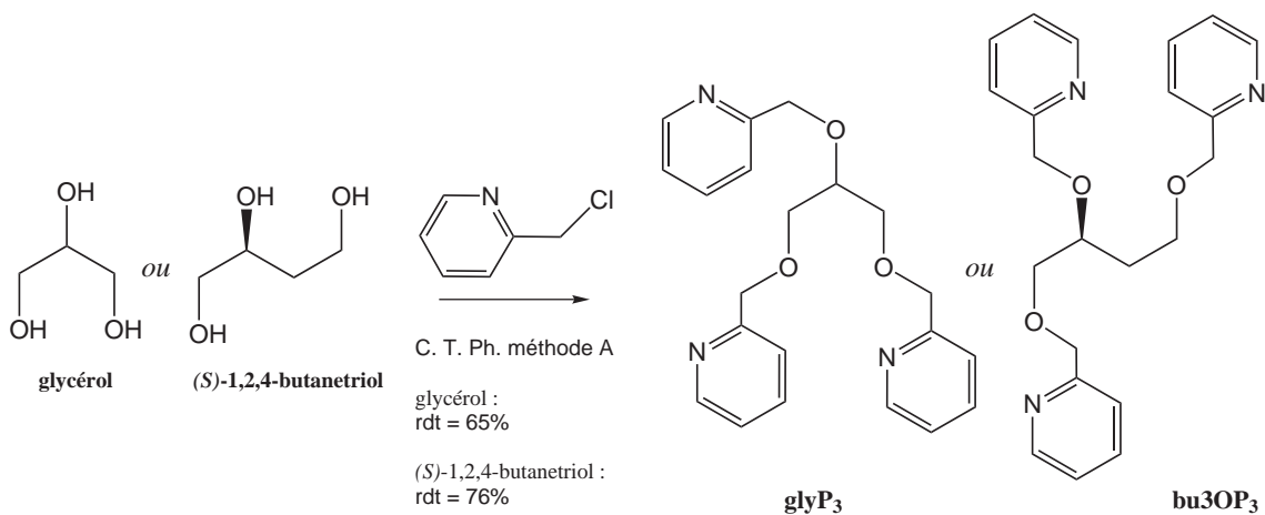
FIG. 2.6 – Synthèse de glyP 3 et bu3OP 3 : analogues acycliques des glycoligands triéther.
