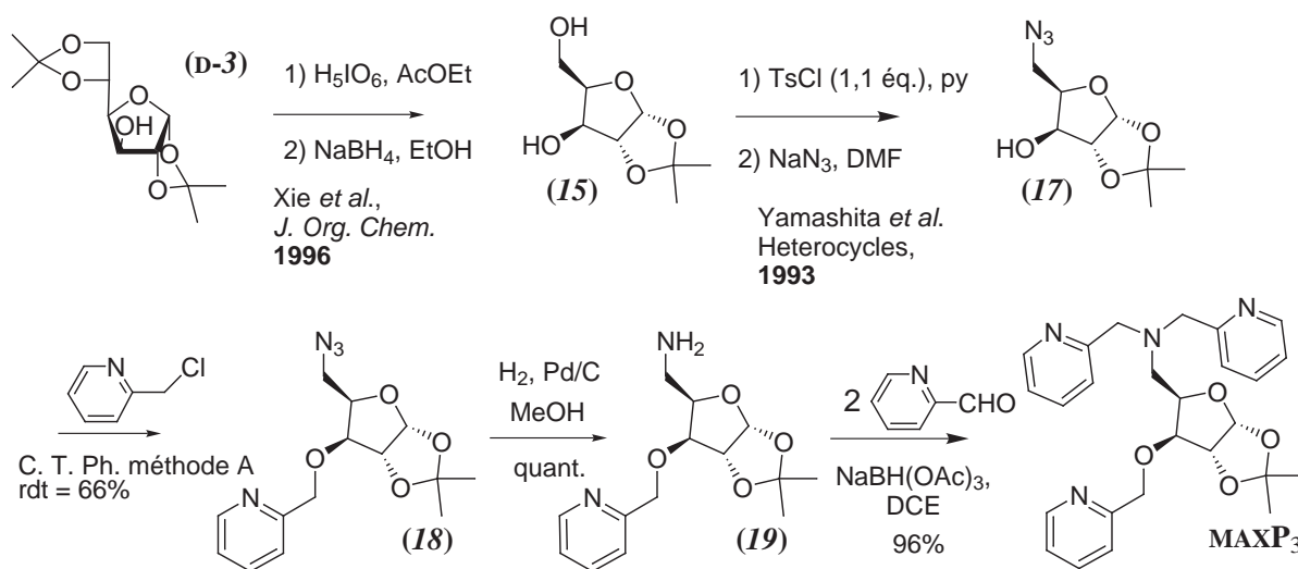
FIG. 3.7 – Synth\u00e8se de MAXP 3 .
