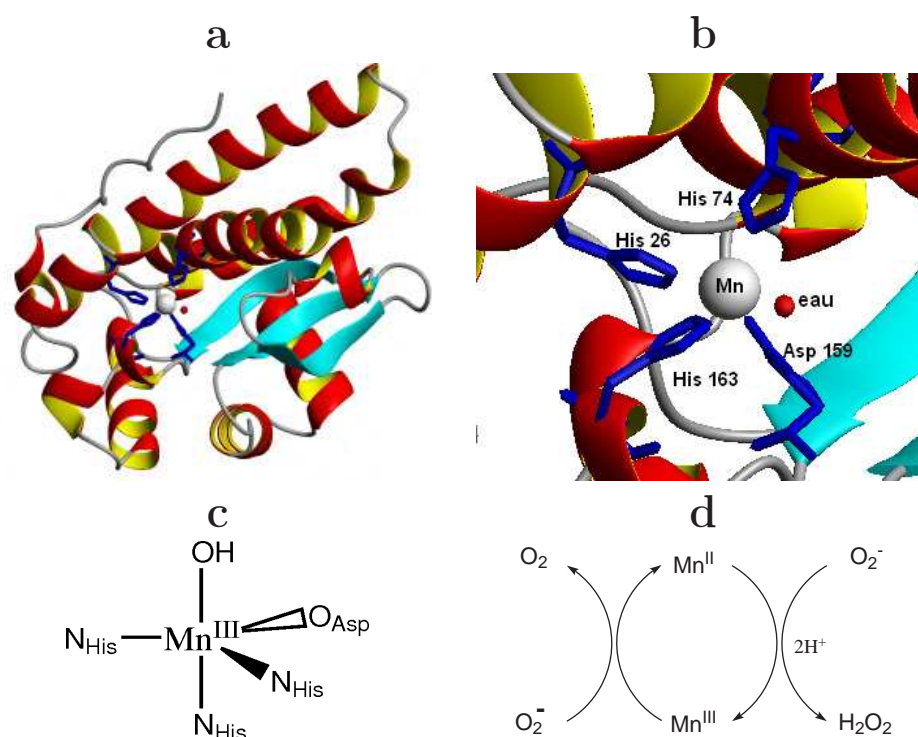
FIG. 4.2 – a : structure d'un monomère de la SOD à Mn mitochondriale humaine [254] . b : zoom sur le site actif. c : représentation schématique de la sphère de coordination. d : mécanisme catalytique simplifié.
