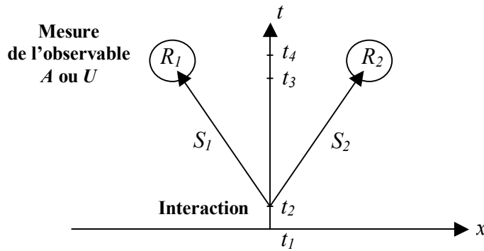
Figure 4.1 Schéma de l'expérience EPR
