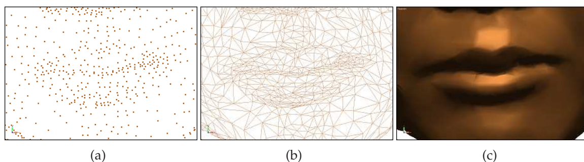
Figure 3.22 – Triangulation d'un nuage de point : (a) nuage de point ; (b) maillage obtenu par triangulation ; (c) rendu
