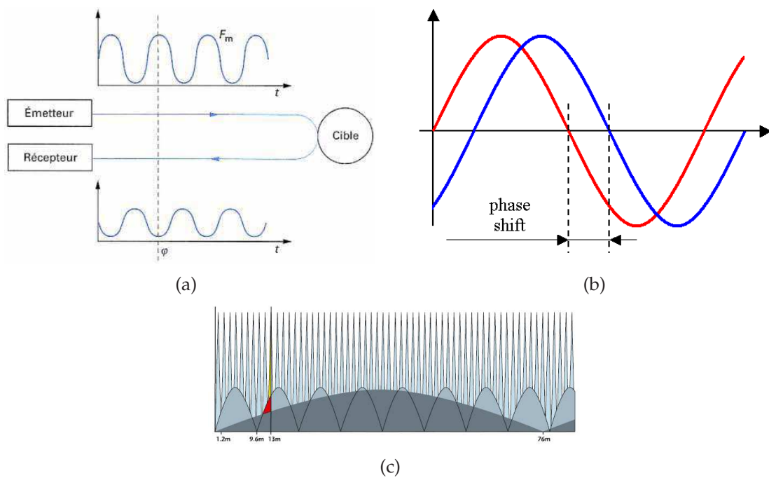
Figure 2.23 – Temps de vol à décalage de phase : (a-b) mesure du décalage ; (c) combinaison de plusieurs fréquences pour lever l'ambiguïté [Faro, 1983]
