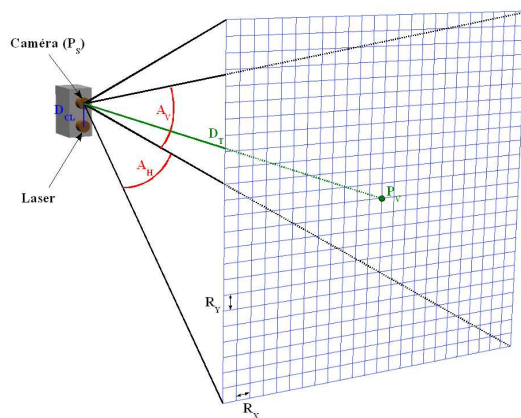
Figure 4.36 – Réglages initiaux : position scanner ( P_S ), position visée ( P_V ), résolution en X ( R_X ), résolution en Y ( R_Y ), angle horizontal ( A_H ), angle vertical ( A_V ), distance caméra-laser ( D_{CL} ), distance de travail ( D_T )
