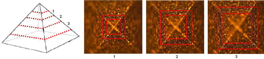
Figure 2.27 – Shape from Focus : objet à numériser et acquisitions à différentes altitudes, avec le système InfiniteFocus de Alicona
