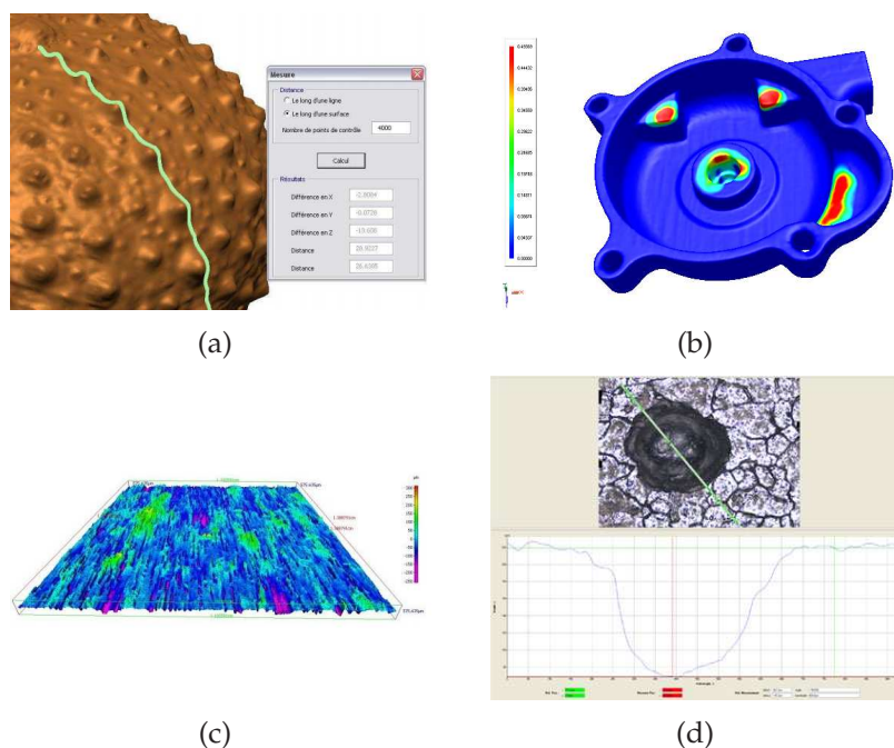
Figure 3.13 – Applications liées à l'analyse : (a) mesure dimensionnelle ; (b) carte de déviation ; (c) rugosité ; (d) mesure de profil
