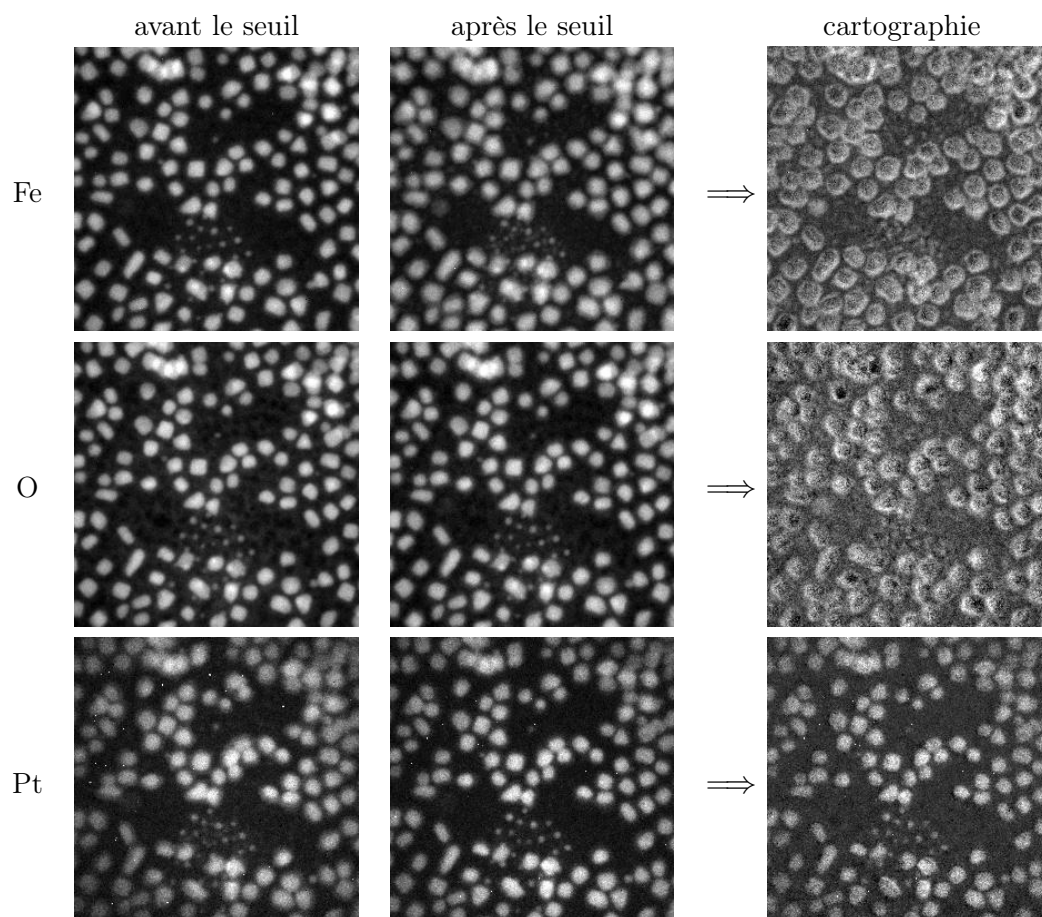
FIG. 6.10 – Images de nanoparticules de FePt, synthétisées avec le protocole \text{Fe}^0 \text{Pt}^{2+} dicytylether, filtrées en énergie avant et après les seuils du fer (710 eV), de l'oxygène (530 eV) et du platine (Pt 2192 eV). La taille de chacune des images est de 146 nm. Un profil radial de ces particules montre qualitativement la présence d'une coquille de 1 nm d'épaisseur contenant du fer et de l'oxygène autour d'un cœur riche en platine.
