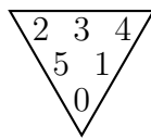
\Delta S_4
