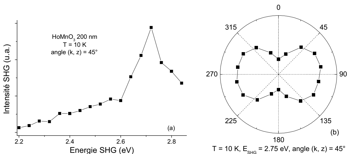
Figure 4.53 : intensité SHG en fonction (a) de l'énergie et (b) de l'angle entre le polariseur et l'analyseur, d'un film d' \text{HoMnO}_3 de 200 nm déposé à 850^\circ\text{C} , mesurée à 10 K avec un angle de 45^\circ entre k et z.
