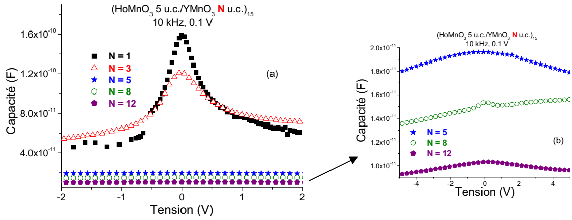
Figure 5.19 : (a) mesures C(V) de multicouches (\text{HoMnO}_3 \text{ 5 u.c./YMnO}_3 \text{ N u.c.})_{15} déposées sur Pt/Si à 825°C, effectuées sur des électrodes de surfaces 110 \times 110 \mu\text{m}^2 . (b) Agrandissement des courbes pour N = 5, 8 et 12.
