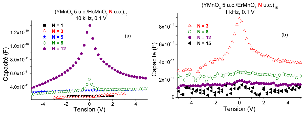
Figure 5.20 : mesures C(V) (a) de multicouches (\text{YMnO}_3 \text{ 5 u.c./HoMnO}_3 \text{ N u.c.})_{15} déposées sur Pt/Si à 825°C et (b) de multicouches (\text{YMnO}_3 \text{ 5 u.c./ErMnO}_3 \text{ N u.c.})_{15} déposées sur Pt/Si à 850°C - mesures effectuées sur des électrodes de surfaces 150 \times 150 \mu\text{m}^2 .
