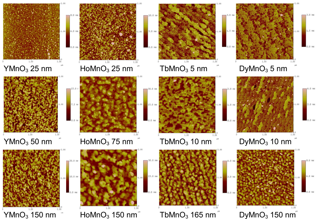
Figure 3.41 : images AFM 2x2 μm 2 de films RMnO 3 de différentes épaisseurs élaborés sur YSZ.
