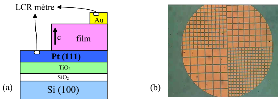
Figure 4.27 : (a) structure capacitive utilisée pour les mesures électriques - (b) image au microscope optique des électrodes d'or évaporées à travers un masque de carrés de 50x50, 70x70, 110x110 et 150x150 μm 2 .
