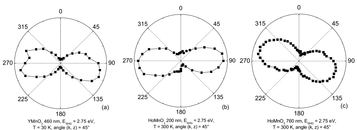
Figure 4.54 : intensité SHG en fonction de l'angle entre le polariseur et l'analyseur avec un angle de 45^\circ entre k et z, à 2.75 eV, de films élaborés à 850^\circ\text{C} sur YSZ : (a) \text{YMnO}_3 460 nm à 30 K, (b) \text{HoMnO}_3 200 nm à 300 K et (c) \text{HoMnO}_3 760 nm à 300 K.
