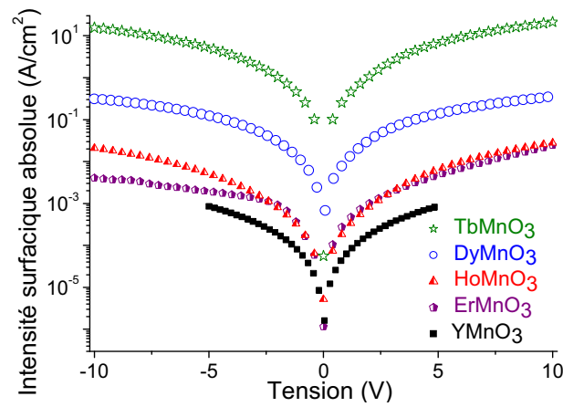
Figure 4.30 : mesures J(V) de films de RMnO_3 de 500 nm d'épaisseur (450 nm pour YMnO_3 ) déposés sur Pt/Si à 850°C.
