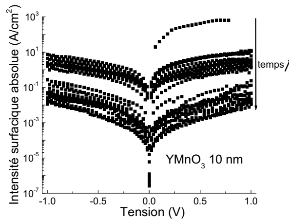
Figure 4.29 : mesures J(V) successives d'un film d'YMnO 3 de 10 nm d'épaisseur déposé sur Pt/Si à 800°C.
