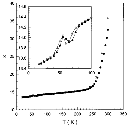
Figure 1.26 : constante diélectrique en fonction de la température sous 0 T (carrés blancs) et 5 T (cercles noirs) d'une pastille dense d'YMnO 3 [Hua97].
