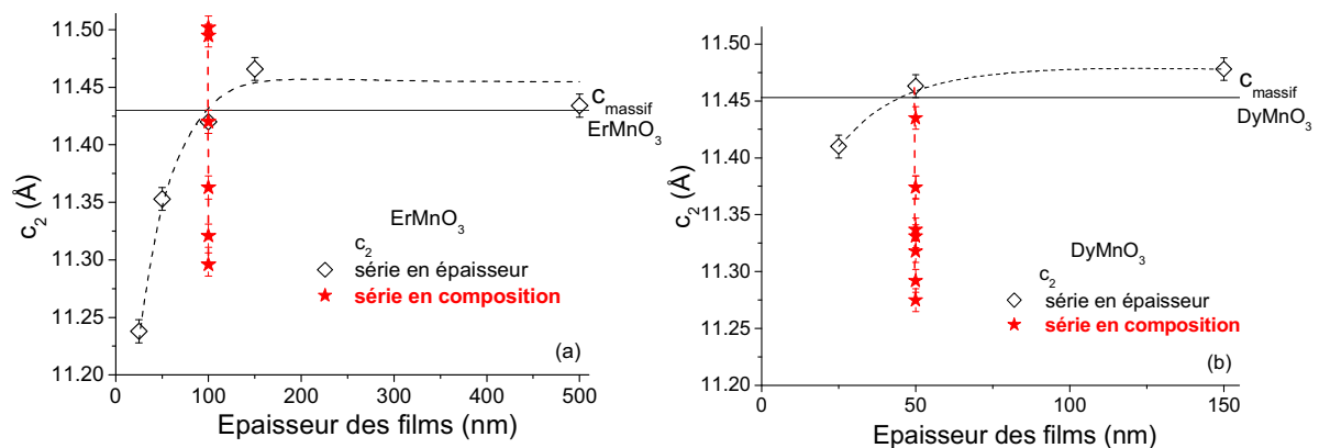
Figure 3.54 : paramètres de maille c_2 en fonction de l'épaisseur (a) de films d'ErMnO 3 et (b) de films de DyMnO 3 élaborés sur YSZ à 850°C. Les points correspondant aux différentes compositions pour les films de 100 nm (ErMnO 3 ) ou 50 nm (DyMnO 3 ) sont indiqués.
