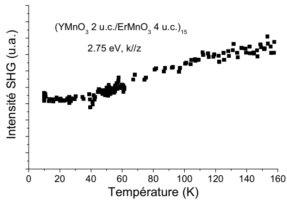
Figure 5.30 : intensité SHG en fonction de la température à 2.75 eV d'une multicouche (\text{YMnO}_3 \text{ 2 u.c./ErMnO}_3 \text{ 4 u.c.})_{15} élaborée à 850°C sur YSZ, avec k parallèle à z .
