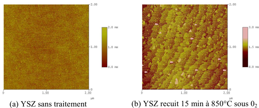
Figure 3.43 : images AFM 2x2 μm 2 d'un substrat d'YSZ (a) sans traitement et (b) après chauffage à 850°C et recuit sous une atmosphère d'O 2 pendant 15 minutes.
