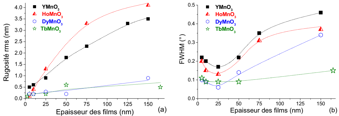
Figure 3.42 : (a) rugosité rms mesurée par AFM et (b) largeur à mi-hauteur des rocking curves mesurées sur les raies 004, de films RMnO 3 de différentes épaisseurs déposés sur YSZ.
