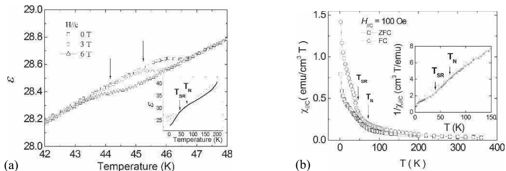
Figure 4.40 : (a) constante diélectrique sous différents champs magnétiques et (b) susceptibilité magnétique, en fonction de la température, d'un film de TbMnO 3 de structure hexagonale [Lee07c].
