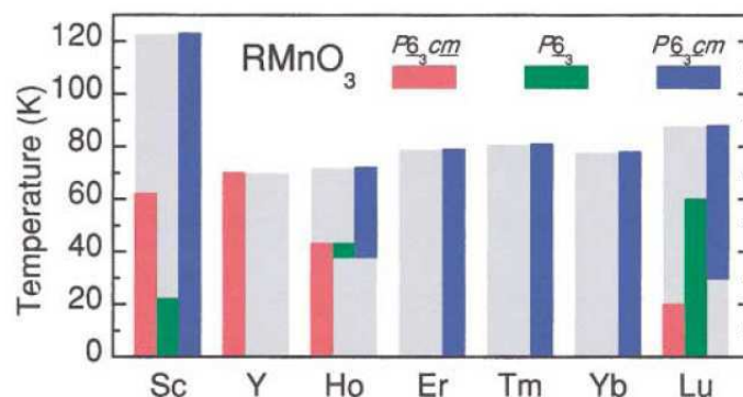
Figure 4.6 : symétries magnétiques des différents manganites de terres rares hexagonaux en fonction de la température [Fie00a].
