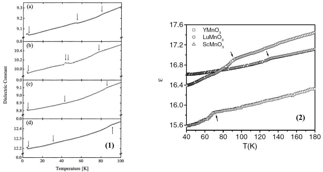
Figure 1.24 : anomalies de la constante diélectrique observées (1) sur des monocristaux de (a) HoMnO 3 , (b) ErMnO 3 , (c) TmMnO 3 et (d) YbMnO 3 [Iwa98], et (2) sur des monocristaux d'YMnO 3 , LuMnO 3 et ScMnO 3 [Tom01], aux températures de transitions magnétiques.
