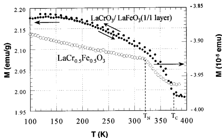
Figure 1.36 : comparaison de l'aimantation en fonction de la température d'une hétérostructure ( \text{LaCrO}_3 1 u.c./ \text{LaFeO}_3 1 u.c.) et d'un film de \text{LaCr}_{0.5}\text{Fe}_{0.5}\text{O}_3 . Du ferromagnétisme est induit dans l'hétérostructure [Ued98].
