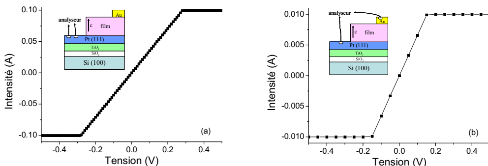
Figure 4.36 : (a) mesure I(V) effectuée en prenant les deux contacts sur le platine. (b) Mesure I(V) représentative du résultat souvent obtenu en mesurant la capacité d'un film élaboré sur Pt/Si.
