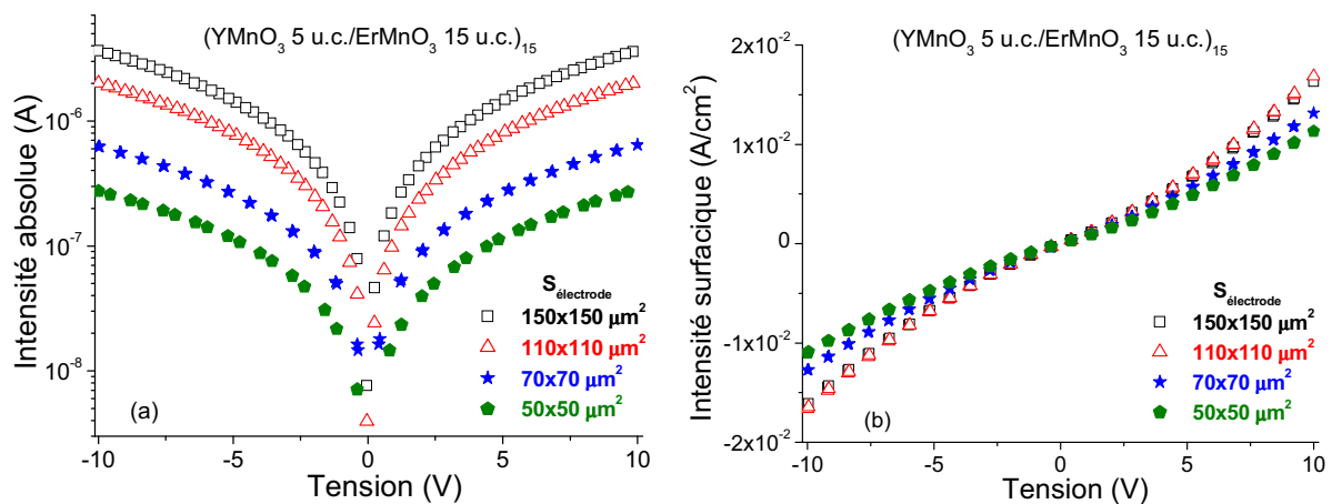
Figure 5.15 : mesures I(V) sur des électrodes de différentes surfaces d'une multicouche ( \text{YMnO}_3 5 u.c./ \text{ErMnO}_3 15 u.c.) 15 élaborée sur Pt/Si à 850°C : (a) intensité absolue, en échelle logarithmique et (b) intensité rapportée à la surface des électrodes, en échelle linéaire.
