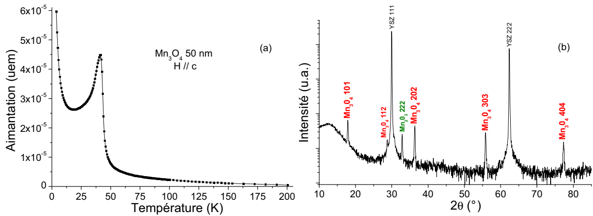
Figure 5.13 : (a) aimantation en fonction de la température d'un film de Mn 3 O 4 déposé sur YSZ à 850°C – aimantation mesurée sous 0.2 T, en ZFC, avec H//c. (b) Diagramme de diffraction \theta/2\theta du film (intensité en échelle logarithmique).
