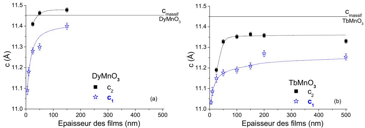
Figure 3.36 : paramètres de mailles c_1 et c_2 en fonction de l'épaisseur des films stabilisés de (a) \text{DyMnO}_3 et (b) \text{TbMnO}_3 déposés sur YSZ (calculés d'après la position des pics de la raie 008 du manganite).
