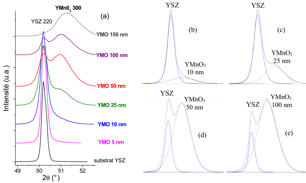
Figure 3.39 : (a) diagrammes de diffraction \theta/2\theta mesurés en incidence rasante sur les raies 220 du substrat YSZ et 300 de films d'YMnO 3 de différentes épaisseurs élaborés à 850°C. Exemples de déconvolution des pics pour les films de (b) 10, (c) 25, (d) 50 et (e) 100 nm d'épaisseur.
