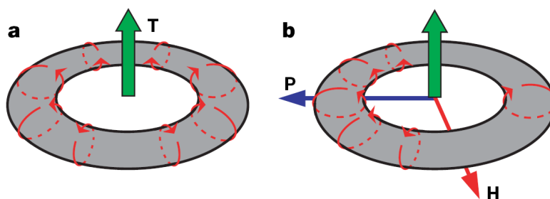
Figure 1.5 : (a) repr sentation d'un moment toroïdique. (b) Induction d'une polarisation  lectrique P par un champ magn tique H dans un compos  ferrotoroïdique [Van07].
