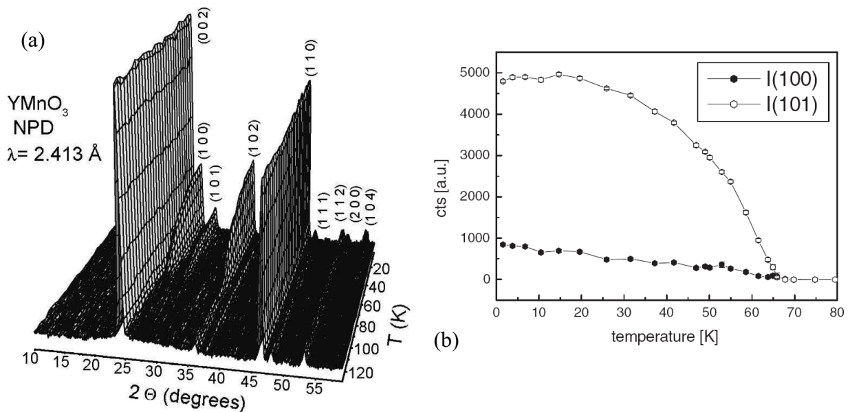
Figure 4.8 : (a) diagramme de diffraction neutronique en fonction de la température d'une poudre d' \text{YMnO}_3 [Muno00]. (b) Intensité des raies 010 et 011 d'une poudre d' \text{YMnO}_{3-\delta} , avec \delta = 0.29 , mesurée en fonction de la température par diffraction des neutrons [Lon02].
