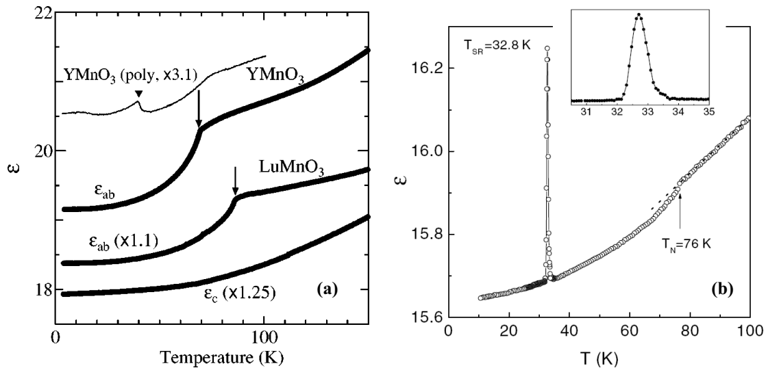
Figure 1.25 : anomalies de la constante diélectrique observées (a) sur des monocristaux d'YMnO 3 et LuMnO 3 à T_N [Kat01] et (b) sur un monocristal d'HoMnO 3 à T_{SR} et T_N [Lor04a].
