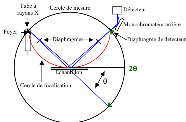
Figure 2.7 : schéma de principe du montage Bragg-Brentano.
