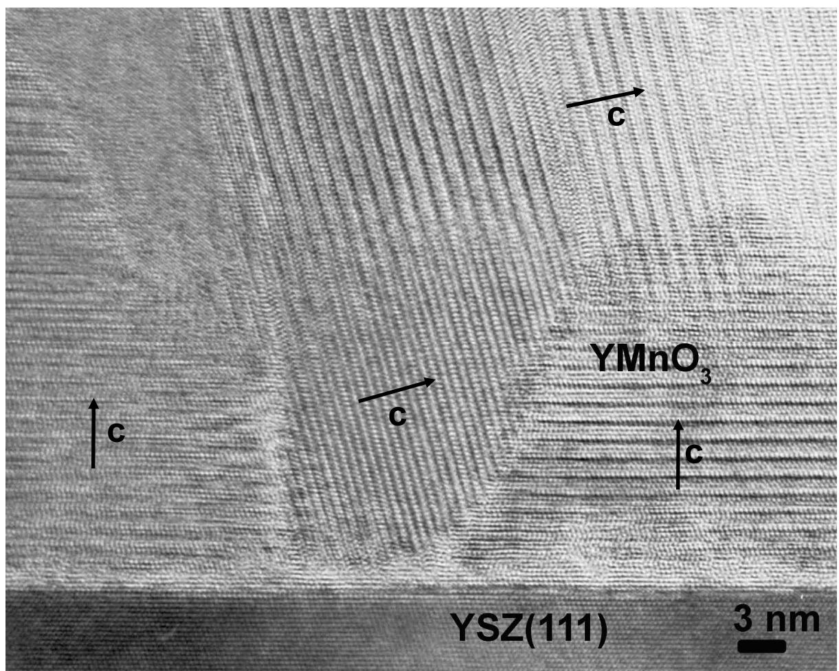
Figure 3.15 : image HRTEM de la cross-section d'un film d' \text{YMnO}_3 de 100 nm d'épaisseur déposé sur YSZ à 800°C. Des orientations secondaires 111 sont observées.
