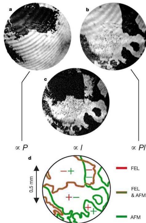
Figure 1.27 : domaines (a) ferroélectriques FEL, (c) antiferromagnétiques AFM et (b) FEL et AFM, d'une pastille dense d'YMnO 3 , imagés par génération de second harmonique à 6 K. (d) Schéma de ces domaines avec le signe de l'orientation des paramètres d'ordres [Fie02a].
