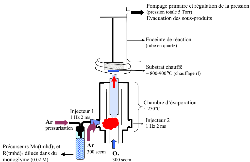
Figure 2.4 : schéma du réacteur MOCVD à injection utilisé. Adaptée d'après [The06].
