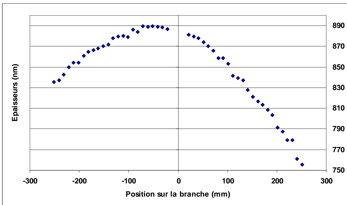
Figure 3-40 : Mesures d'épaisseurs sur la branche en orientation +45^\circ . La position sur la branche correspond à l'abscisse curviligne.
