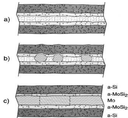
Figure 3-5 : Schéma de la transition amorphe-cristallin des couches de Mo. (a) La couche est amorphe tant que l'épaisseur est inférieure à \tau_c . (b) La rugosité de surface de la couche permet d'atteindre ponctuellement \tau_c , ce qui entraîne la cristallisation en ces points. (c) Au-dessus de l'épaisseur critique la couche est presque entièrement polycristalline. [73]
