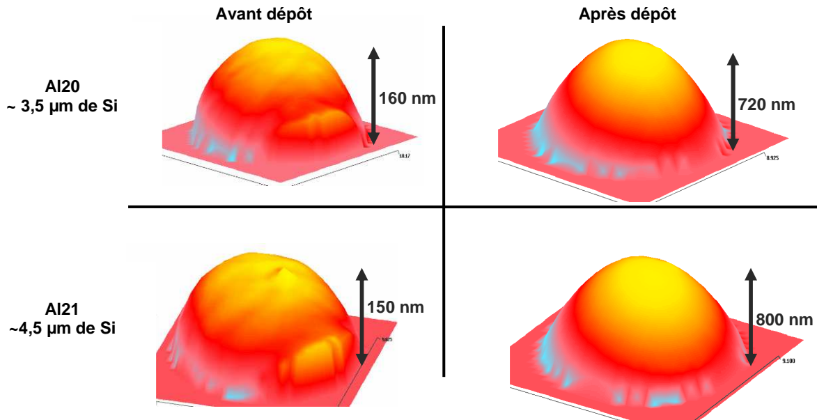
Figure 2-31 : Surface et flèche des échantillons AL20 et AL21 avant et après dépôt d'une couche de silicium. L'épaisseur de la couche pour AL20 est de 3,5\mu\text{m} et celle pour AL21 est de 4,5\mu\text{m} .
