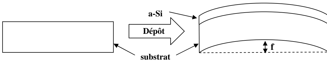
Figure 2-29 : Principe de la mesure de contraintes mécaniques dans les couches.
