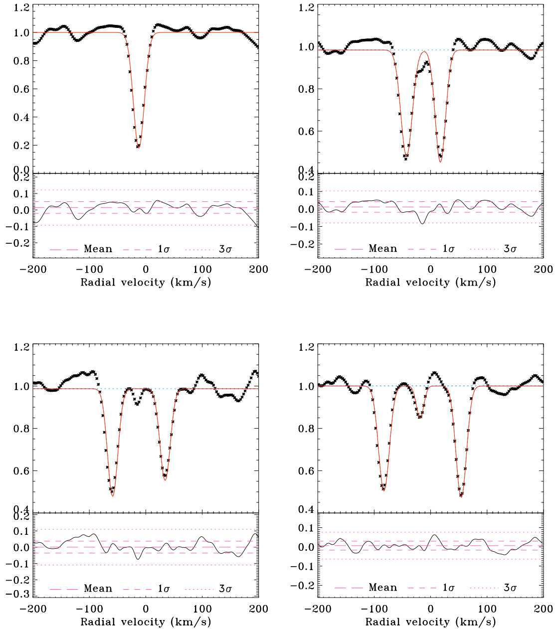
FIG. IV.2 – Les CCFs de RasTyc 0524+6739 à différentes phases orbitales. Elles permettent de souligner le changement de la configuration orbitale d’une forme avec un pic à la conjonction ( en haut à gauche ) à trois pics proche de la quadrature ( en bas à droite ), en passant par une phase intermédiaire où seulement deux pics sont visibles ( en haut à droite et en bas à gauche ). L’incertitude de RV est d’environ 1 \text{ km s}^{-1} à notre résolution spectrale. Dans chaque figure, les ajustements des CCFs par de multiples gaussiennes sont affichés avec des lignes rouges ( boîtes du haut ) ainsi que les résidus des ajustements ( boîtes du bas ).
