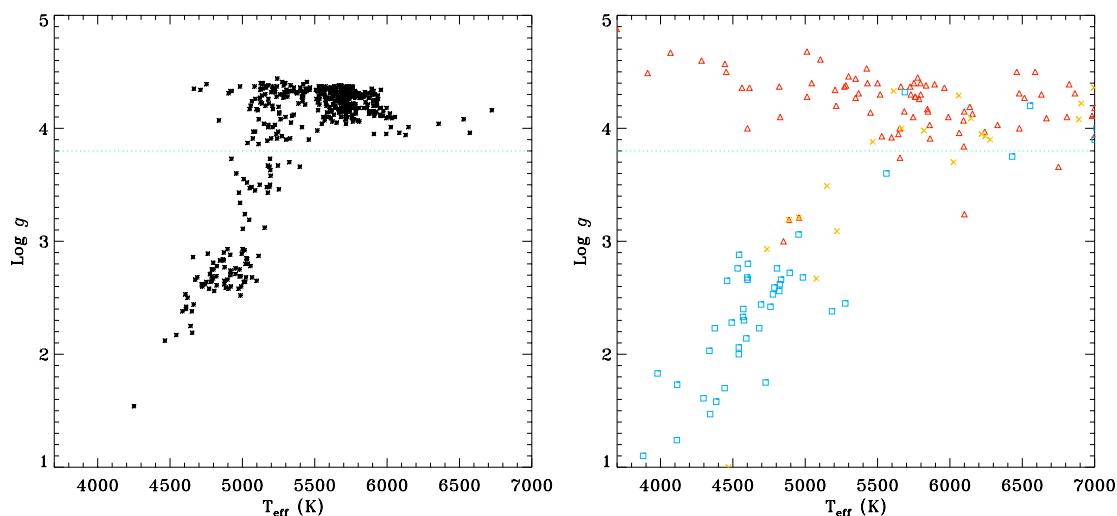
FIG. II.15 – Diagramme \log g vs. T_{eff} des étoiles analysées avec ROTFIT ( panneau de gauche ) comparable au diagramme des étoiles de TGMET ( panneau de droite ).
