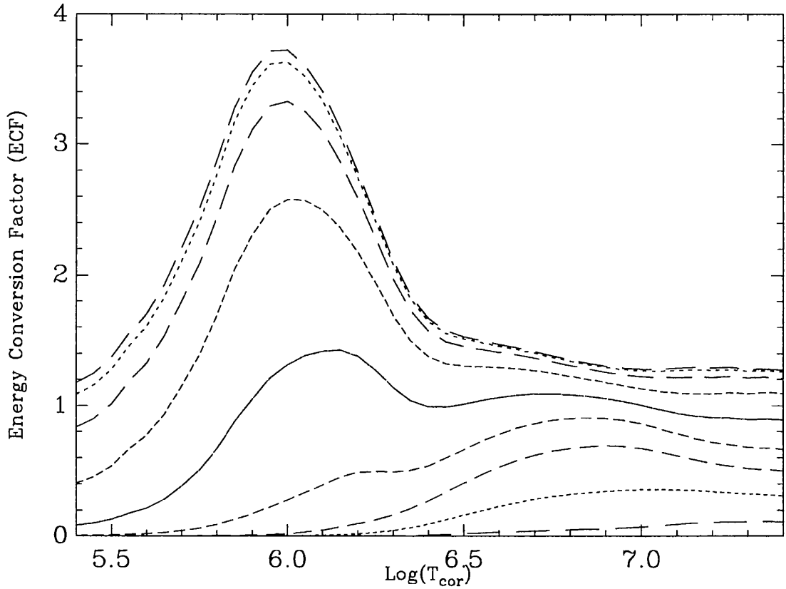
FIG. V.2 – Valeurs du Facteur de Conversion en Énergie (ECF) pour le PSPC de ROSAT dans le cas d'un plasma thermique de type Raymond Smith et d'une loi d'absorption galactique standard. Cette ECF est calculé en fonction de la température du plasma ( T_{cor} ) et pour des valeurs de la colonne densité N_H allant de 10^{18.0} (enveloppe supérieure) à 10^{22.0} (enveloppe inférieure) avec un pas de 0.5 sur une échelle logarithmique. Cette figure est extraite de Guillout et al. (1996).
