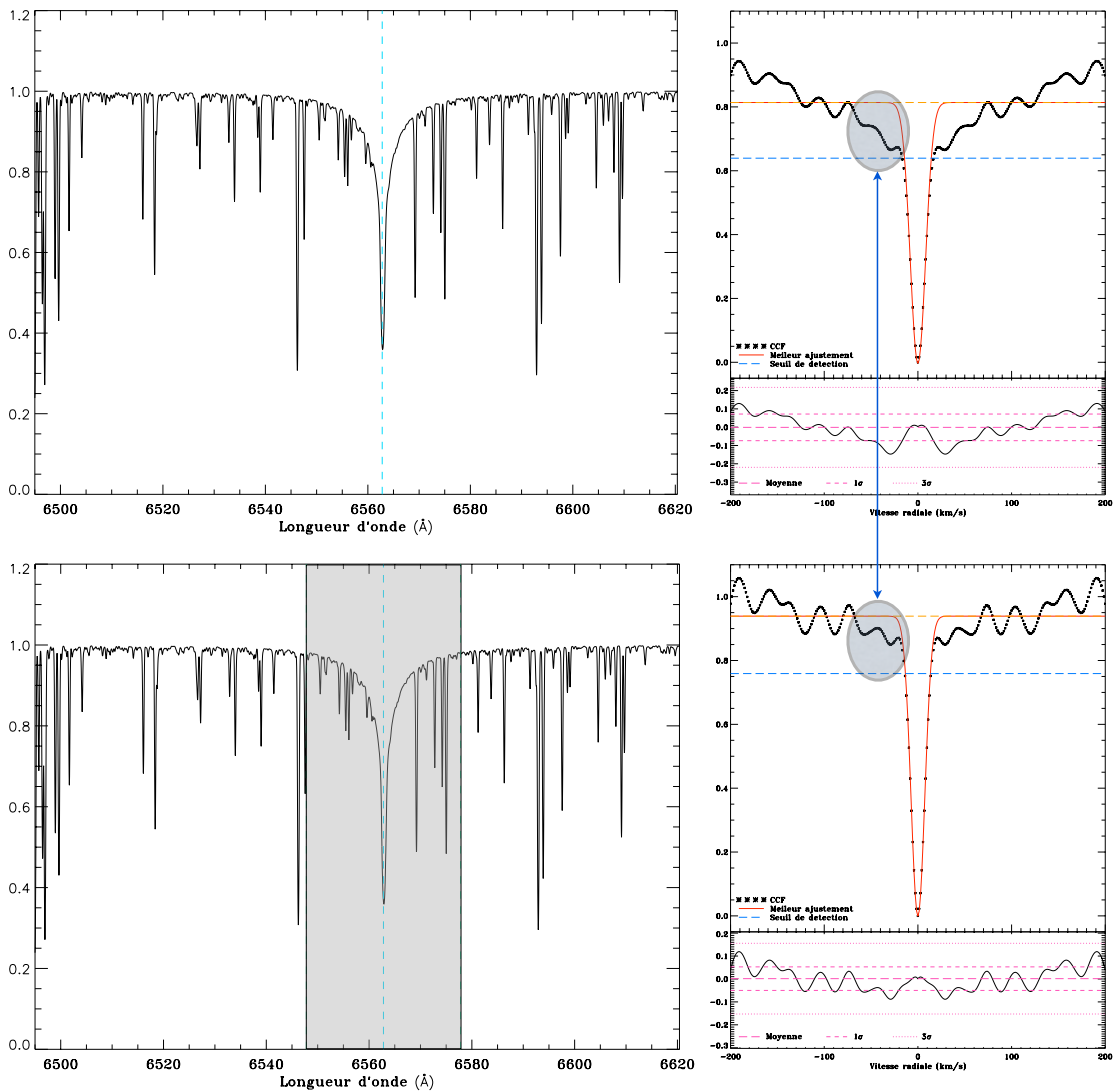
FIG. II.3 – Application d’un masque pour la raie H\alpha . Pour illustrer le rôle de ce masque, j’ai généré le spectre synthétique d’une étoile G5 V ( T_{eff} = 5500 K, \log g = 4.0 , [Fe/H] = 0.00 et v \sin i = 0.0 km s ^{-1} ). Les spectres ( panneaux de gauche ) et leurs CCFs associées ( panneaux de droite ) sont indiqués pour le cas sans masque ( panneaux supérieurs ) et avec masque ( panneaux inférieurs ). La CCF obtenue résulte de la corrélation de chaque spectre avec lui-même. Ces deux CCFs montrent que l’influence des ailes est nettement réduite lors de l’application du masque. En effet, la base de la gaussienne ligne orange pointillée passe de \sim 8.1 (sans masque) à \sim 9.4 (avec masque) ce qui est notamment dû à la diminution des “ailes” autour du pic significatif (zones encerclée).
