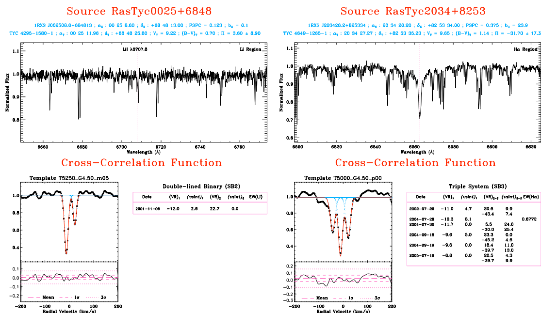
FIG. II.12 – Fiches d'identification ( panneaux de gauche à droite ) du système binaire RasTyc 0025+6848 (BD+67 34) et du système triple RasTyc 2034+8253 (BD+82 622).
