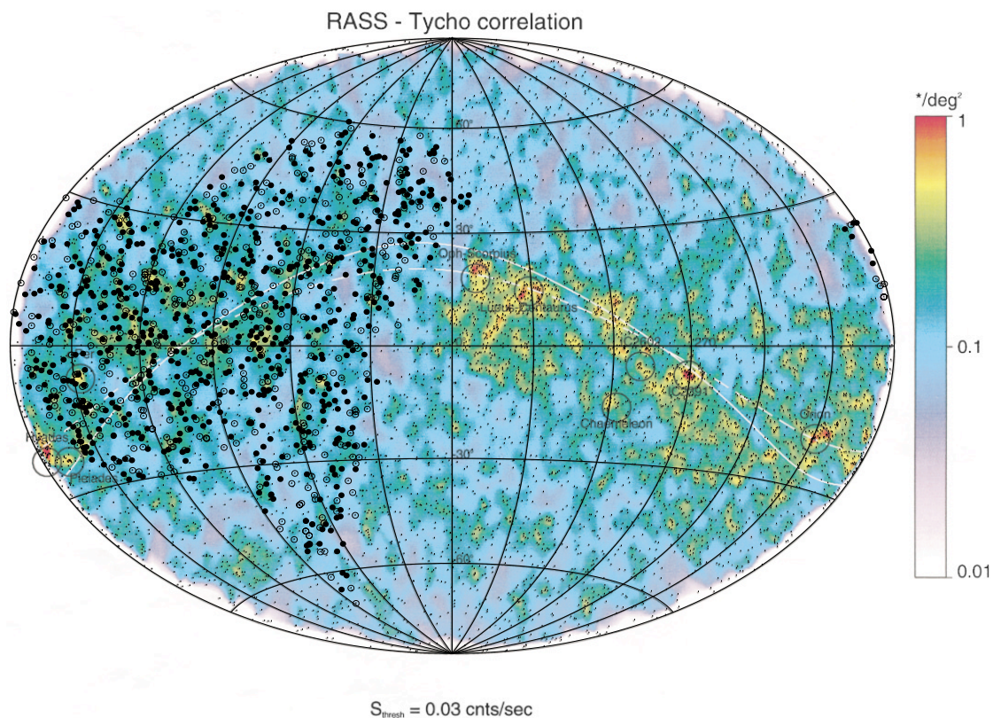
FIG. I.6 – Distribution galactique (projection "Aitoff") des étoiles sélectionnées pour le programme d'observations ( grands cercles ) indiquée par-dessus celles des 8 593 sources RasTyc ( petits points ). Toutes les sources de l'échantillon BRILLANT ( cercles pleins ) ont déjà été observées et analysées, tandis que celles de l'échantillon FAIBLE ( cercles vides ) sont en cours d'observations sur le TNG T358 (télescope italien) à La Palma.
