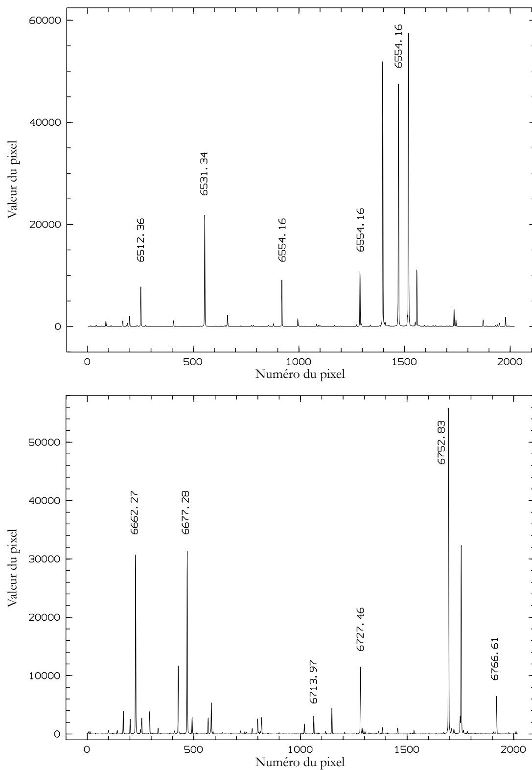
FIG. I.12 – Identification des raies utilisées lors de la calibration des spectres dans les régions spectrales centrées autour de la raie H\alpha ( en haut ) et de celle du lithium ( en bas ). Toutes les longueurs d'onde indiquées sur la figure s'expriment en Å.
