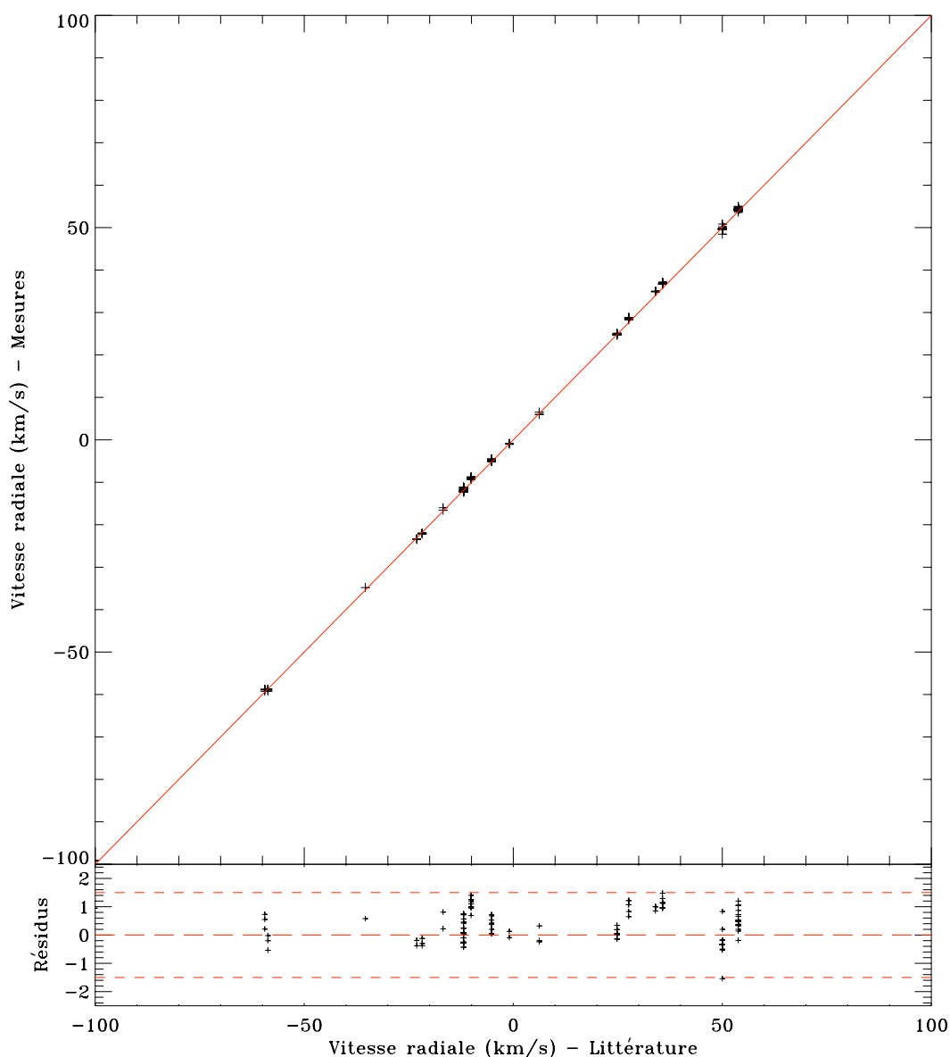
FIG. II.6 – Comparaison de nos mesures de vitesses radiales ( symboles “+” des étoiles standards avec celles trouvées dans la littérature. Ces étoiles ont été observées au cours du même programme d’observations. La relation unitaire ligne rouge en continu est indiquée sur le panneau du haut. La différence entre nos mesures et cette relation est montrée sur le panneau inférieur avec la ligne composée de longs tirets. Celles composées de petits tirets délimitent la région de 1.5 \text{ km s}^{-1} autour de la relation unitaire.
