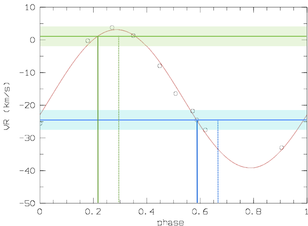
FIG. I.9 – Schéma présentant notre stratégie pour l'identification des systèmes de type SB1 : DFCam est prise comme exemple. Les mesures de vitesses radiales et la solution orbitale sont indiquées par des cercles noirs et une ligne continue rouge, respectivement. Nous avons illustré notre stratégie d'observations pour une observation proche de conjonction ( en bleu ) et pour une seconde proche de la quadrature de phase ( en vert ). Pour ces deux observations, nous avons également indiqué le milieu de la première observation ( trait vertical en continu ), celui (au plus tôt) de la seconde ( trait vertical en pointillé ) et la boîte d'incertitude (deux fois celle théorique) due à la résolution de nos données centrée sur la vitesse radiale dérivée lors de la première observation ( trait horizontal en continu ).
