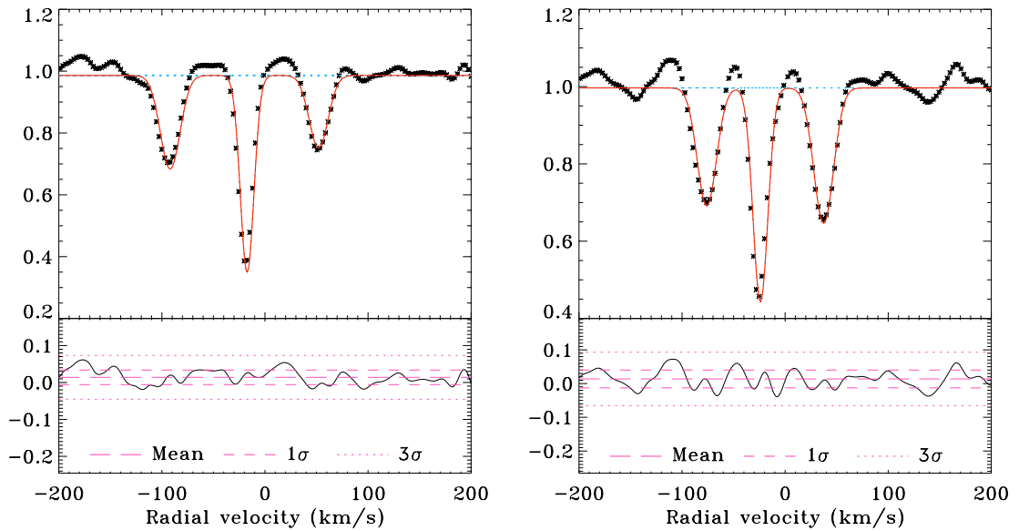
FIG. IV.3 – Les CCFs de RasTyc 1828+3506 montrent clairement trois pics avec des poids différents. Les composantes de la binaire interne semblent avoir une rotation plus rapide que celle de la troisième étoile, probablement due à une synchronisation des périodes de rotation axiale et de révolution orbitale.
