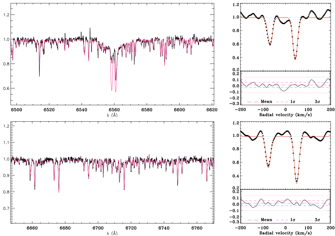
FIG. II.9 – Spectres Aurélie observé ( panneaux de droite, ligne continue en noir ) du système SB2, BD+02 4456 (RasTyc 2159+0302), dans les régions spectrales de H \alpha ( panneaux du haut ) et du lithium ( panneaux du bas ) sur lequel on a superposé le spectre synthétique ( ligne continue en rouge ) construit comme la somme pondérée de deux spectres de référence Elodie élargis à la vitesse de rotation des composante du système et décalés suivant les vitesses radiales. Ces deux paramètres sont déterminés à partir de l'ajustement de la CCF ( panneaux de droite ).
