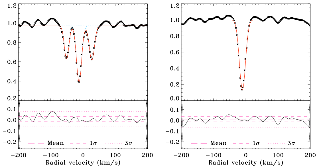
FIG. IV.4 – Les CCFs de RasTyc 2034+8253 a deux phases orbitales. La nature du système triple apparaît dans la CCF ( à gauche ) alors qu'elle est complètement cachée dans une autre phase ( à droite ).
