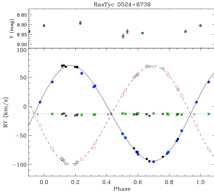
FIG. IV.5 – Courbes de vitesse radiale de RasTyc 0524+6739 (boîte inférieure). Les grands symboles font référence aux données du spectrographe AURELIE tandis que les plus petits sont utilisés pour ceux du spectrographe FRESCO. Des cercles pleins et ouverts réfèrent aux composantes primaire et secondaire de la binaire interne, respectivement. Dans chaque panneau, les lignes en continu et en tirets représentent les solutions orbitales pour la composante primaire et secondaire, respectivement, alors que la ligne en pointillé symbolise le barycentre de la binaire interne. Les astérisques et les “plus” sont utilisées pour la troisième composante et pour les valeurs de RV “mélangées”, respectivement. Toutes les erreurs de RV sont inférieures ou comparables à la taille des symboles. La photométrie est également affichée en fonction de la phase orbitale (boîte supérieure).
