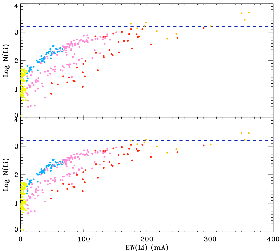
FIG. II.17 – Diagramme de l’abondance du lithium ( \log N(\text{Li}) ) en fonction de la largeur équivalente du lithium ( EW(\text{Li}) ) connaissant les paramètres astrophysiques ( T_{eff} et \log g ) de nos sources. Les couleurs correspondent aux différents groupes d’âge identifiés et sont similaires à celles utilisées en Fig II.16. Nous avons utilisé les calculs de Pavlenko & Magazzu (1996) dans le cas ETL ( panneau supérieur ) et dans le cas NETL ( panneau inférieur ). Les droites horizontales ( \log N(\text{Li}) = 3.2 ) correspondent à l’abondance du lithium primordiale.
