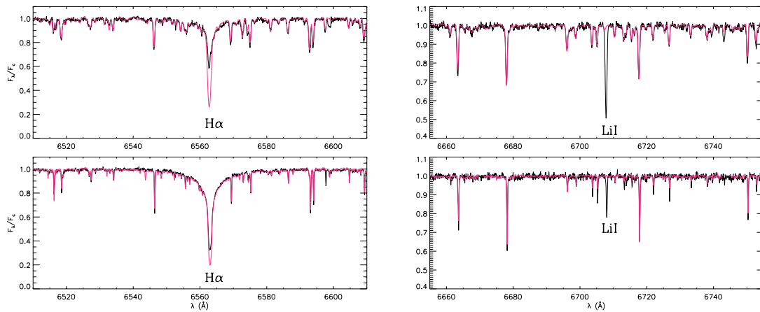
FIG. II.8 – Ajustement avec COMPO1 de spectres ( lignes noires ) dans les régions H \alpha ( panneaux de gauche ) et dans celle du lithium ( panneaux de droite ) pour l'étoile BD+45 598 (RasTyc 0221+4600) riche en lithium ( panneaux du haut ) et pour l'étoile BD+38 194 (RasTyc 0107+3915) assez jeune ( panneaux du bas ). Le spectre de l'étoile de référence (considérée comme n'ayant aucune activité) est également indiqué avec une ligne rouge.
