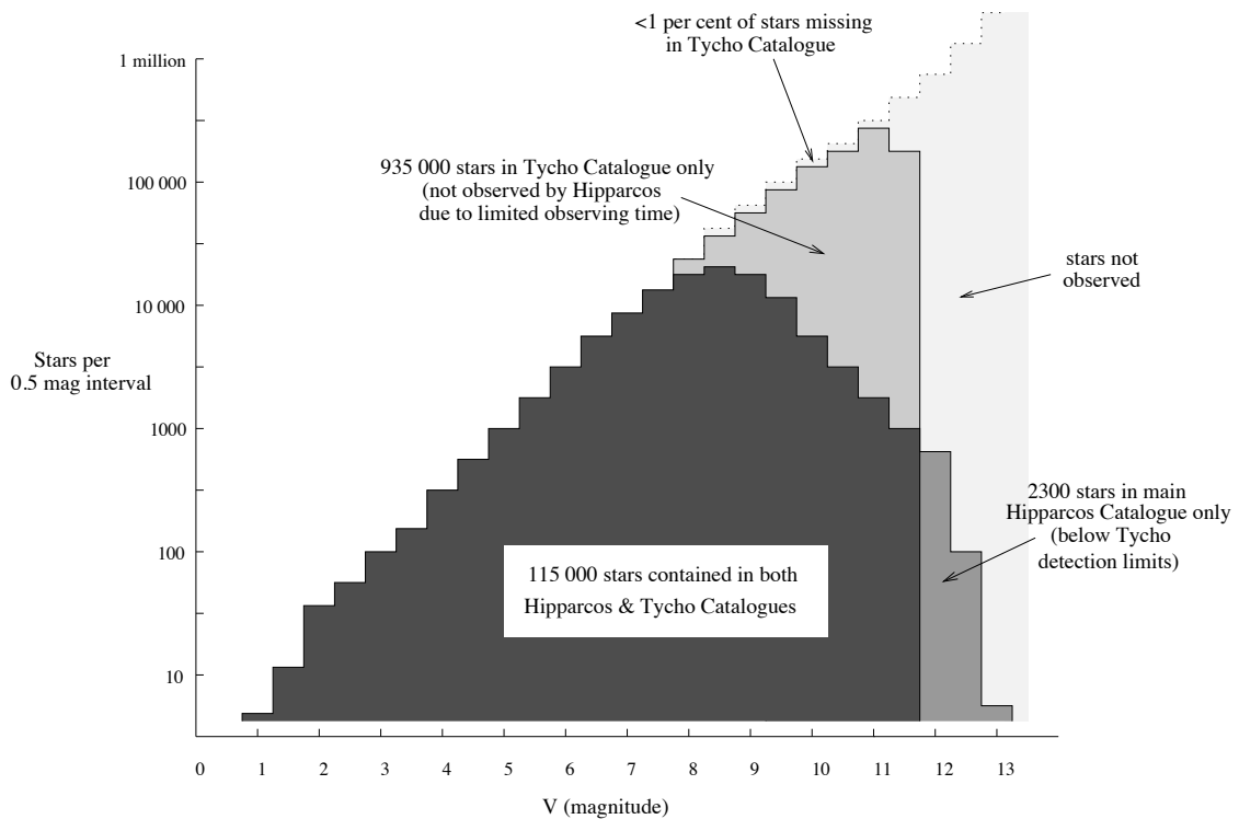
FIG. I.2 – Complétude et superposition des 118 218 entrées du catalogue HIPPARCOS et de l'ensemble du catalogue TYCHO. Le premier est largement complet pour V = 7.3 - 9 mag, en fonction de la latitude galactique et du type spectral. Les étoiles ayant une magnitude V > 9 mag, distribuées avec une densité relativement constante au-dessus de la sphère céleste, sont toutes sous la limite de détection de V \approx 12.5 mag. Le catalogue TYCHO est largement complet jusqu'à environ V = 10.5 mag et contient également des objets jusqu'à la limite de cette instrument ( V \approx 11 - 11.5 mag). Par conséquent, la plupart des entrées HIPPARCOS sont également contenues dans le catalogue TYCHO, sauf pour près de 2300 sources dont la magnitude est supérieure au seuil de détection de TYCHO. Cette figure est extraite de ESA (1997).
