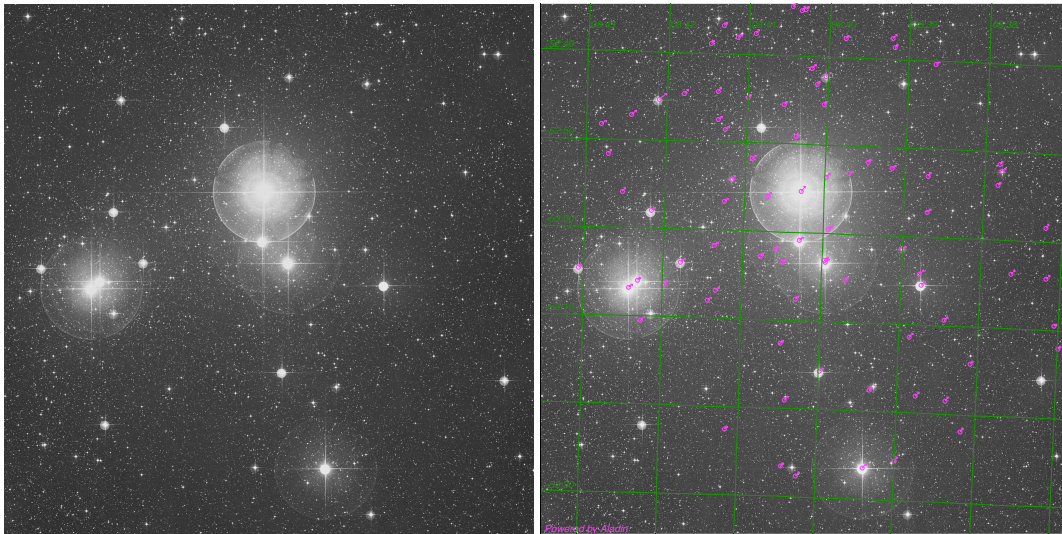
FIG. 3 – À gauche : Un champ DSS typique du ciel de 60 arcmin centré sur l’amas IC 2391 ( \alpha = 8^{\text{h}}40^{\text{m}}2 , \delta = -53^{\circ}04^{\text{m}}0 ). À droite : Même champ dont l’astrométrie a été calibrée avec ALADIN. Nous appliquons grâce à ce même outil une sélection des sources de la base de données SIMBAD partageant le même mouvement spatial (cercles violets). Au final, toutes les étoiles sélectionnées sont effectivement associées à IC 2391 dans cette même base.
