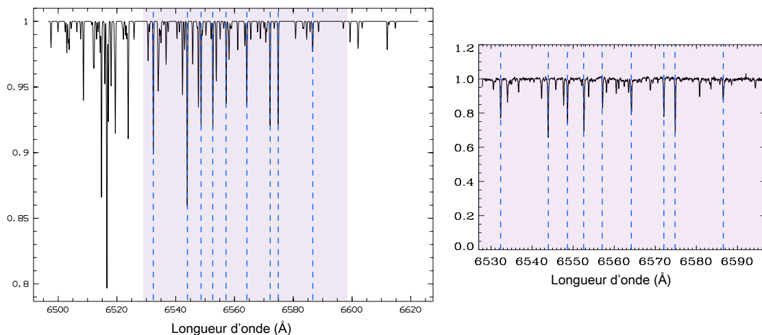
FIG. I.16 – Spectre “synthétique” des raies telluriques utilisé comme modèle dans la région H\alpha (à gauche) à comparer au modèle (à droite) publié par Frasca et al. (2000) obtenu par la division du spectre observé par celui ajusté. J’ai indiqué le positionnement des raies telluriques les plus importantes (ligne bleue en tirets) dans la région commune aux deux spectres (en violet).
