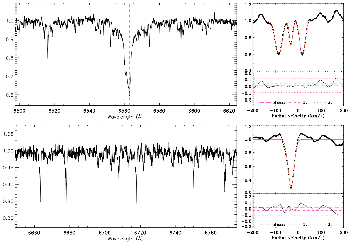
FIG. A.4 – Comme la Fig A.1 mais pour le système triple RasTyc 1522+5516.
