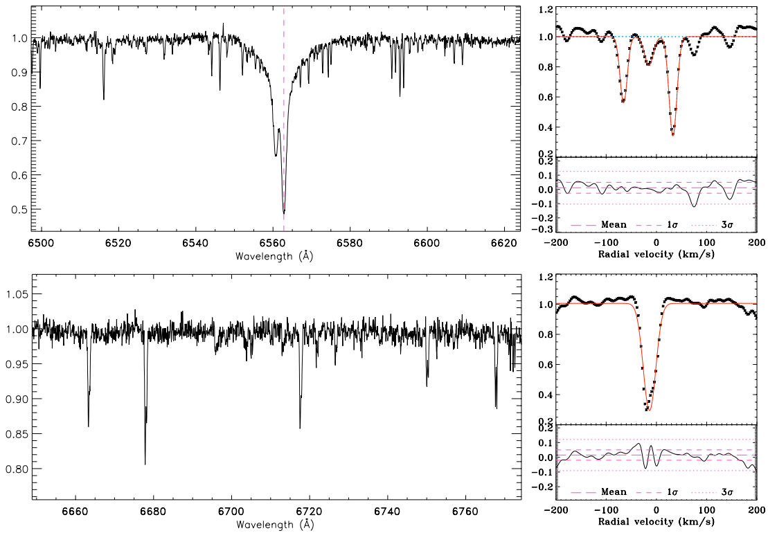
FIG. A.1 – Spectres ( panneaux de gauche ) et fonctions de corrélation ( panneaux de droite ) du système triple RasTyc 0318+3203 obtenus dans la région spectrale centrée sur H \alpha ( panneaux supérieurs ) et sur celle du lithium ( panneaux inférieurs ).
