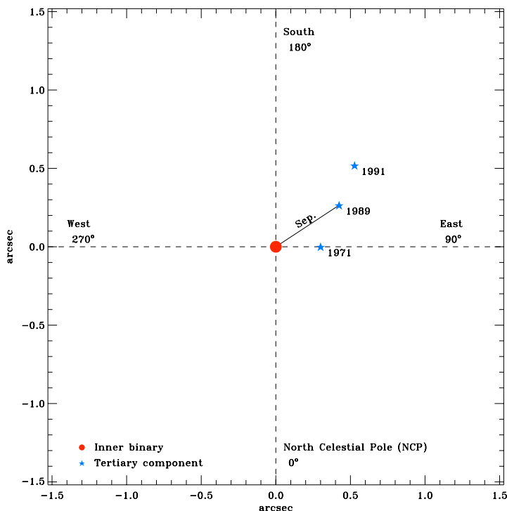
FIG. IV.14 – Évolution temporelle de la troisième composante de RasTyc 2034+8253. Les mesures de PA et de la séparation listées dans la Table IV.9 sont affichées sur le diagramme.
