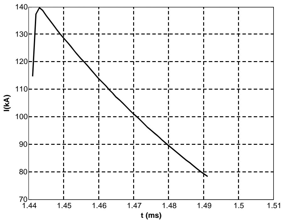
Figure 3.14.g : Courant lors de l'arc retour.
