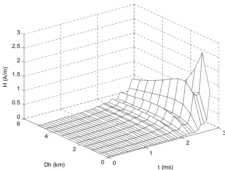
Figure 3.22: Champ magnétique rayonné par le leader négatif d'électrode en fonction de la position horizontale D_h avec l'axe de la décharge et en fonction du temps avant le début saut final. Distance nuage – sol = 7500 m ; tension 50 MV.
