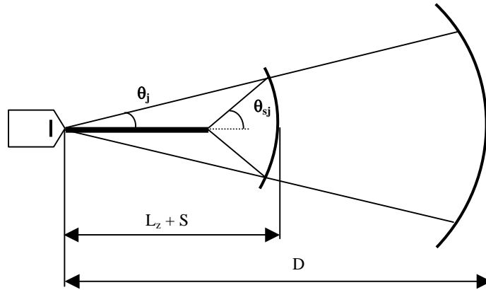
Figure 2.9 : Approximation sphérique utilisée pour le calcul des capacités [18]
