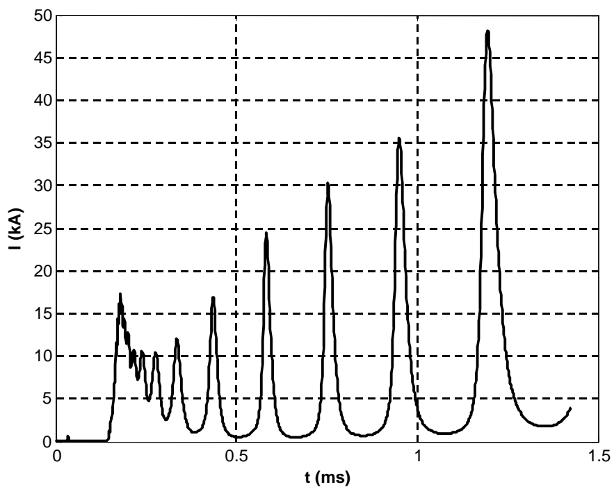
Figure 3.14.b : Courant dans le leader négatif d'électrode pendant la propagation.
