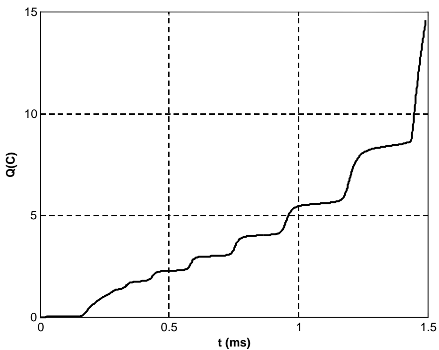
Figure 3.13.c : Charge injectée dans l'intervalle d'air.
