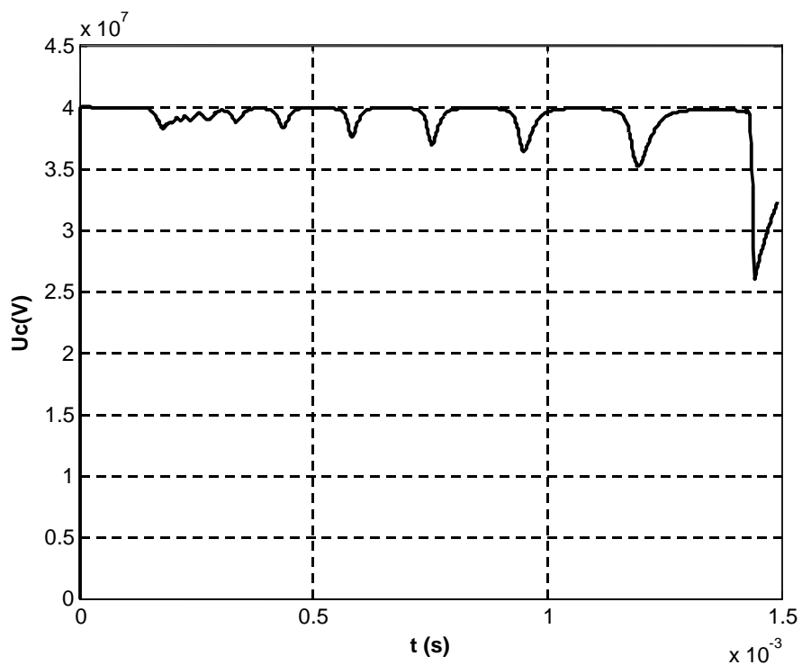
Figure 3.14.i : Tension appliquée dans l'intervalle d'air.
