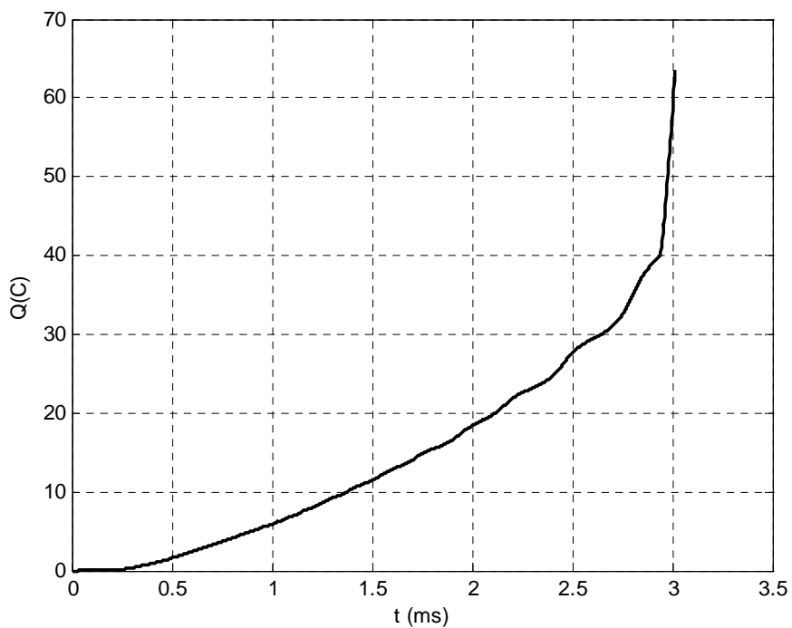
Figure 3.16.c : Charge injectée dans l'intervalle d'air.
