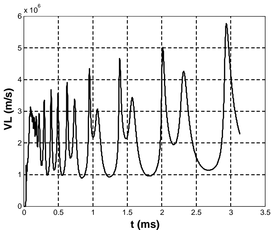
Figure 3.15.e : Vitesse instantanée du leader négatif d'électrode.
