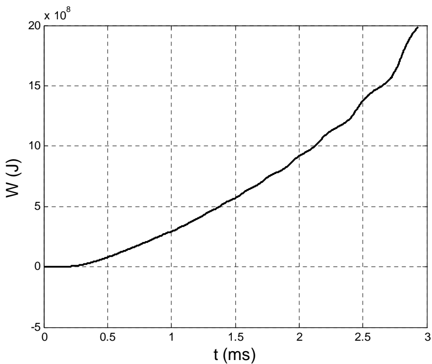
Figure 3.16.g : Energie injectée dans l'intervalle d'air.
