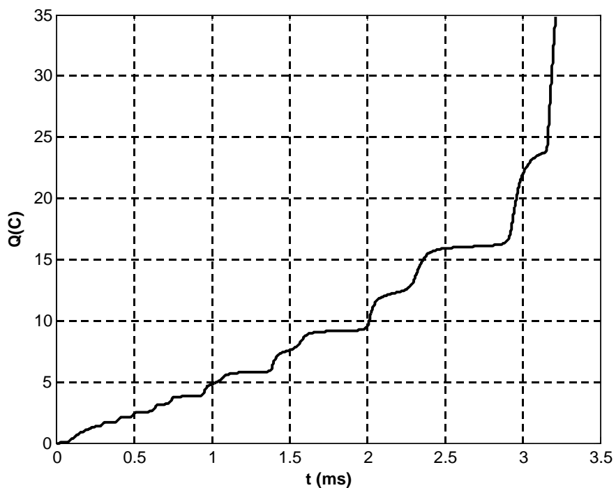
Figure 3.15.c : Charge injectée dans l'intervalle d'air.
