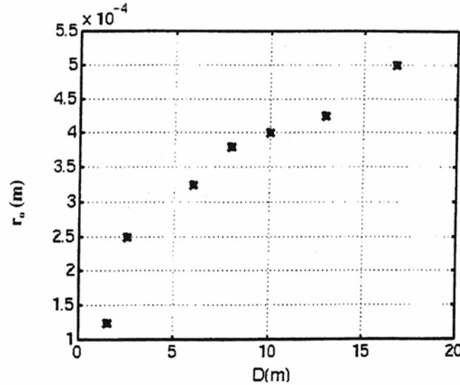
Figure 2.6 : La variation du rayon initial du leader positif en fonction de la distance interélectrode extrapolée obtenus à partir des valeurs expérimentales [9, 10].
