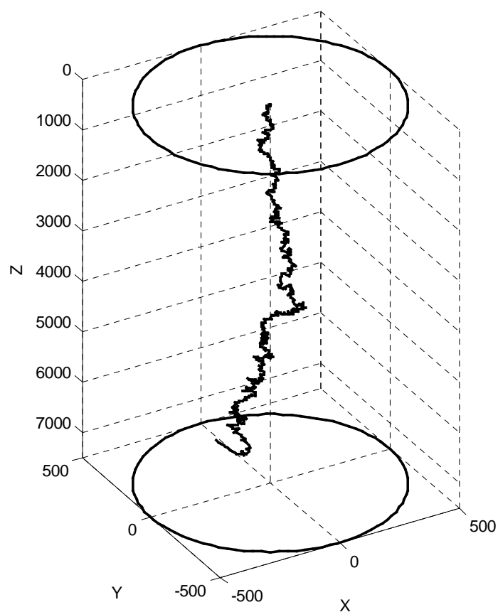
Figure 3.16.a : Trajectoire spatiale du leader négatif d'électrode.
