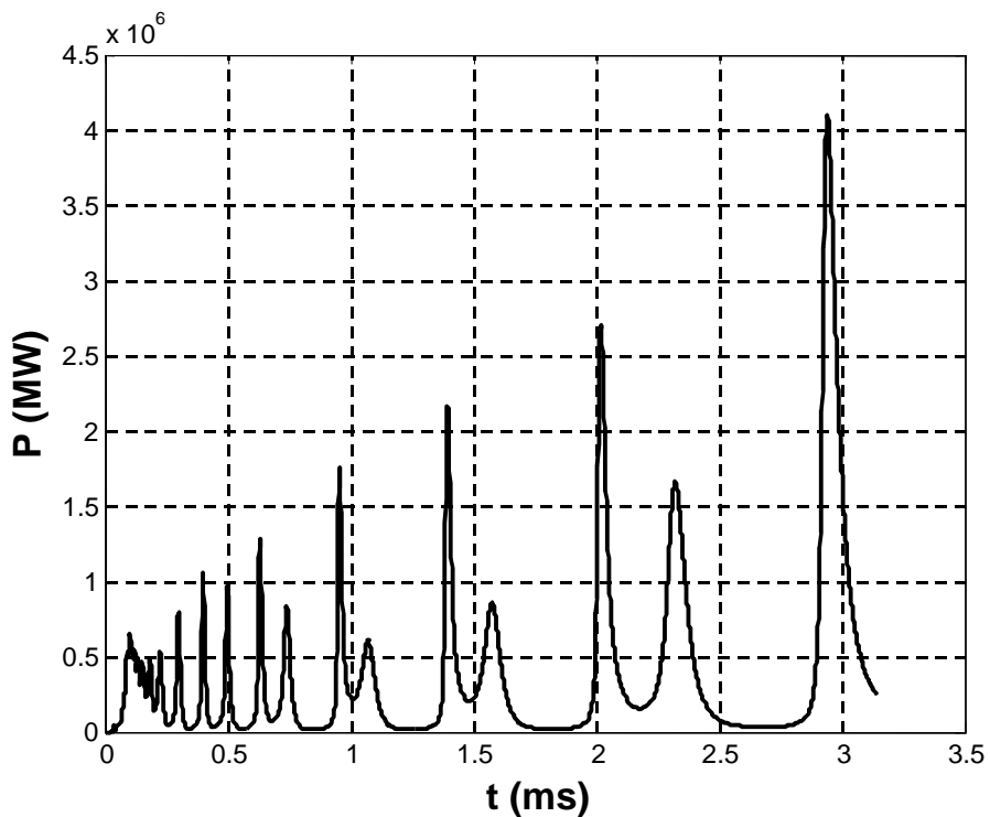
Figure 3.15.g : Puissance injectée dans l'intervalle d'air.
