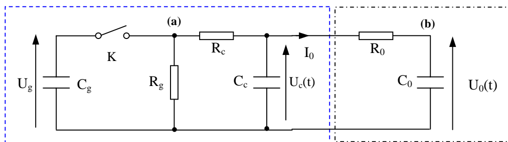
Figure 2.10 : Schéma équivalent du générateur de Marx (a) et de l'électrode équivalente (b)
