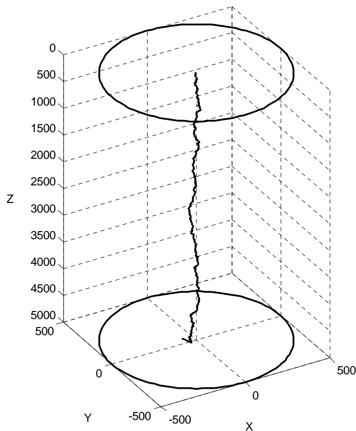
Figure 3.15.a : Trajectoire spatiale du leader négatif d'électrode.
