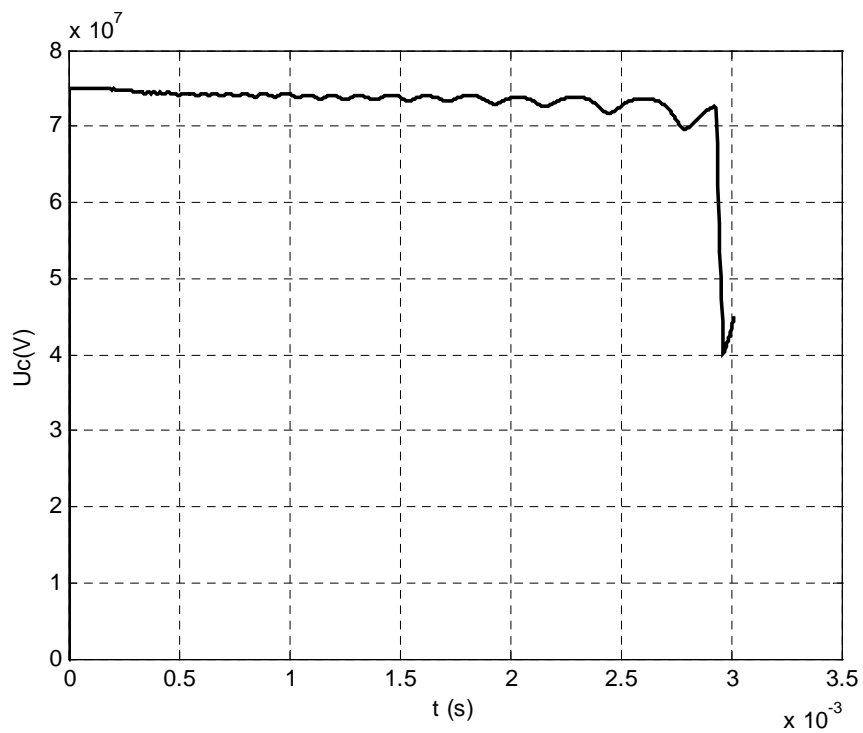
Figure 3.16.h : Tension appliquée dans l'intervalle d'air.
