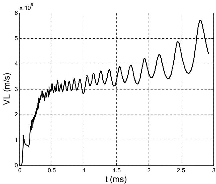
Figure 3.16.e : Vitesse instantanée du leader négatif d'électrode.
