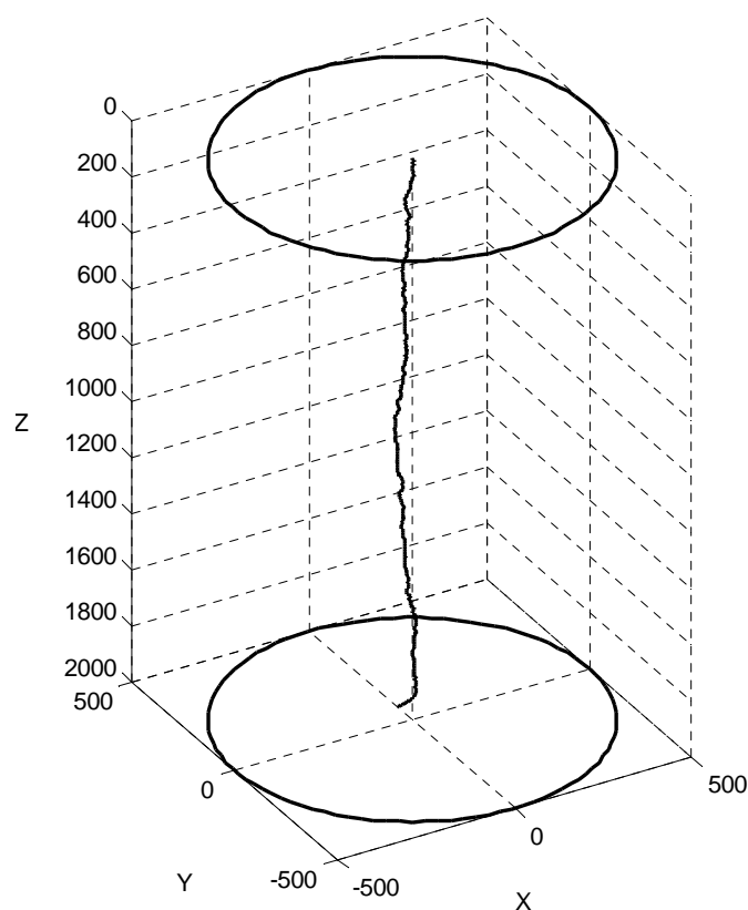
Figure 3.14.a : Trajectoire spatiale du leader négatif d'électrode.
