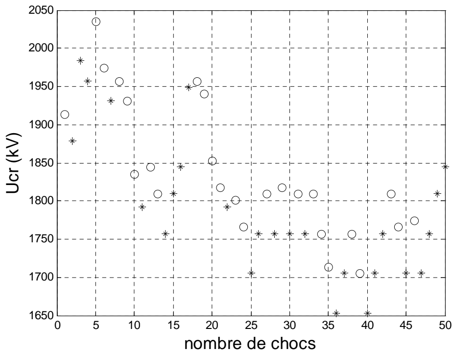
Figure 3.4: Une séquence "up and down". Intervalle D = 2,6 m. Onde 60/3000 \mu s . Les cas d'amorçage sont caractérisés par les points « o » et les cas de tenue par des astérix « * ». U_{50} = 1813,9 kV et \sigma = 2,4\% .
