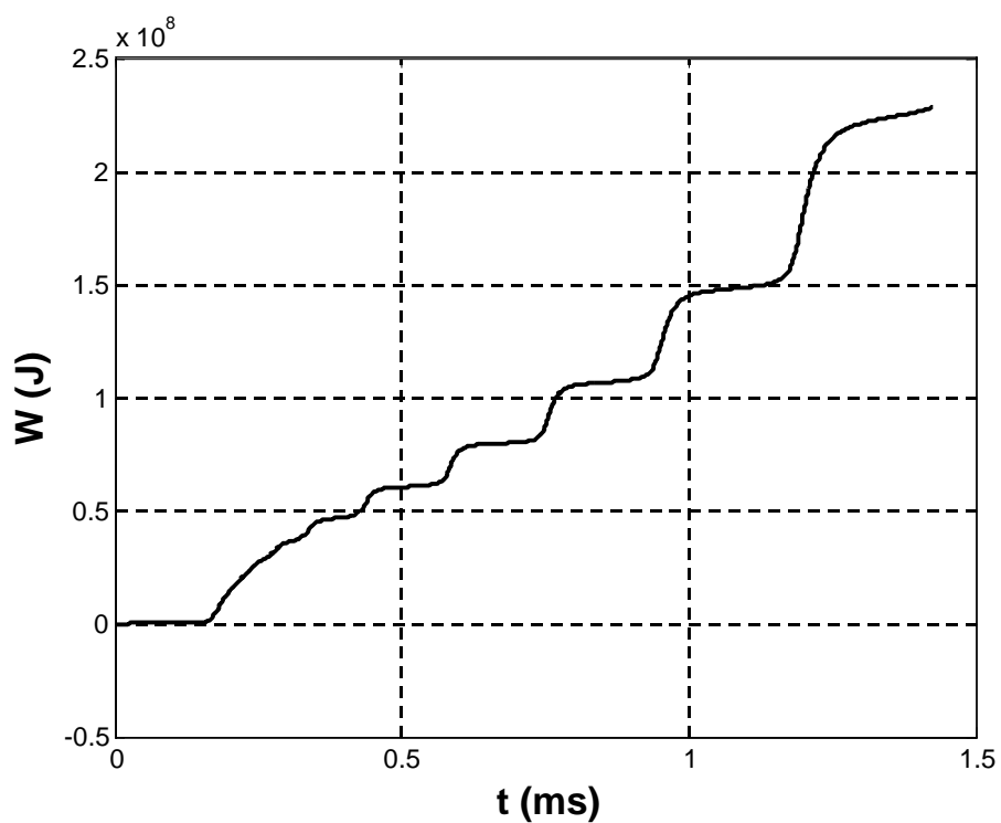
Figure 3.14.h : Energie injectée dans l'intervalle d'air.
