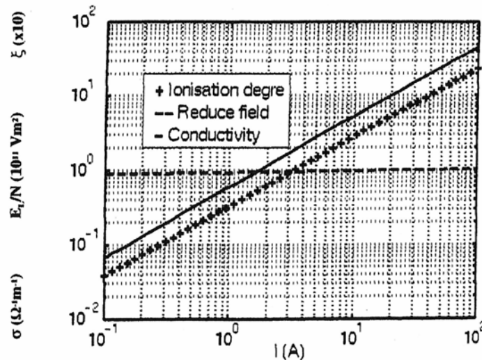
Figure 2.7 : Caractéristiques du canal de leader positif en fonction du courant pour r_0 = 1 \text{ mm} et T_0 = 100 \text{ K} ; degré d'ionisation (+) ; champ réduit (- -) ; conductivité (-) [9]
