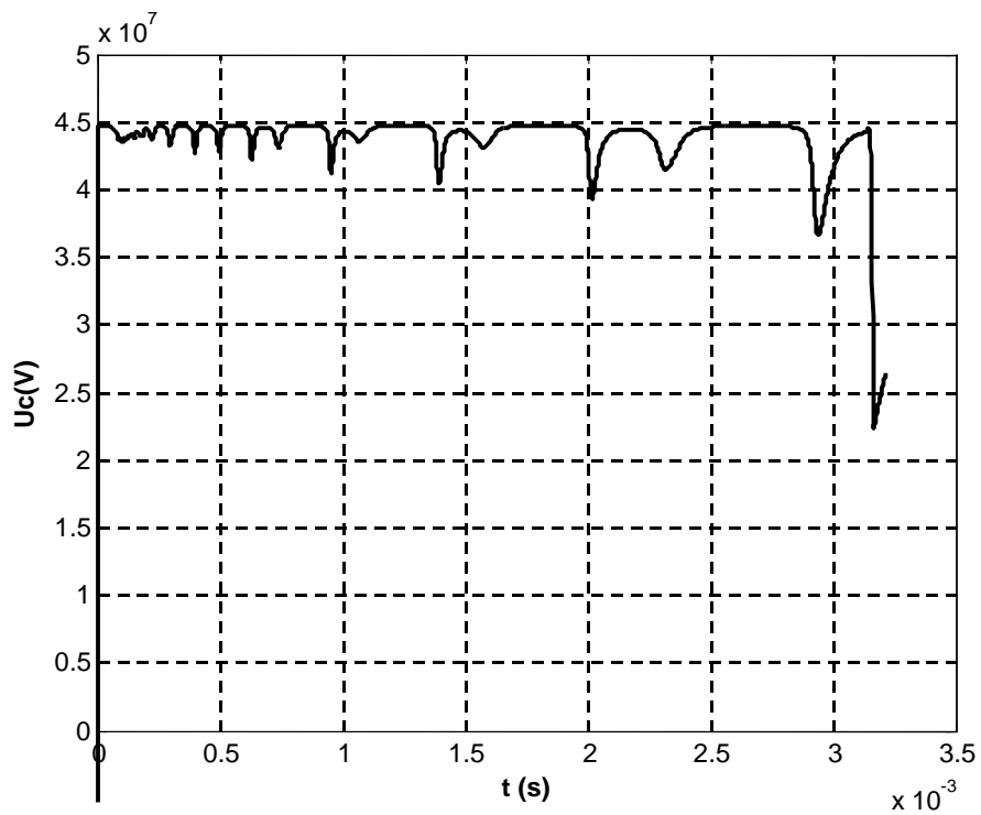
Figure 3.15.i : Tension appliquée dans l'intervalle d'air.
