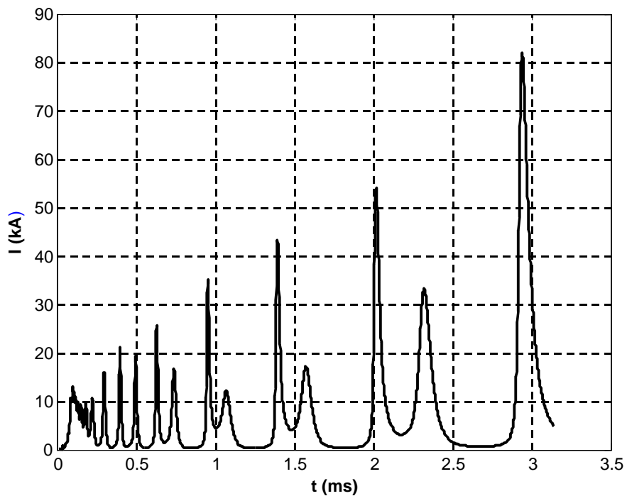
Figure 3.15.b : Courant dans le leader négatif d'électrode pendant la propagation.
