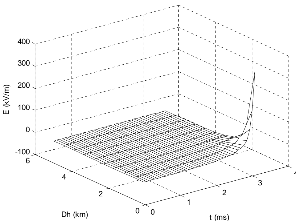
Figure 3.19: Champ électrique du leader à différentes distances de la décharge à différentes positions et en fonction du temps avant le début du saut final. Distance nuage – sol = 5000 m ; tension 45 MV.
