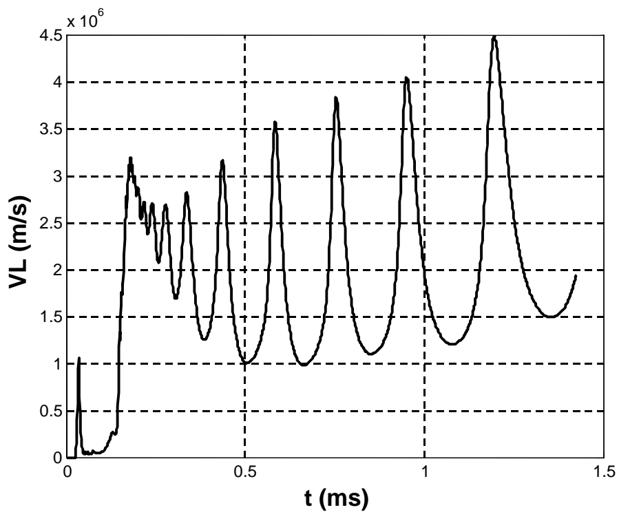
Figure 3.14.e : Vitesse instantanée du leader négatif d'électrode.
