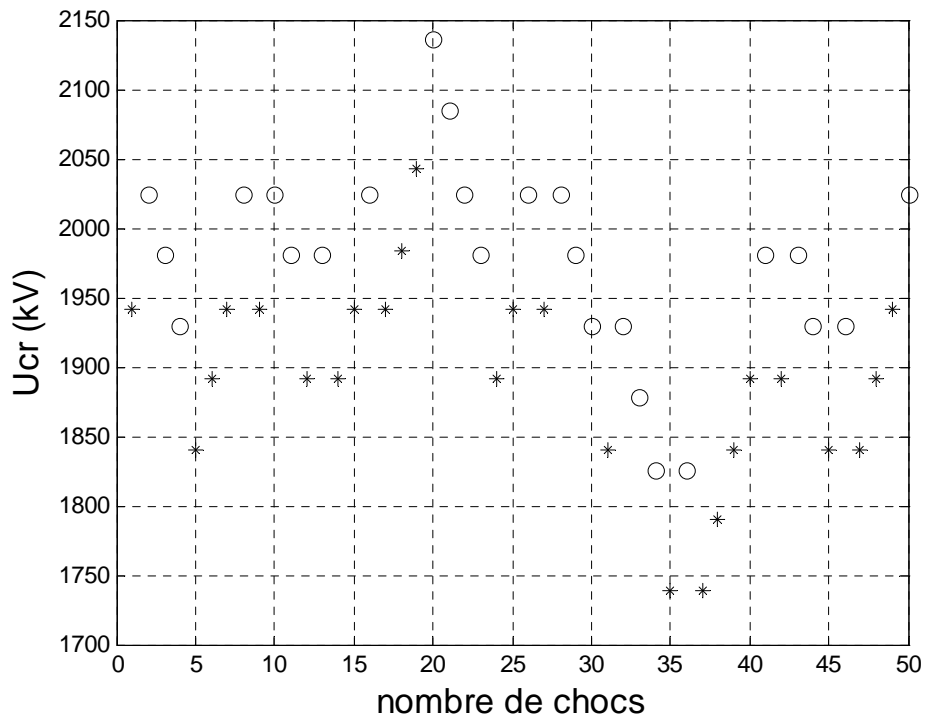
Figure 3.5: Une séquence "up and down". Intervalle D = 3 m. Onde 60/3000 \mu s . Les cas d'amorçage sont caractérisés par les points « o » et les cas de tenue par des astérix « * ». U_{50} = 1934,6 kV et \sigma = 3,0\% .
