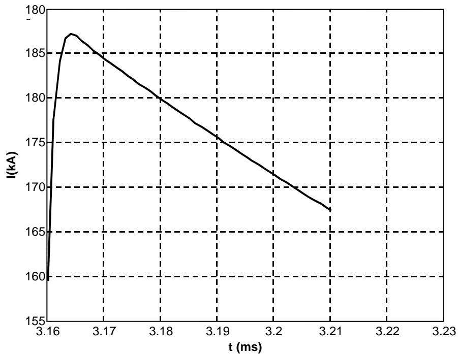
Figure 3.15.j : Courant de l'arc en retour.
