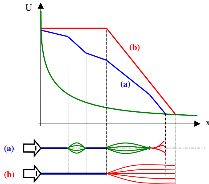
Figure 2.4: Distribution des potentiels avant (a) et après (b) la jonction entre le leader spatial et le leader négatif issu de l'électrode
