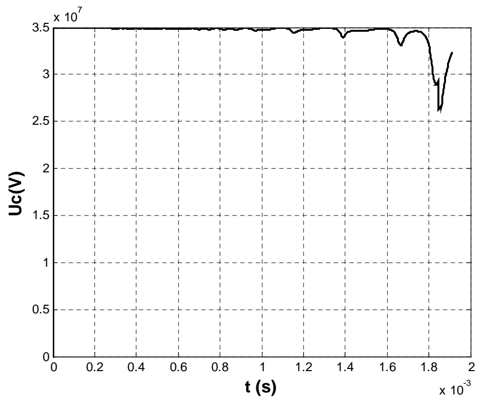
Figure 3.14.i : Tension appliquée dans l'intervalle d'air.
