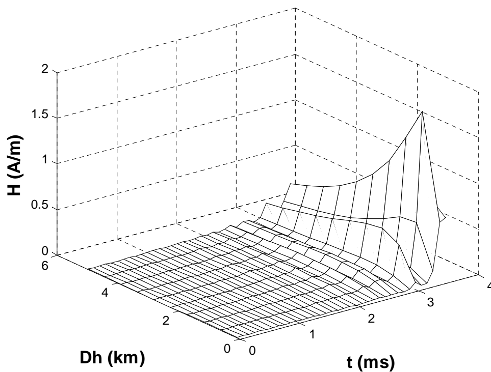
Figure 3.20: Champ magnétique rayonné par le leader négatif d'électrode en fonction de la position horizontale D_h avec l'axe de la décharge et en fonction du temps avant le début saut final. Distance nuage – sol = 5000 m ; tension 45 MV.
