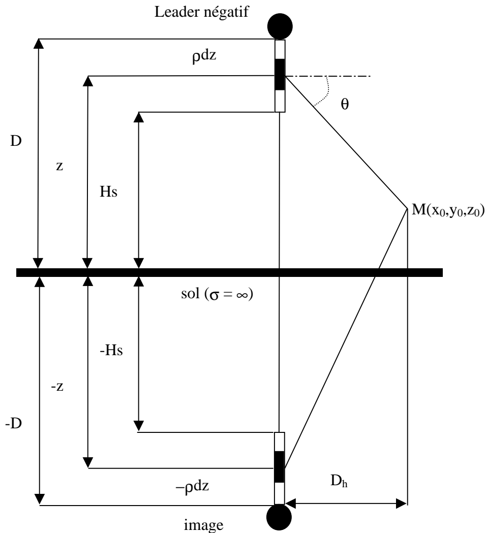
Figure 3.17 : Modèle géométrique simplifié utilisé calculant le champ électrique associé au leader [34]
