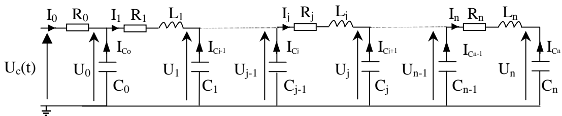
Figure 2.5 : Schéma électrique équivalent à la propagation de la décharge
