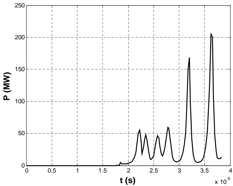
Figure 3.1.g : Puissance injectée dans l'intervalle
