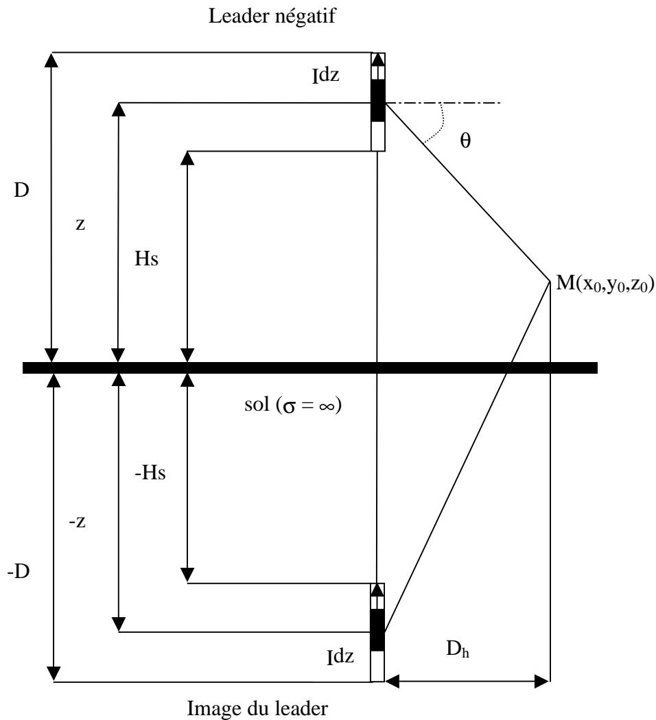
Figure 3.18 : Modèle géométrique simplifié utilisé calculant le champ magnétique associé au leader [34]
