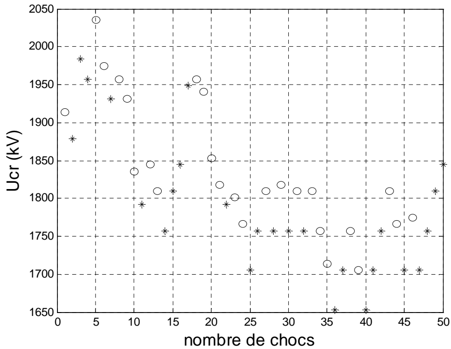
Figure 3.4: Une séquence "up and down". Intervalle D = 2,6 m. Onde 60/3000 \mu s. Les cas d'amorçage sont caractérisés par les points « o » et les cas de tenue par des astérisx « * ». U_{50} = 1813,9 kV et \sigma = 2,4\% .
