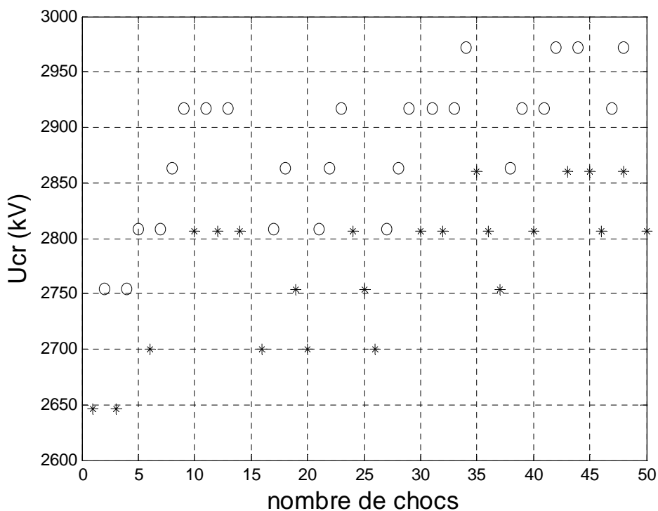
Figure 3.7: Une séquence "up and down". Intervalle D = 7 m. Onde 60/3000 \mu s. Les cas d'amorçage sont caractérisés par les points « o » et les cas de tenue par des astérix « * ». U_{50} = 2832,5 kV et \sigma = 3,9\% .
