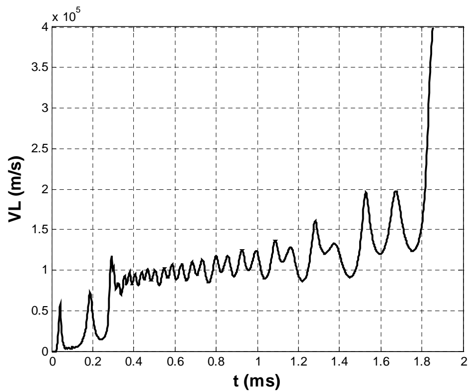
Figure 3.14.e : Vitesse instantanée du leader négatif d'électrode.
