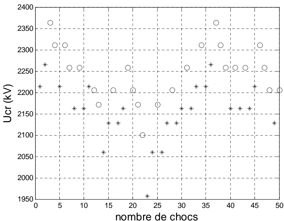
Figure 3.6: Une séquence "up and down". Intervalle D = 4 m. Onde 60/3000 \mu s. Les cas d'amorçage sont caractérisés par les points « o » et les cas de tenue par des astérix « * ». U_{50} = 2202 kV et \sigma = 3,4\% .
