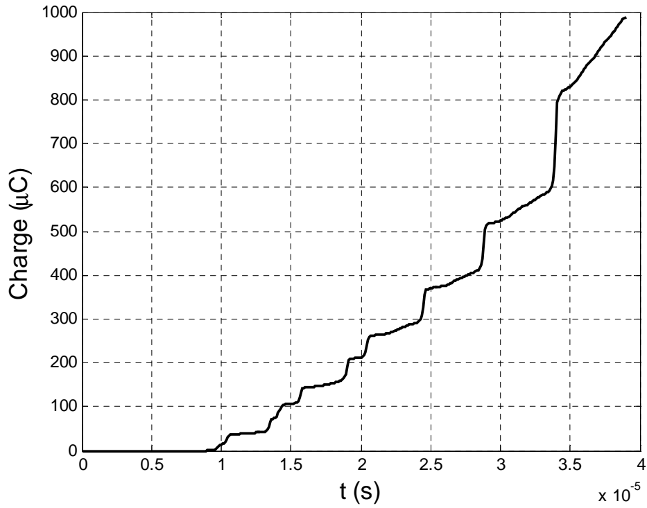
Figure 3.2.g: Charge injectée
