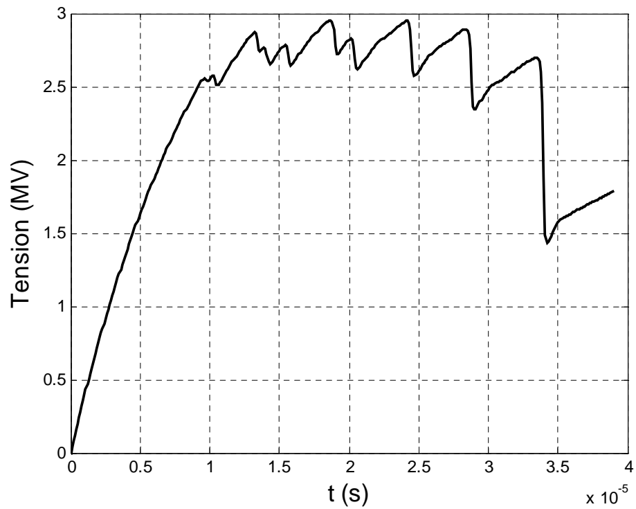
Figure 3.2.e: Tension appliquée.
