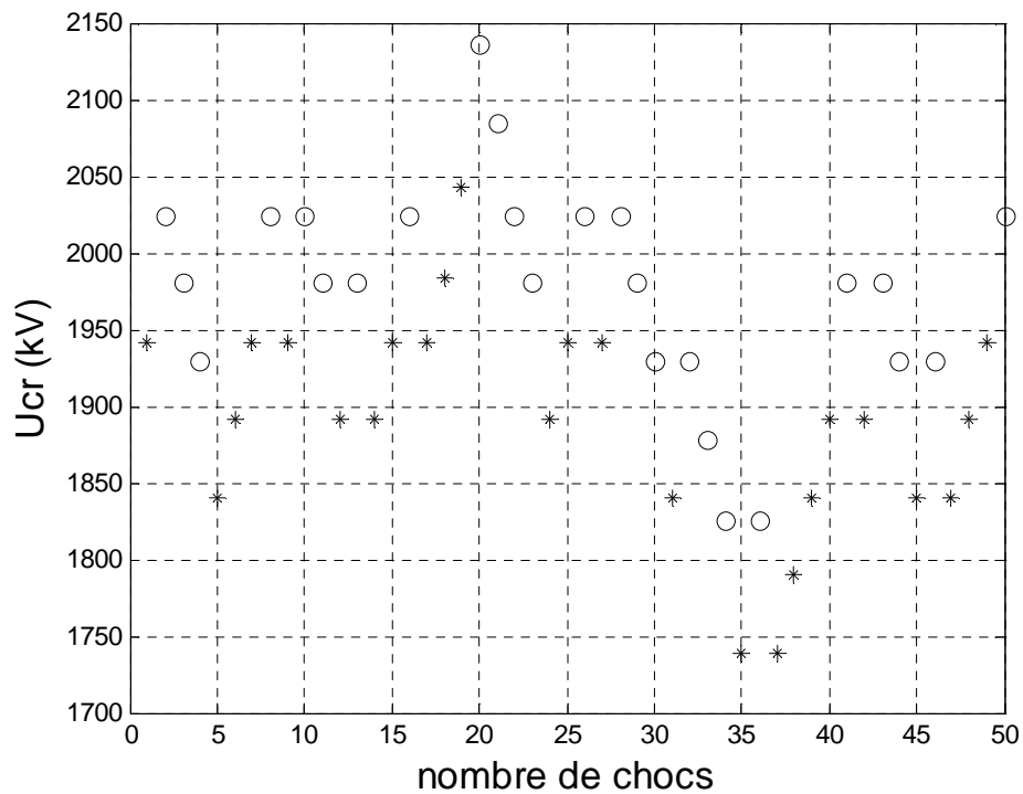
Figure 3.5: Une séquence "up and down". Intervalle D = 3 m. Onde 60/3000 \mu s. Les cas d'amorçage sont caractérisés par les points « o » et les cas de tenue par des astérisx « * ». U_{50} = 1934,6 kV et \sigma = 3,0\% .
