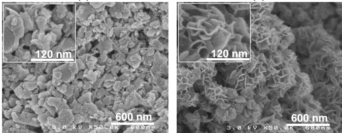
Figure III-14 : Clichés MEB focalisés sur les particules de l'additif au cobalt d'une électrode de Ni(OH) 2 avec 33% de Co(OH) 2 ajoutés, à l'état initial et après 30 cycles. Deux types de morphologie (a) et (b) sont observées sur la même électrode cyclée.
