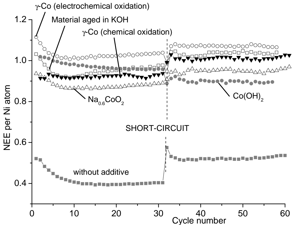
Figure III-11 : Evolution du nombre d'électrons échangés par atome de nickel, pour des électrodes à base de \text{Ni}(\text{OH})_2 , sans additif conducteur ou avec 33 % d'additif ajouté. Les cinq additifs étudiés sont : \text{Na}_{0,6}\text{CoO}_2 , matériau issu du vieillissement de \text{Na}_{0,6}\text{CoO}_2 dans \text{KOH} , \gamma\text{-Co} obtenues par oxydation électrochimique ou chimique de \text{Na}_{0,6}\text{CoO}_2 , \text{Co}(\text{OH})_2 jouant le rôle d'additif de référence.
