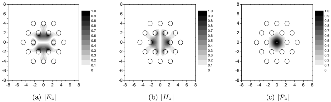
FIG. 7.18 – Cartes de champs normalisés du mode fondamental de classe C4 à deux couches d'inclusions pour \lambda = 1.56 \mu m , N = 60 et L_1 = 20 . n_{eff} = 1.42103506 + i2.36433 \cdot 10^{-5}
