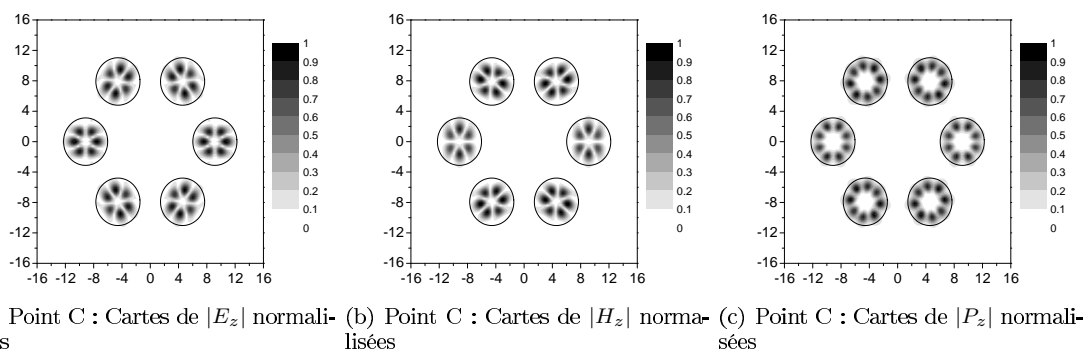
FIG. 7.52 – Cartes de champs calculées par la MD pour les points C de la figure 7.48 à \lambda = 0.598 \mu\text{m}
