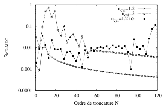
FIG. 3.25 – Convergence selon N de \tau_{MD-MDC}
