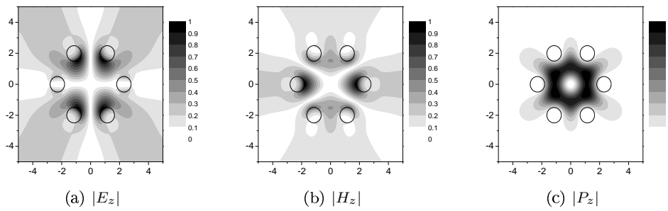
FIG. 7.12 – Cartes de champs normalisés du mode C6-a pour \lambda = 1.56 \mu\text{m} , N = 60 et L = 25 . n_{eff} = 1.38686852 + i5.03490 \cdot 10^{-3}
