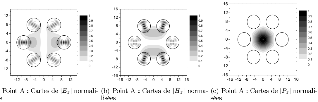
FIG. 7.50 – Cartes de champs calculées par la MD pour les points A de la figure 7.48 à \lambda = 0.55 \mu\text{m}
