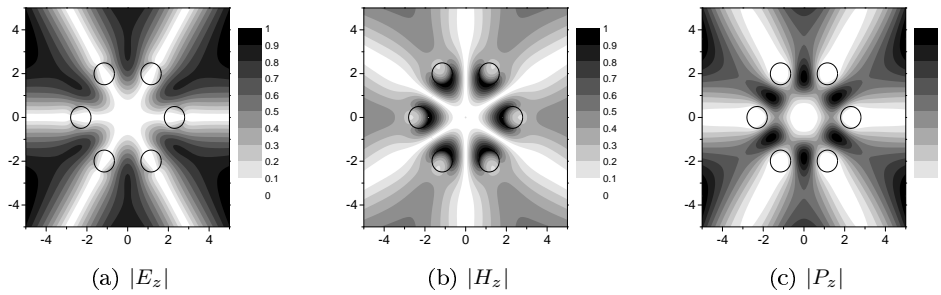
FIG. 7.14 – Cartes de champs normalisés du mode C8-a pour \lambda = 1.56 \mu\text{m} , N = 60 et L = 25 . n_{eff} = 1.35131984 + i2.15436 \cdot 10^{-2}
