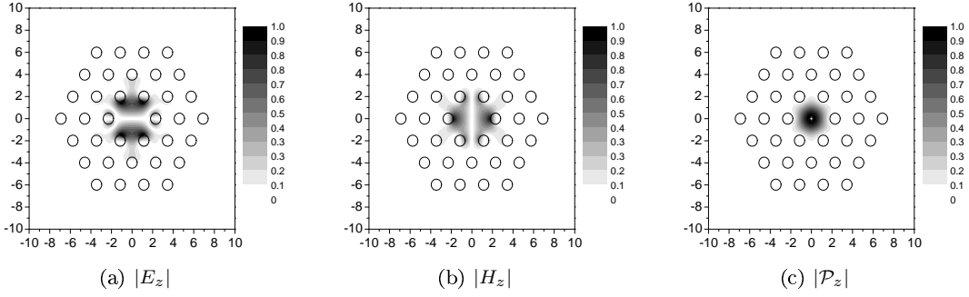
FIG. 7.19 – Cartes de champs normalisés du mode fondamental de classe C4 à trois couches d'inclusions pour \lambda = 1.56 \mu\text{m} , N = 60 et L_1 = 20 . n_{eff} = 1.4210445 + i7.928 \cdot 10^{-7}
