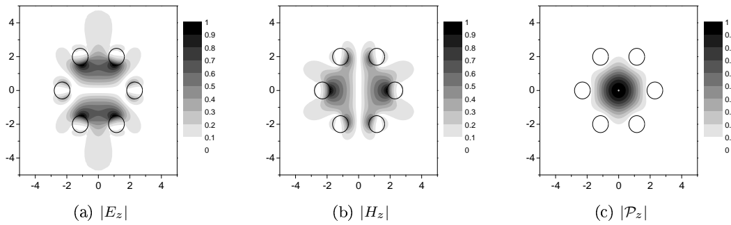
FIG. 7.4 – Cartes de champs normalisés du mode fondamental C4\text{-a} pour \lambda = 1.56 \mu\text{m} , N = 60 , L_1 = L_2 = 10 et L_3 = 5 . n_{eff} = 1.42078315 + i7.20465 \cdot 10^{-4}
