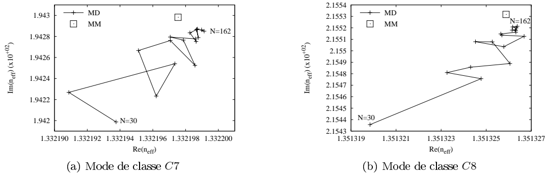
FIG. 7.13 – Indice effectif des modes C7-a et C8-a en fonction de N pour \lambda = 1.56 \mu\text{m} et L = 25
