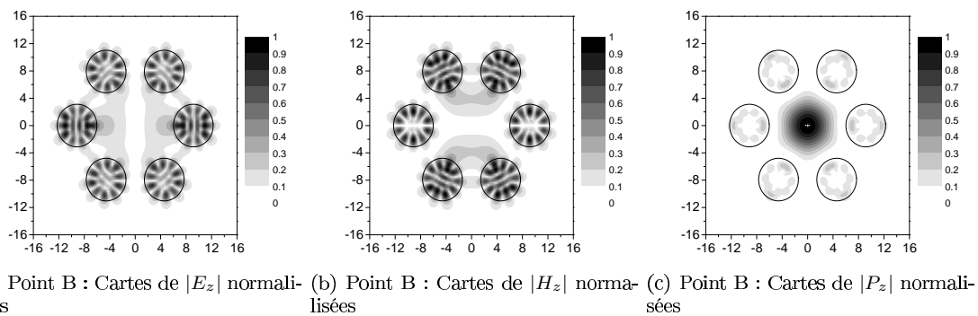
FIG. 7.51 – Cartes de champs calculées par la MD pour les points B de la figure 7.48 à \lambda = 0.5926 \mu\text{m}
