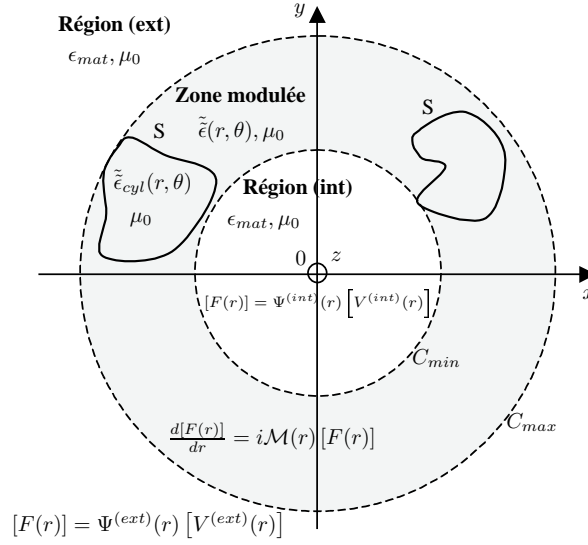
FIG. 5.6 – Généralisation de la méthode différentielle à des milieux anisotropie : cas des cylindres excentrés par rapport à l'origine
