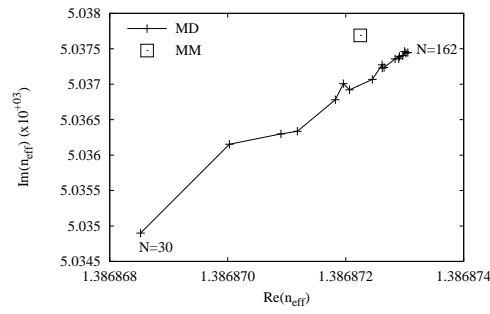
FIG. 7.11 – Indice effectif du mode de classe C5/6 en fonction de N pour \lambda = 1.56 \mu\text{m} et L = 25
