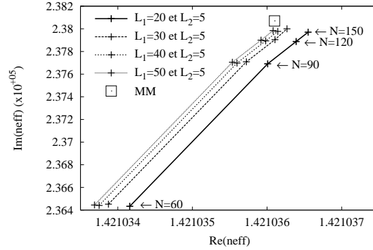
FIG. 7.16 – Convergence selon N de l'indice effectif du mode fondamental d'une FOM à deux couches d'inclusions dans le plan complexe, pour différentes valeurs de L_1 et \lambda = 1.56 \mu m . La valeur trouvée par la MM est également représentée.
