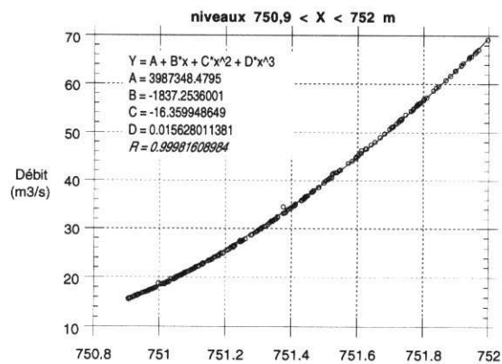
Fig. 28 Courbe de tarage des débits à l'exutoire du lac
