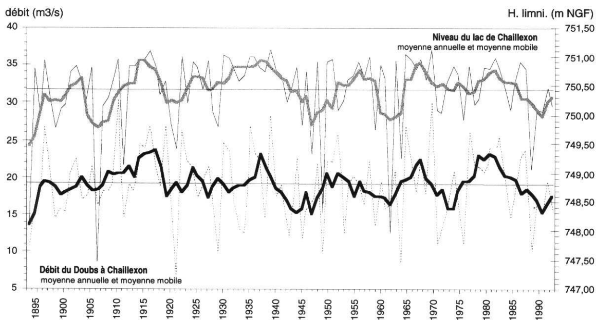
Fig. 38 Moyennes annuelles (et moyenne mobile sur 5 ans) des débits du Doubs et des niveaux du lac (1893-1993)
