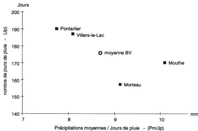
Fig. 11 Indice de précipitation et jours de pluies dans le bassin versant (moyenne interannuelle).
