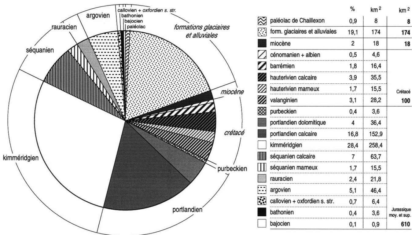
Fig. 17 répartition des surfaces d'affleurement par étages
