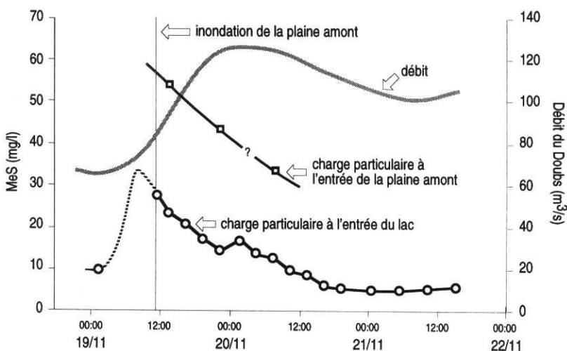
Fig. 68 Différence de charge particulaire dans les eaux du Doubs à l'entrée du lac (Villers-le-Lac) et à l'amont de la plaine de Morteau (Pont de la Roche) lors de la crue inondante de novembre 1992
