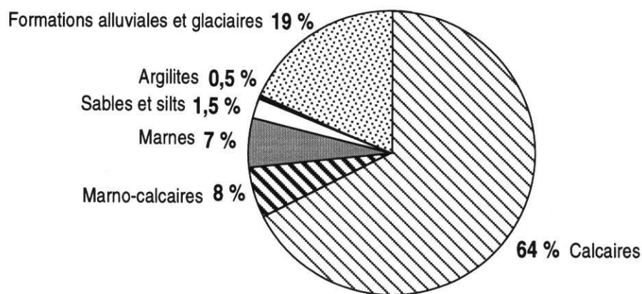
Fig. 18 Répartition des différents faciès pétrographiques du BV
