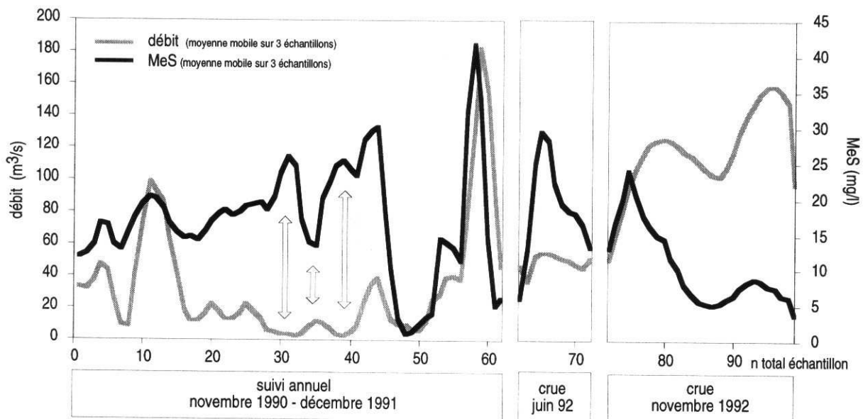
Fig. 55 évolution des moyennes mobiles (sur 3 échantillons) du débit et de la charge en MeS à Villers-le-Lac au cours de l'échantillonnage.
