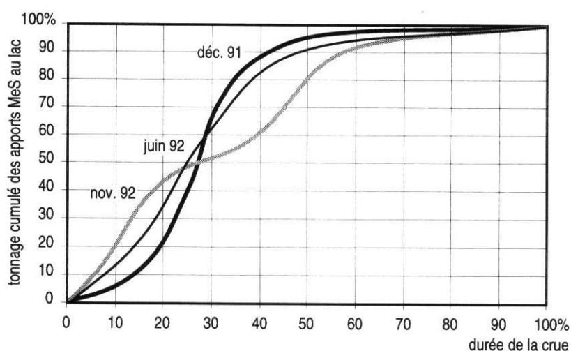
Fig. 59 Tonnage cumulé des apports particuliers en période de crue
