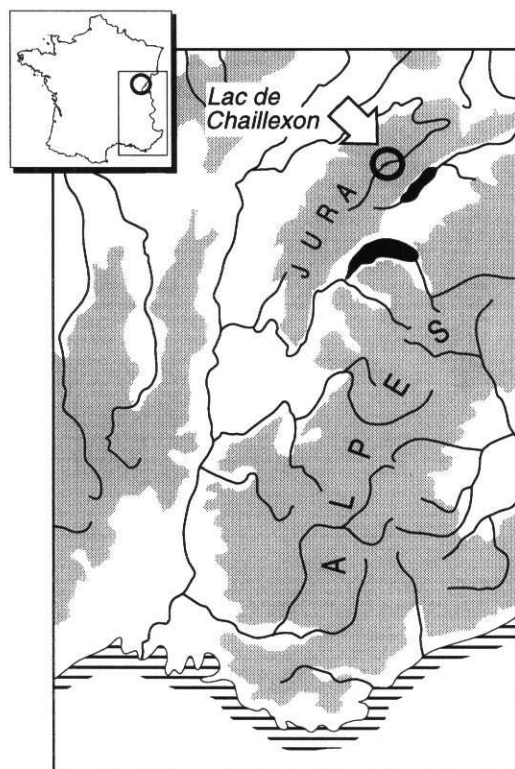
Fig. 1 Localisation du lac de Chaillexon et de son bassin versant
