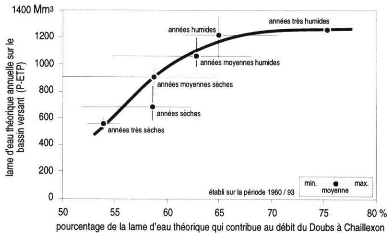
Fig. 44 Contribution théorique du bassin versant aux flux hydrologiques à l'entrée du lac
