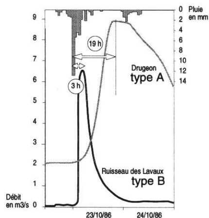
Fig. 69 Réponses hydrologiques de deux types différents de SBV soumis à une averse identique (le comportement du type C est intermédiaire).
