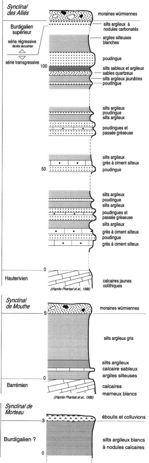
Fig. 16 Log stratigraphique synthétique du bassin versant (d'après cartes BRGM et Pharissat et al., 1986)
