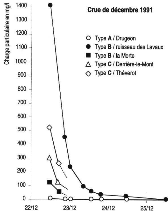
Fig. 70 Charge particulaire des SBV lors de la crue de décembre 1991
