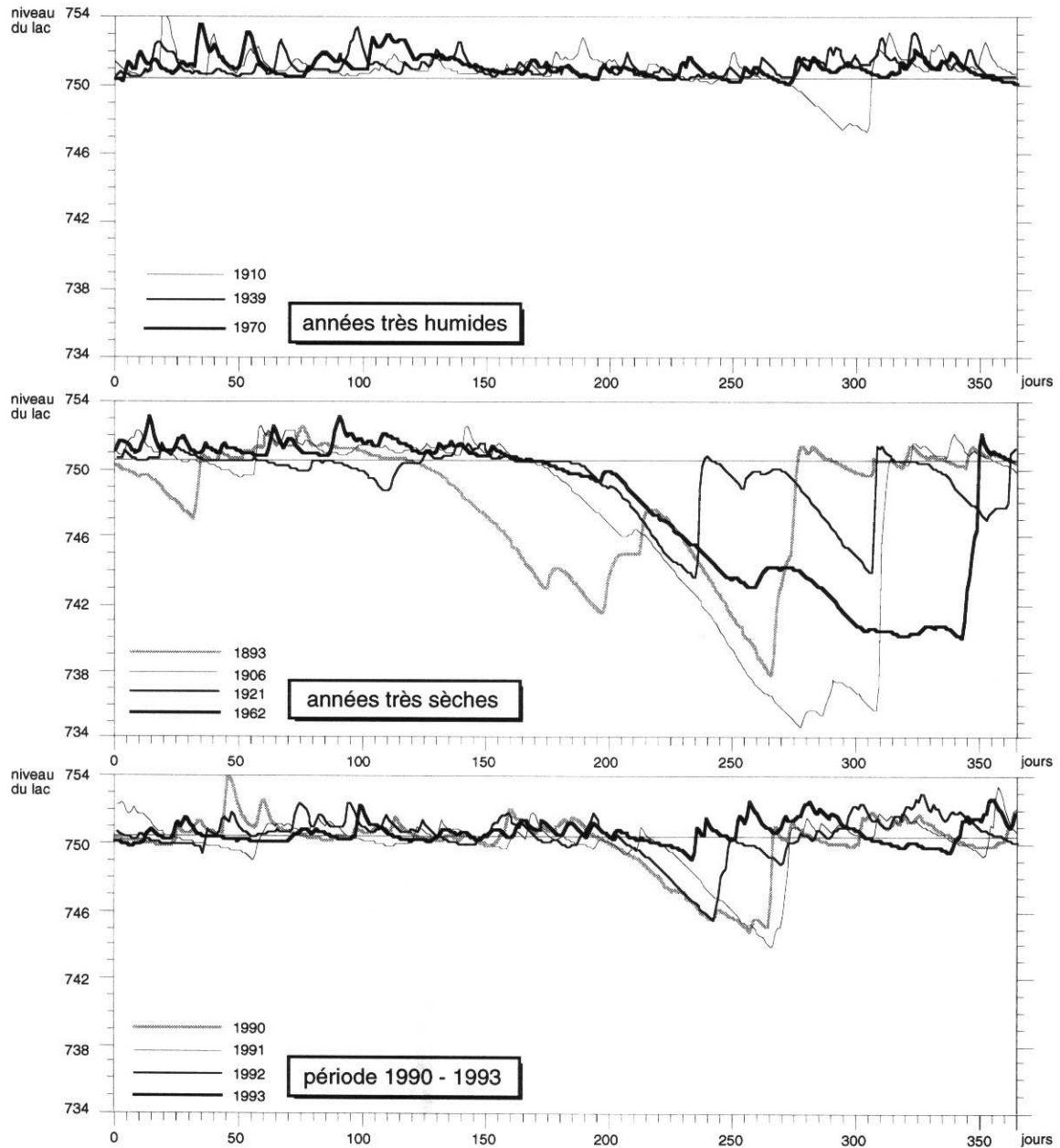
Fig. 41 Limnigrammes annuels du niveau du lac (années extrêmes et période 1990-1993)
