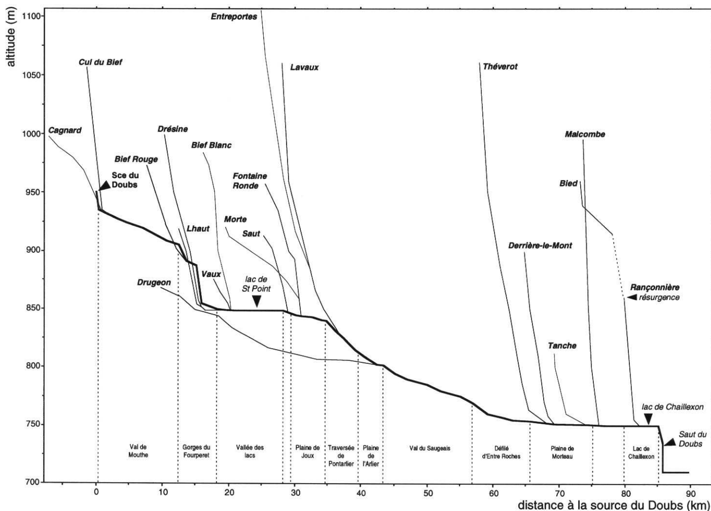
Fig. 5 Profil longitudinal du réseau hydrographique
