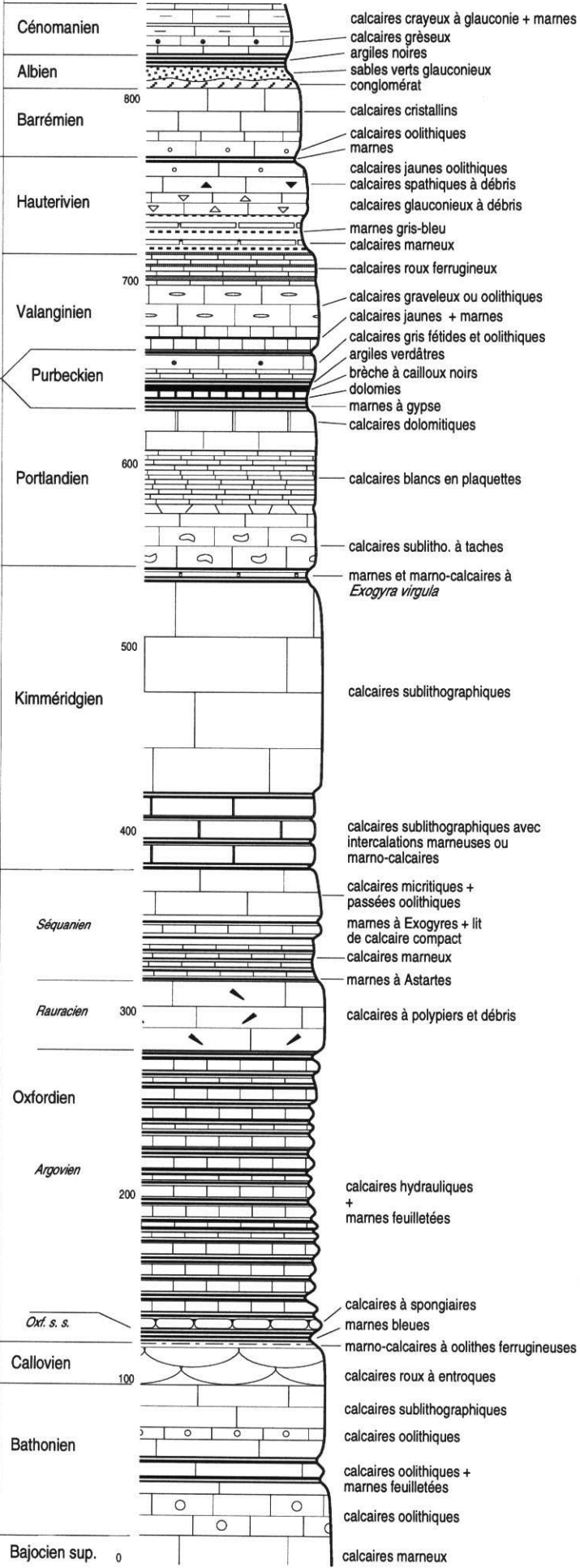
Fig. 16 Log stratigraphique synthétique du bassin versant (d'après cartes BRGM et Pharissat et al., 1986)
