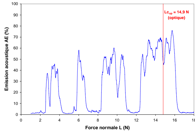
Figure VI.11 : Emission acoustique lors du test de rayure du revêtement multicouches CrN/Cr-C de bipériode 200 nm sur acier SS304L
