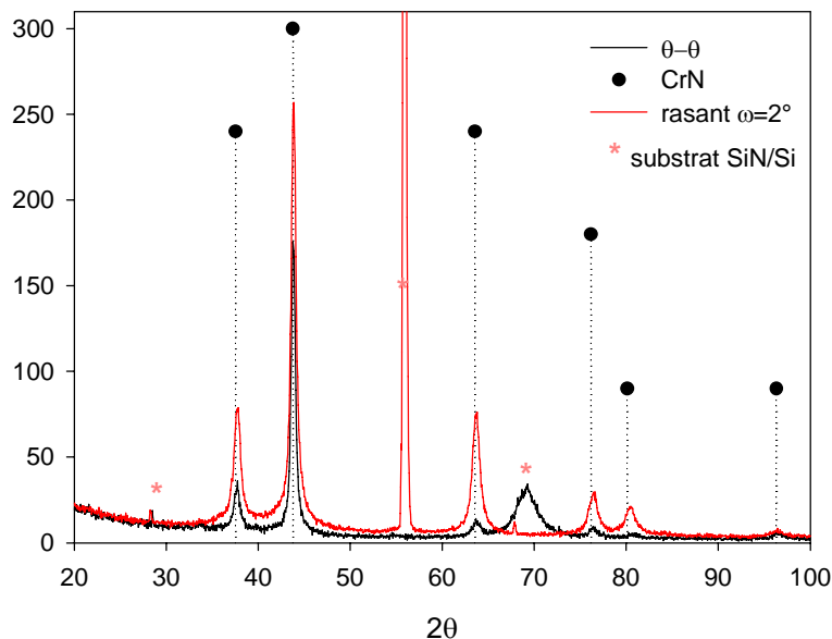
Figure V.27 : Diagrammes DRX en configuration symétrique (en noir) et en configuration rasante (en rouge) d'un revêtement multicouches CrN/Cr-C de bipériode 50 nm sur substrat SiN/Si
