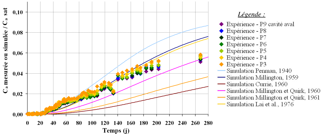
Figure 93 - Sensibilité des transferts en sable non saturé modélisés aux formules décrivant la tortuosité
