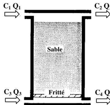
Figure 14 - Dispositif expérimental de Batterman et al., 1996
