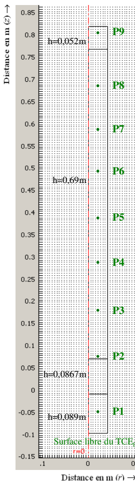
Figure 80 - Géométrie du modèle de dimensionnement sous Comsol
