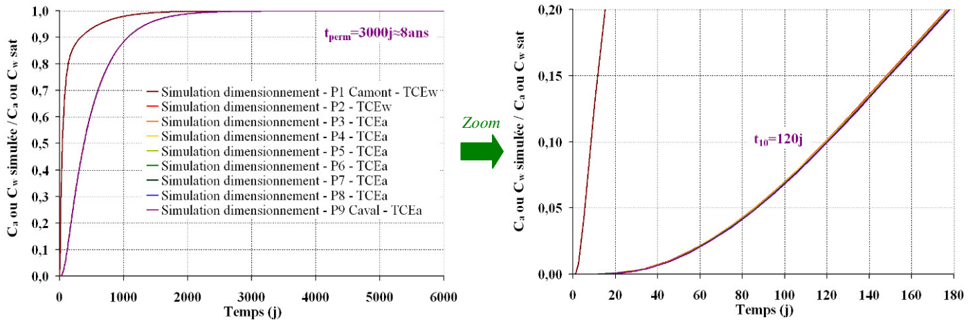
Figure 81 - Evolution temporelle simulée des concentrations en TCE_a ou en TCE_w aux points de prélèvements
