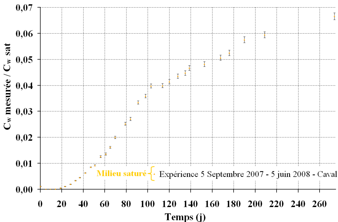
Figure 119 - Courbe des concentrations en cavité aval avec incertitudes de mesure - essai de diffusion aqueuse
