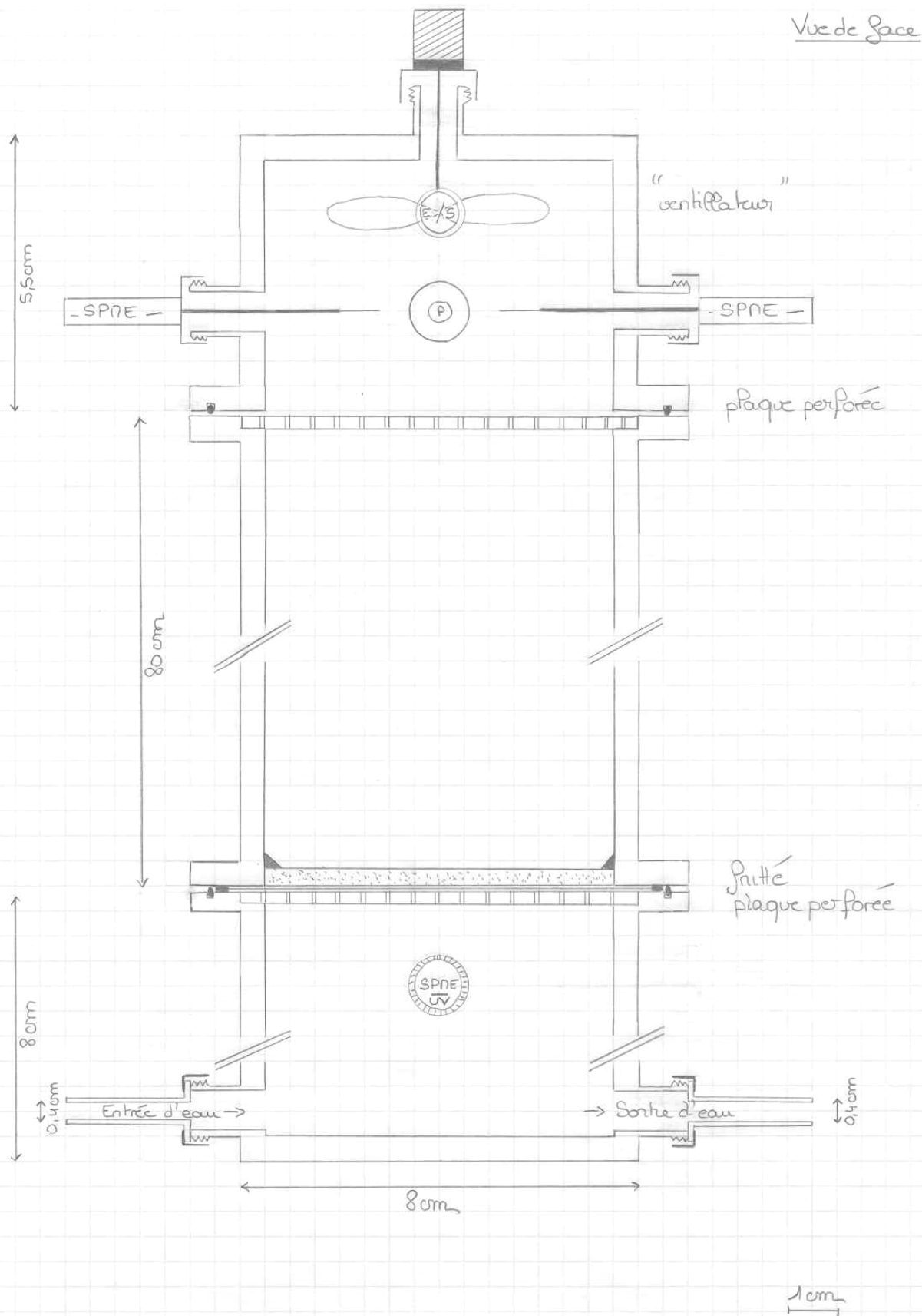
Figure 99 - Vue de face : cavité amont + colonne + cavité aval correspondant à un terme source de TCE_w
