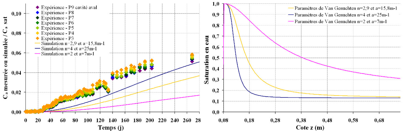
Figure 94 - Sensibilité des transferts en sable non saturé modélisés au profil de teneur en eau
