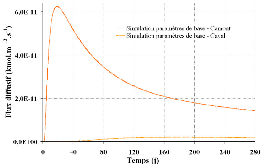
Figure 122 - Flux diffusif simulé - essai de diffusion aqueuse
