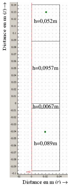
Figure 64 - Géométrie
