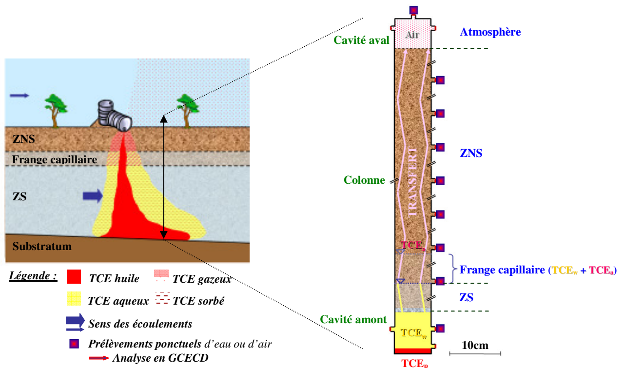
Figure 79 - Schématisation du dispositif utilisé lors de l'expérience de transfert
