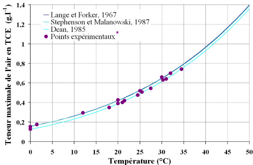
Figure 33 - Sensibilité de la pression de vapeur saturante du TCE à une variation de température (inspiré de Mendoza et al., 1990)
