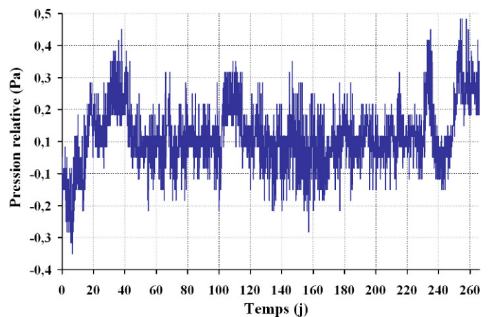
Figure 86 - Suivi de la pression - essai de transfert de TCE
