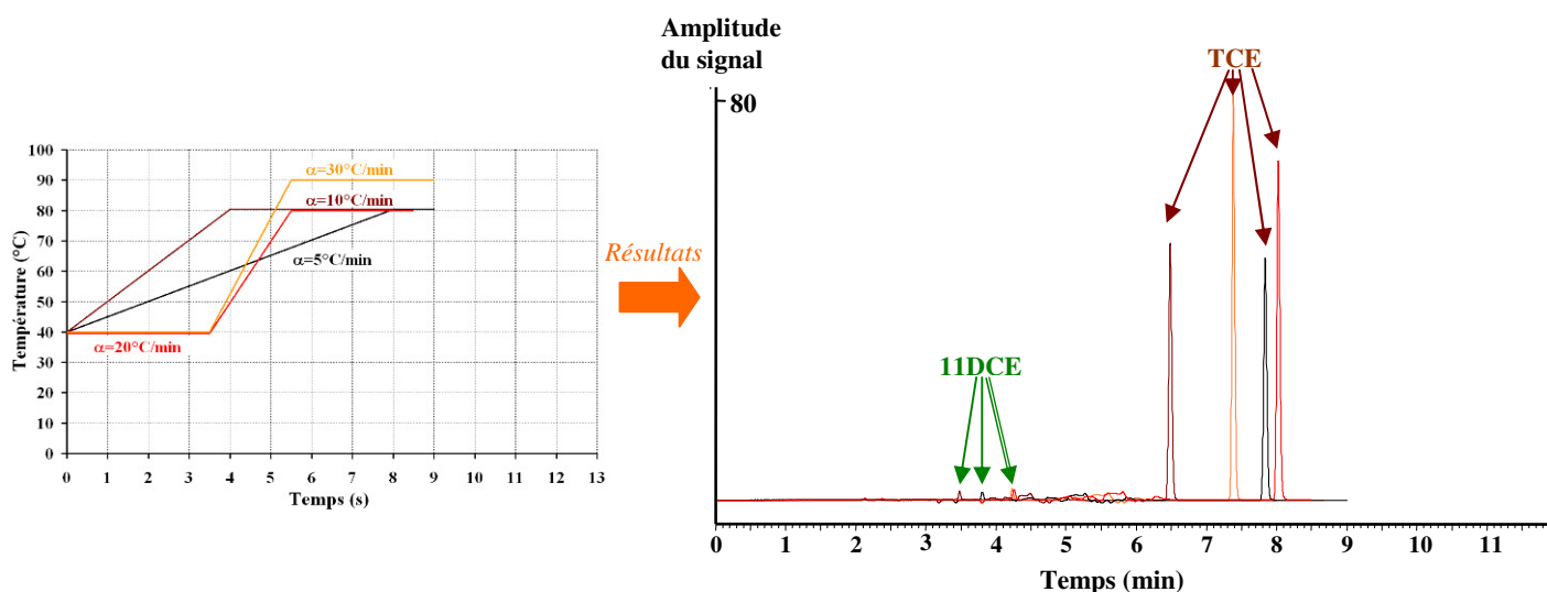
Figure 106 - Programmations non isothermes 40/80 ou 90 du four testées en relation avec les résultats d'analyse
