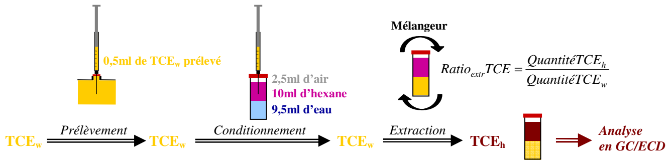
Figure 46 - Etapes à mettre au point pour l'analyse d'échantillons de TCE w
