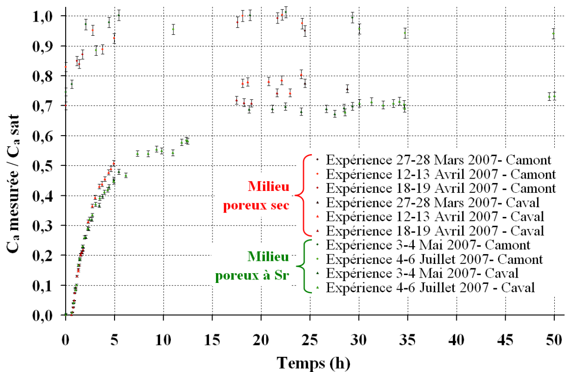
Figure 120 - Courbe des concentrations en cavité aval avec incertitudes de mesure - essais de diffusion gazeuse
