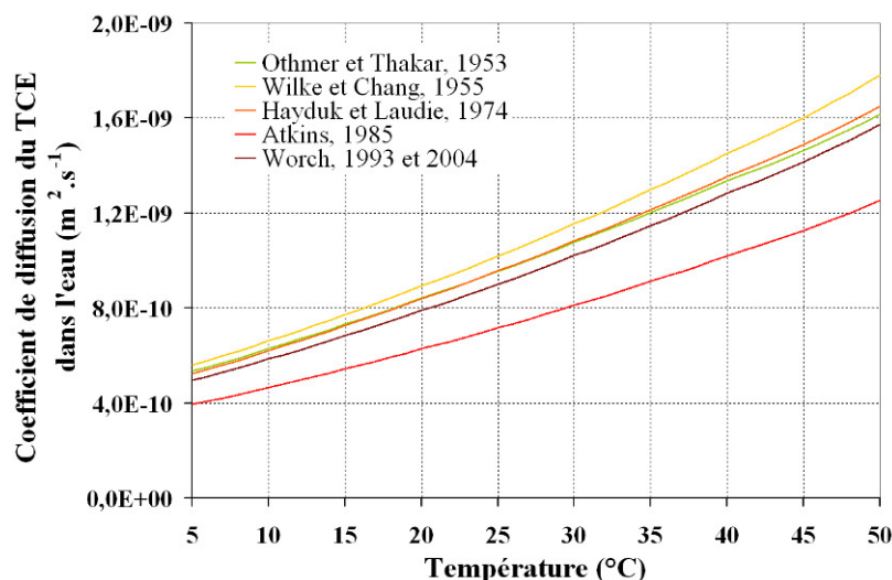
Figure 25 - Sensibilité du coefficient de diffusion du TCE w dans l'eau libre à une variation de température (inspirée de Grathwohl, 1998)
