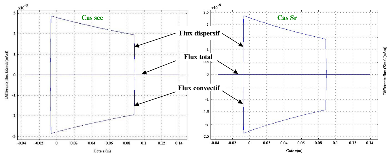
Figure 126 - Divers flux au régime permanent (couplage des deux équations) - essais de diffusion gazeuse en milieu sec et à Sr
