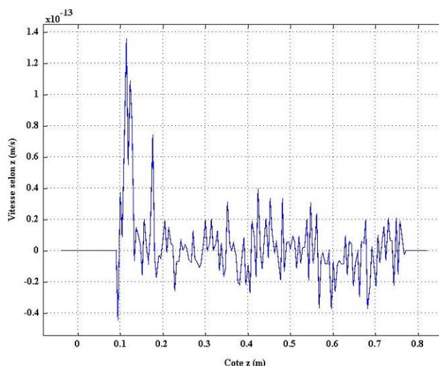
Figure 134 - Vitesses au régime permanent (équation de l'écoulement seule) - essai de transfert de TCE w et TCE a
