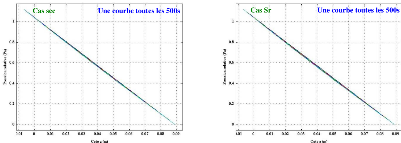
Figure 132 - Evolution du profil de pression relative en fonction du temps - essais de diffusion gazeuse en milieu sec et à Sr
