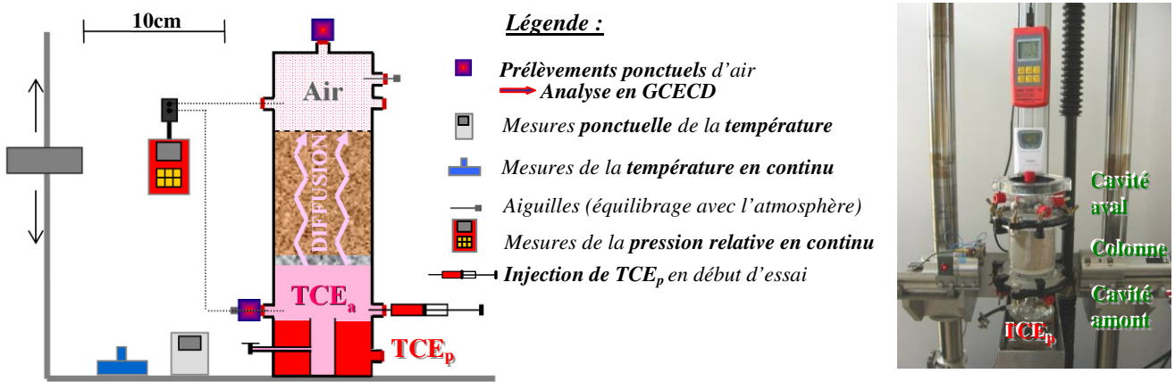
Figure 68 - Schématisation et photo du montage des essais de diffusion gazeuse
