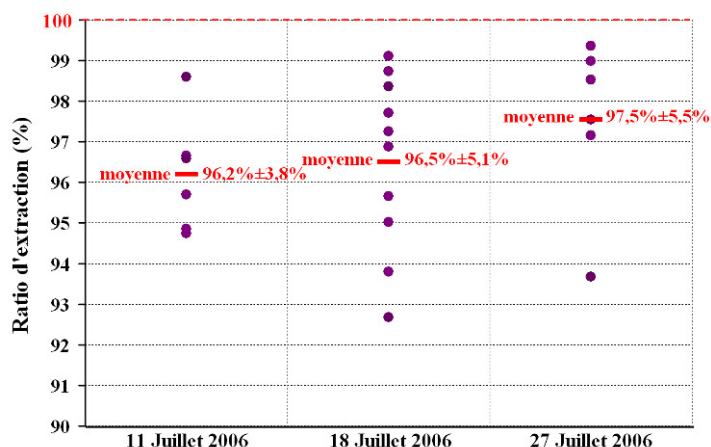
Figure 47 - Séries d'extraction d'échantillons subissant exactement le même traitement que ceux issus des essais
