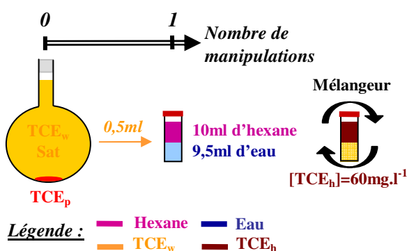
Figure 47 - Séries d'extraction d'échantillons subissant exactement le même traitement que ceux issus des essais
