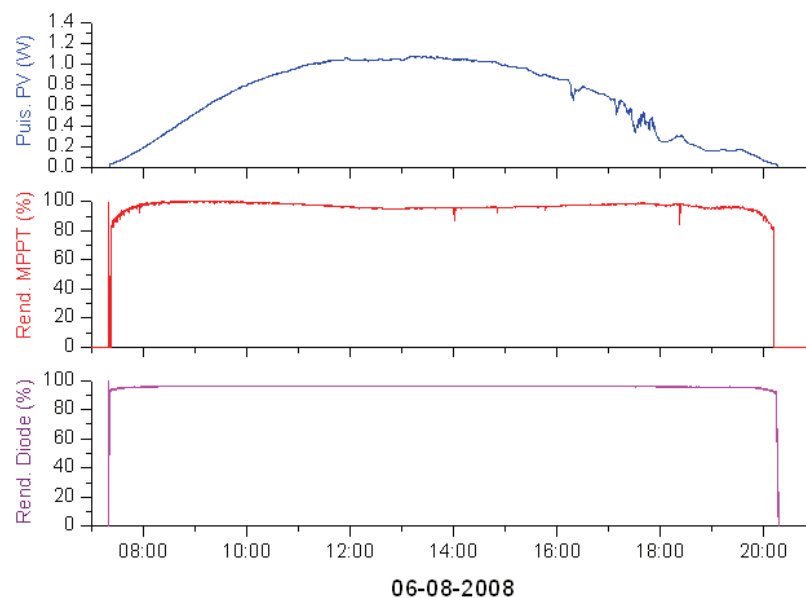
Figure 5-16. Puissance P_{PV} et rendements \eta_{MPPT} et \eta_{conv} d'un GPV référencé 14/150/300TD connecté directement avec diode anti-retour à une batterie de 6V.
