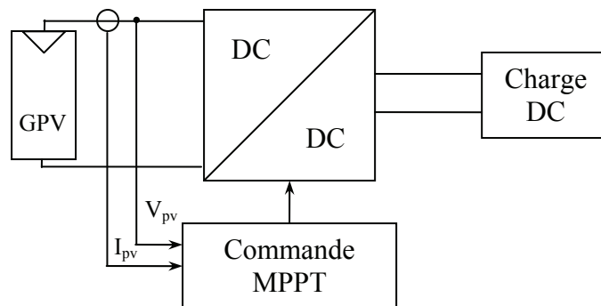
Figure 3-9. Chaîne de conversion photovoltaïque avec convertisseur DC/DC contrôlé par une commande MPPT sur charge DC.
