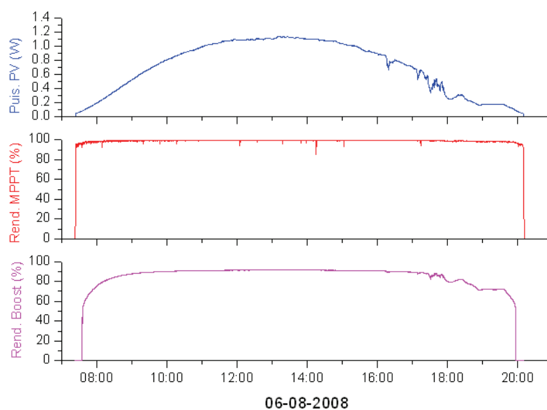
Figure 5-17. Puissance P_{PV} et rendements \eta_{MPPT} et \eta_{conv} d'un GPV référencé 14/150/300TD connecté avec un étage d'adaptation Boost et MPPT à une batterie de 6V
