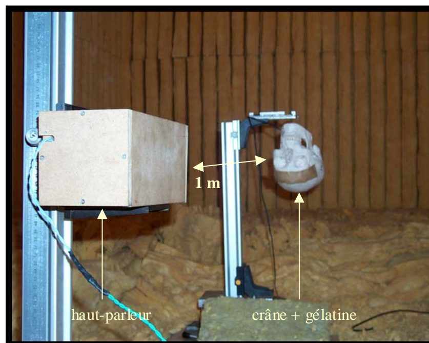
Fig. 35 : Photographie du montage expérimental de localisation du son par un crâne humain. Le haut-parleur et le crâne (rempli de gélatine tenant lieu de cerveau) sont distants de 1 mètre. L'expérience s'effectue en chambre anéchoïque pour isoler les effets de réverbération de la boîte crânienne.
