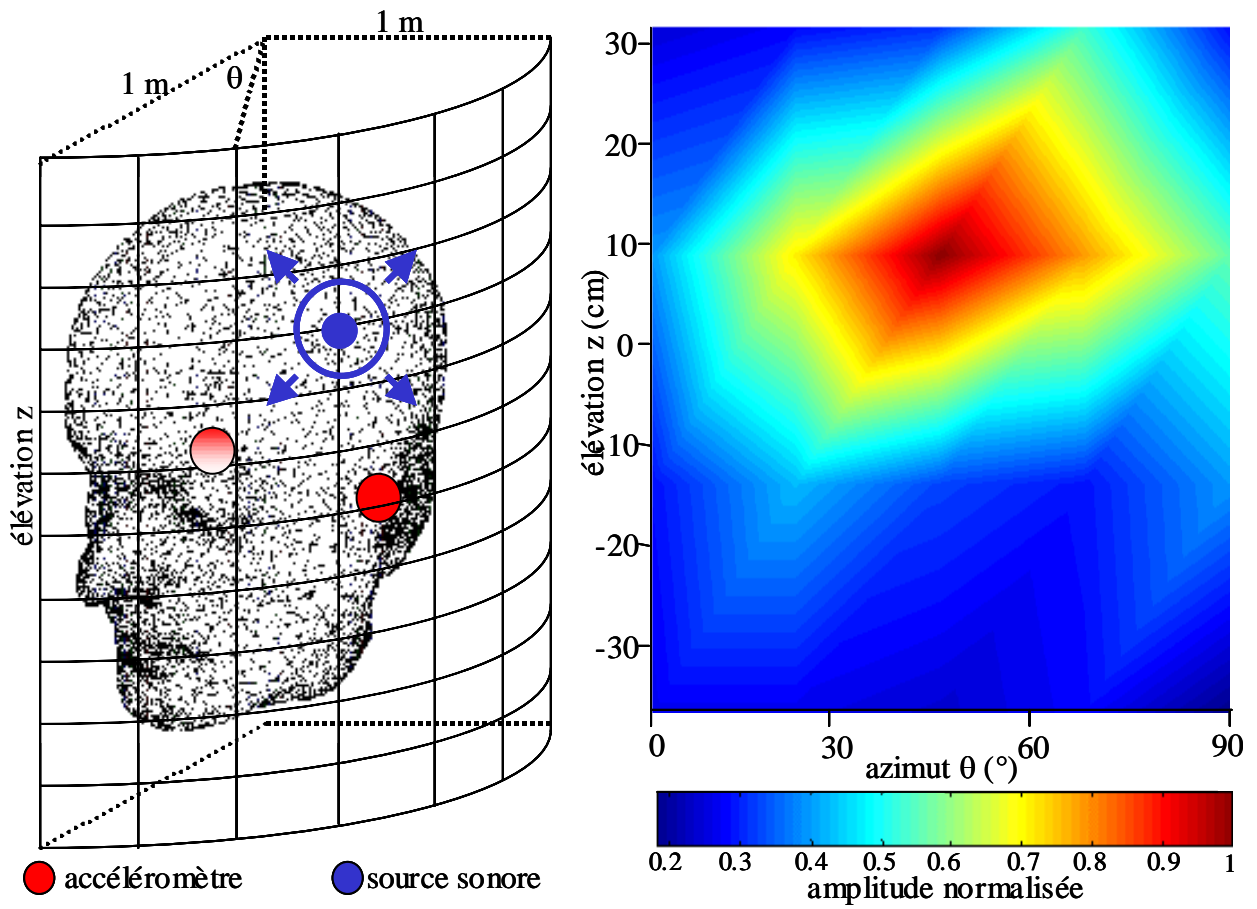
Fig. 36 : Résultat expérimental de focalisation en réception. Le maximum de la tache focale se situe exactement sur la position de la source en azimut ( 45^\circ ) et en élévation (10 cm).
