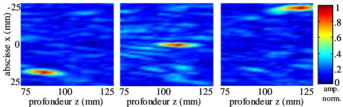
Fig. 22 : Résultat expérimental de focalisation spatiale du champ acoustique avec un unique transducteur ultrasonore. La forme de cigare de la tache focale obéit aux lois de la diffraction d'une ouverture équivalente à la face avant de la cavité réverbérante.
