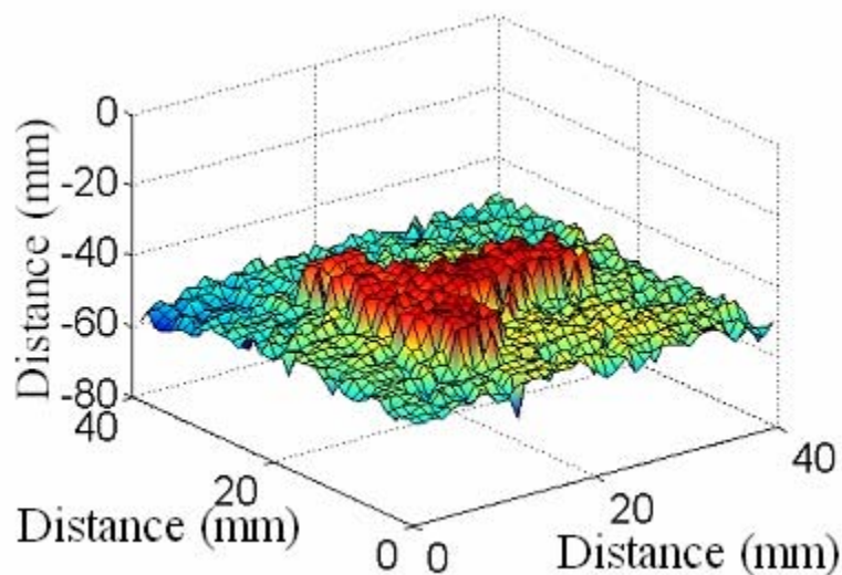
Fig. 31 :Image du relief d'un objet en « T » obtenu par écholocation avec un kaleidoscope couplé à 31 transducteurs ultrasonores. L'imagerie harmonique permet de résoudre le problème posé par la réverbération de la cavité lors de la phase de réception (Image gracieusement prêtée par Delphine Palacio).
