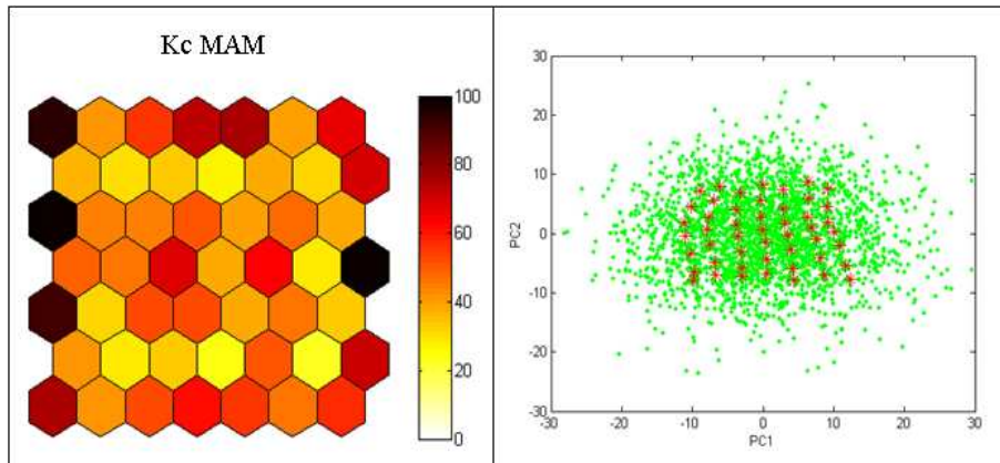
FIGURE 4.11 – Résultat de la méthode neuronale dans la région 10^{\circ}\text{N} - 30^{\circ}\text{S} ; 50 - 80^{\circ}\text{W} . A gauche, la projection de tous les jours de MAM de la période d'étude sur la Kc; à droite, la projection des 49 neurones sur l'espace bidimensionnel des deux composantes principales d'une ACP sur u850 et v850.
