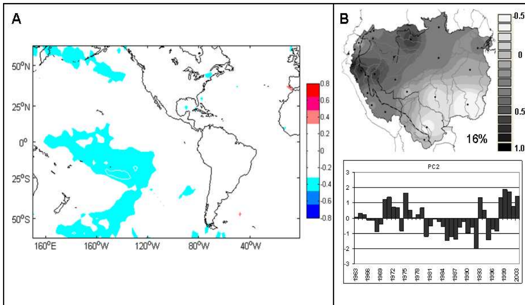
FIGURE 3.43 – Comme pour les Figures 3.30 mais en MAM.
