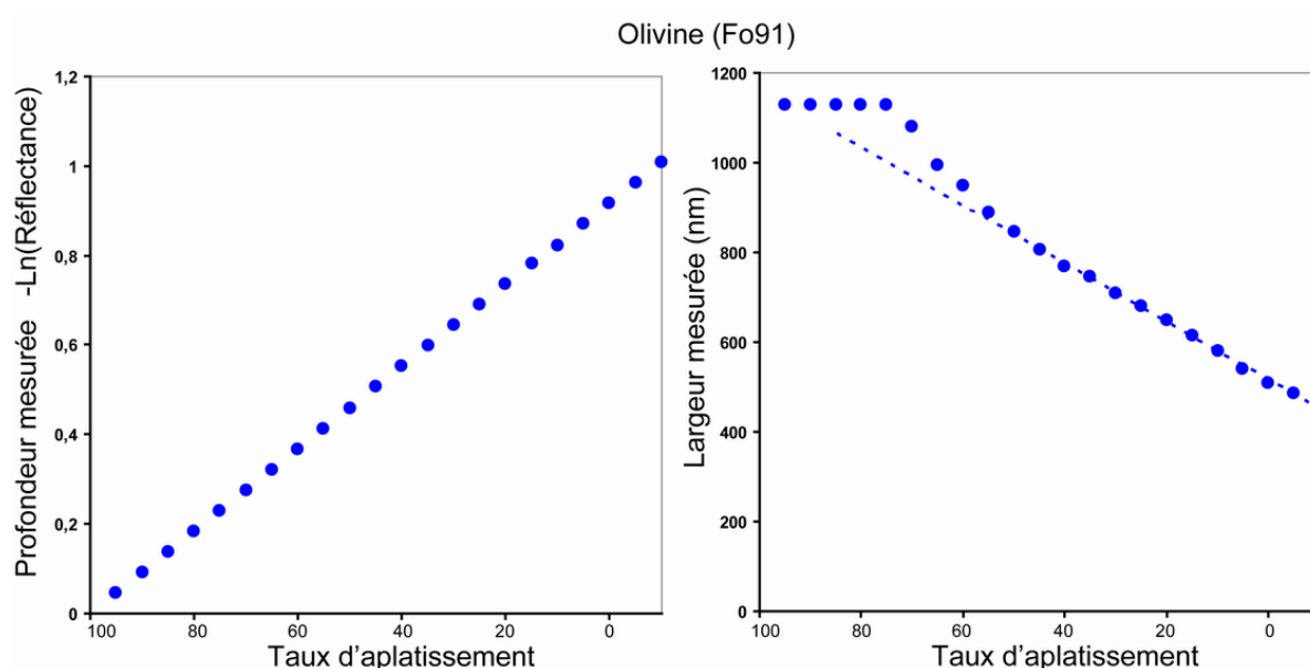
FIG. 5.42 – Evolution des profondeurs et largeurs mesurées en fonction du taux d'aplatissement du spectre. Exemple pour le cas d'un spectre d'olivine (Fo91).
