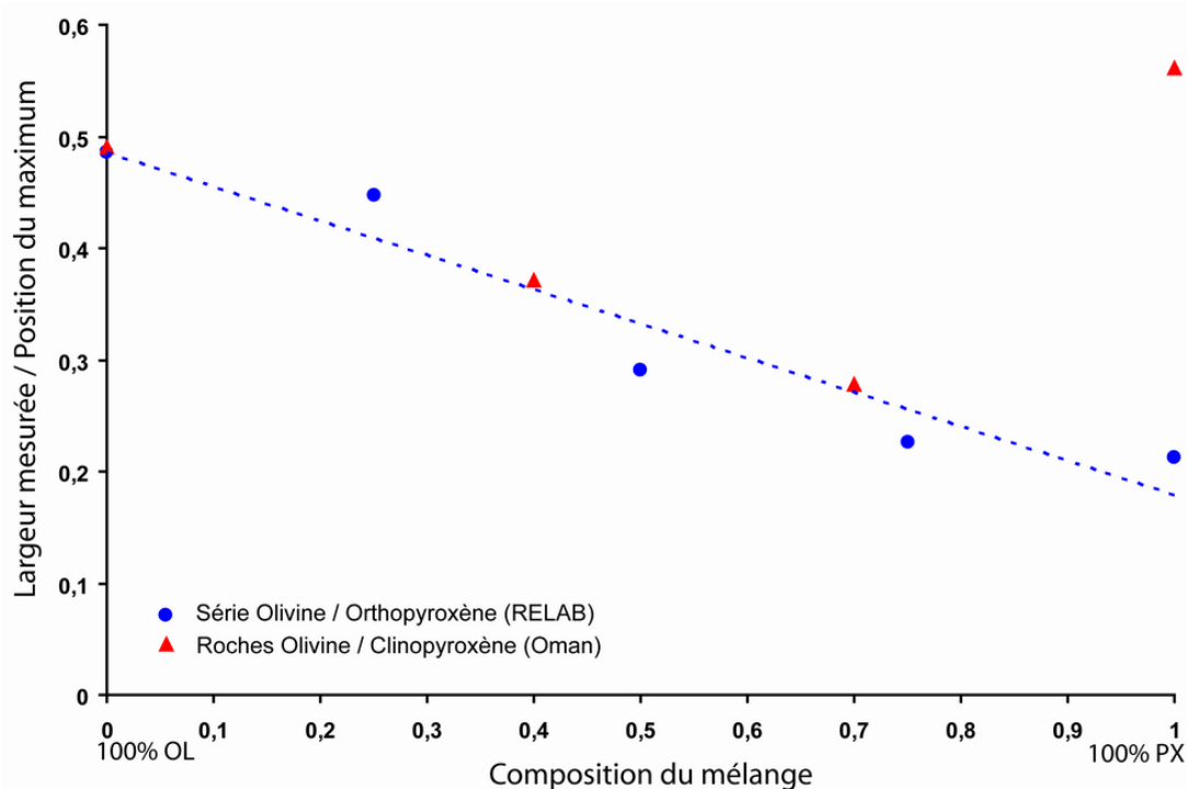
FIG. 5.43 – Rapport entre la largeur mesurée et la position du minimum de réflectance, dans le domaine à 1 \mu\text{m} , par rapport à la composition du mélange olivine-pyroxène. En bleu la série Olivine/Orthopyroxène (RELAB) et en rouge les spectres Olivine/Clinopyroxène (Oman).
