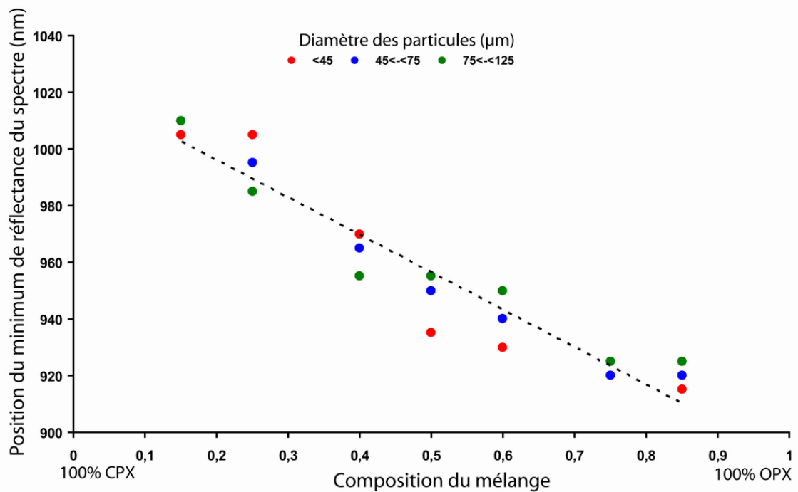
FIG. 4.20 – Position du minimum de réflectance dans le domaine à 1 \mu\text{m} en fonction de la proportion d'orthopyroxène dans le mélange. Les trois couleurs correspondent aux trois tailles de grains étudiées.
