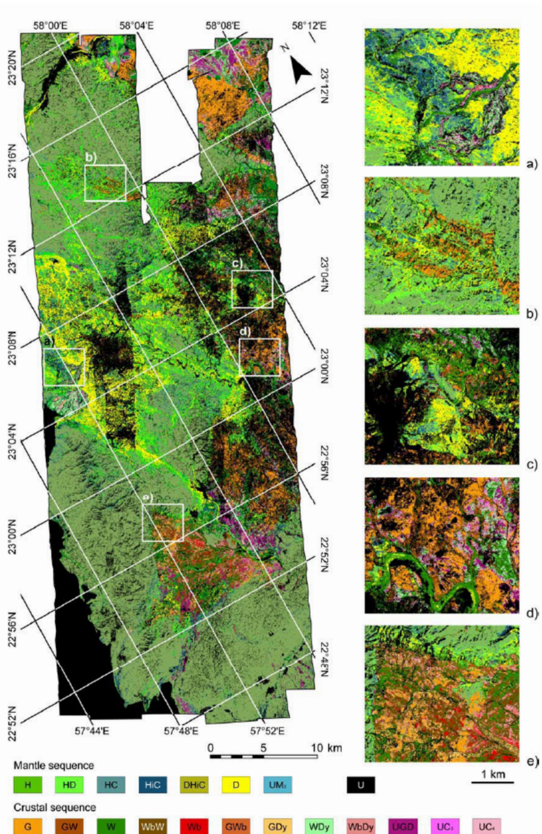
FIG. 2.11 – Carte géologique d'une partie du massif de Sumail créée automatiquement à partir des données hyperspectrales HyMap (extrait de Roy et al. , 2008). H = harzburgite; HD = harzburgite et dunite; HC et HiC = harzburgite et carbonates; DHC = dunite, harzburgite et carbonates interstitiels; D = dunite; UM 3 = roche du manteau non définie; G = gabbro; GW = gabbro et wehrlite; W = wehrlite à plagioclase; WbW = websterite et wehrlite; Wb = websterite; GWb = gabbro et websterite; GDy = gabbro avec dykes; WDy = wehrlite avec dykes; WbDy = websterite avec dykes; UGD = gabbro supérieurs et dykes; UC 3 et UC 4 = roche de la croûte non définie; U = non carté
