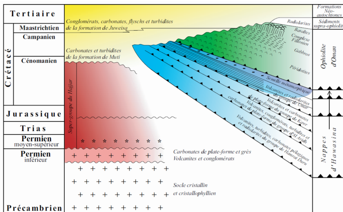
FIG. 2.7 – Schéma simplifié des relations entre les différentes unités structurales et lithologies correspondantes (extrait de Python, 2002, original modifié d'après Searle et Malpas, 1980; Ernewein, 1987; Rabu et al. , 1993)
