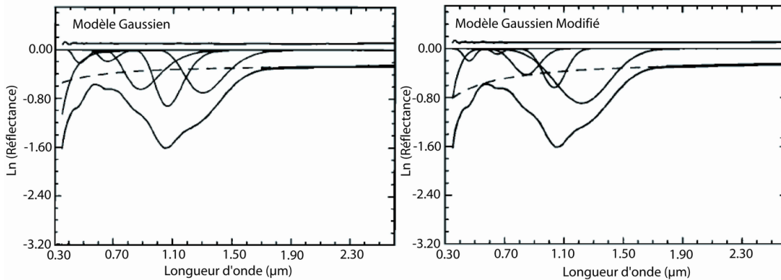
FIG. 3.23 – Différence entre la modélisation effectuée par le Modèle Gaussien classique (à gauche) et le Modèle Gaussien Modifié (à droite). Exemple sur une forstérite, d'après Sunshine et al. (1990).
