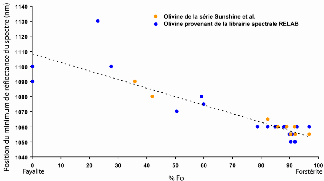
FIG. 4.27 – Position du minimum de réflectance du spectre en fonction de la composition chimique de l'olivine. Les spectres proviennent de la bibliothèque spectrale RELAB, les points oranges étant ceux utilisés par Sunshine et Pieters (1998).
