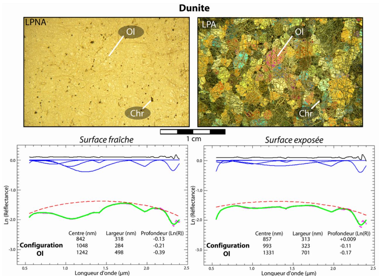
FIG. 7.8 – Dunite, en haut : lame mince en lumière polarisée non analysée (LPNA) et en lumière polarisée analysée (LPA) ; en bas : analyse MGM avec la configuration Ol pour la surface fraîche (à gauche) et la surface exposée (à droite). ( Chr =chromite)
