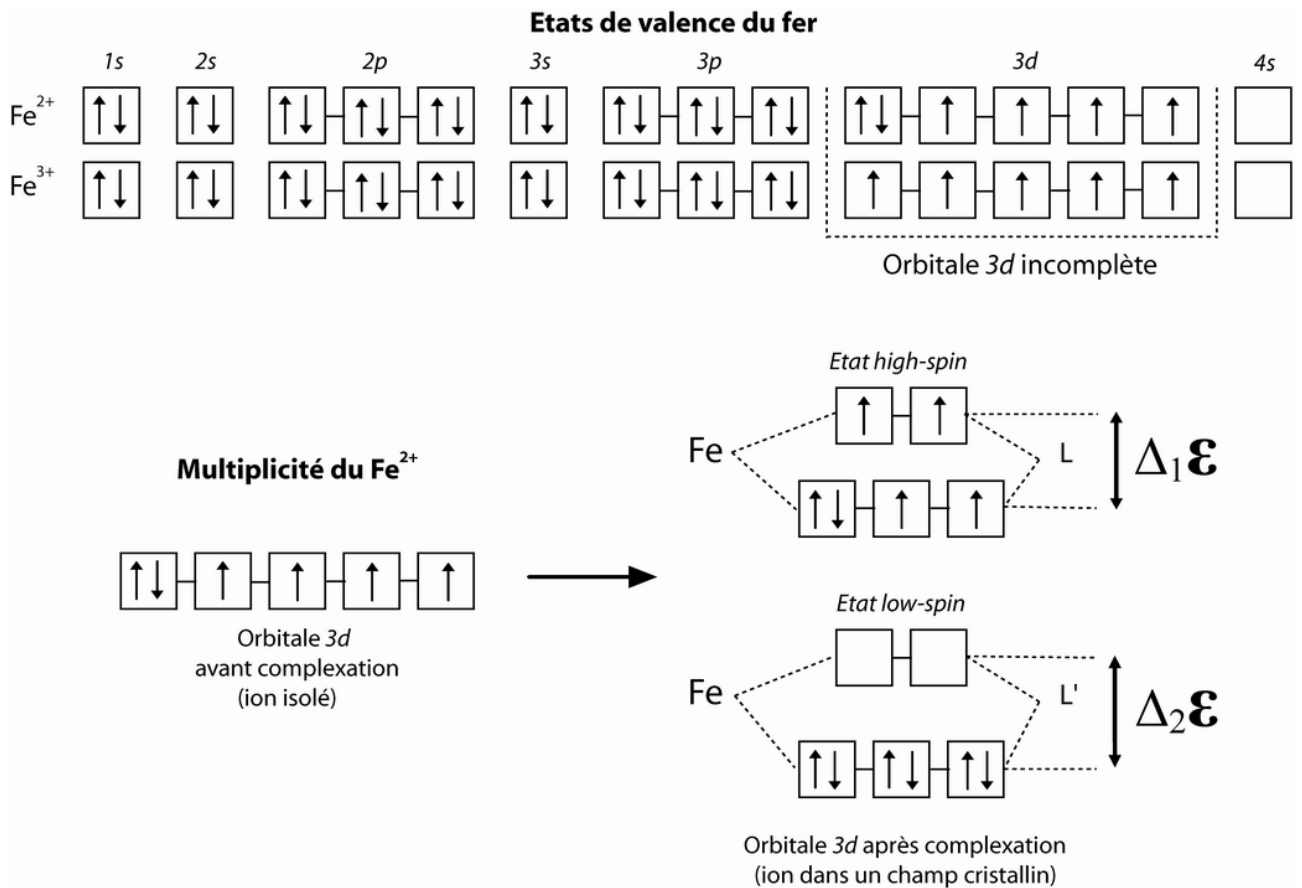
FIG. 3.6 – Évolution de la multiplicité du fer \text{Fe}^{2+} selon la nature du ligand. La complexation avec le ligand L a libérée moins d'énergie que celle avec le ligand L'. \Delta_1 \epsilon est donc une différence d'énergie plus faible que \Delta_2 \epsilon . Dans ce second cas, les électrons restent sur le sous-niveau de plus faible énergie.
