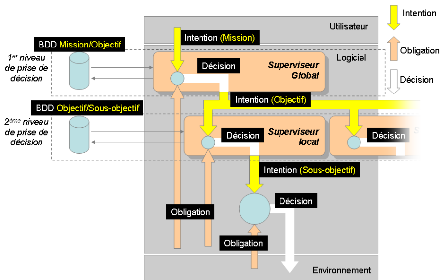
FIG. 6.3 – Deuxième niveau de prise de décision, les superviseurs locaux
