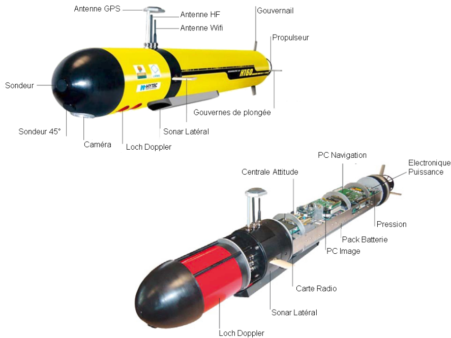
FIG. 8.1 – Véhicule sous-marin autonome Taipan II ou H160
