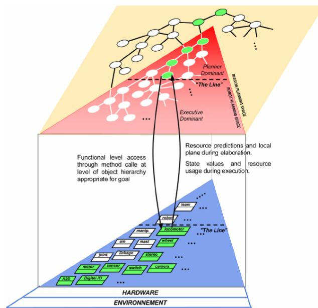
FIG. 2.9 – Modèle d'organisation de l'architecture CLARATy [31]
