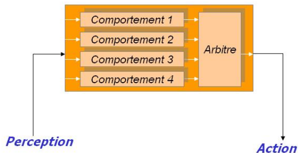
FIG. 2.3 – Architectures réactives arbitrées
