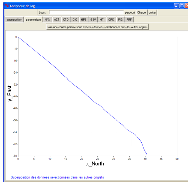
FIG. 11.2 – Trajectoire de l’AUV calculée à partir de l’estimation de déplacement
