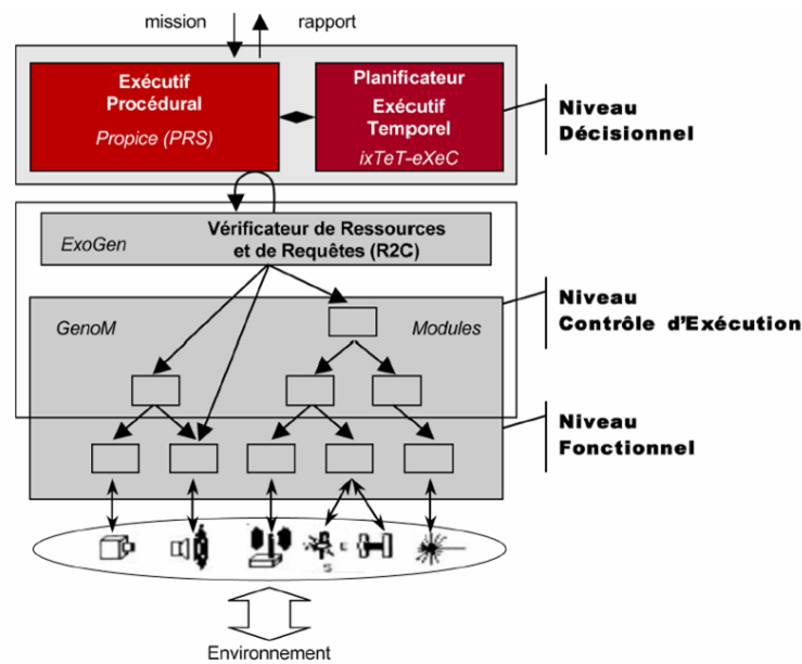
FIG. 2.8 – Modèle d'organisation de l'architecture de contrôle du LAAS [27]
