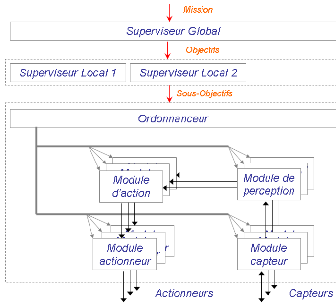
FIG. 6.14 – Architecture logicielle de commande
