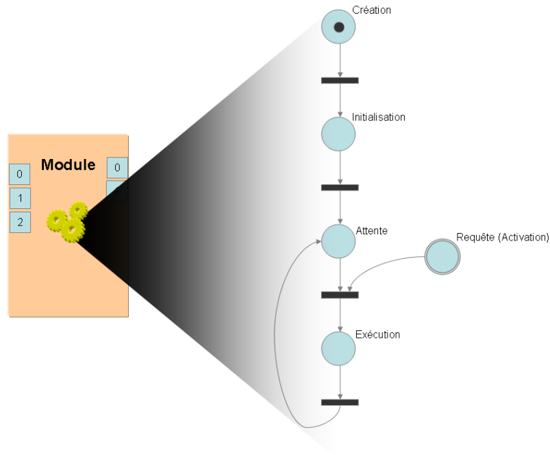
FIG. 5.9 – Modèle simplifié (basé réseau de Petri) d'un module
