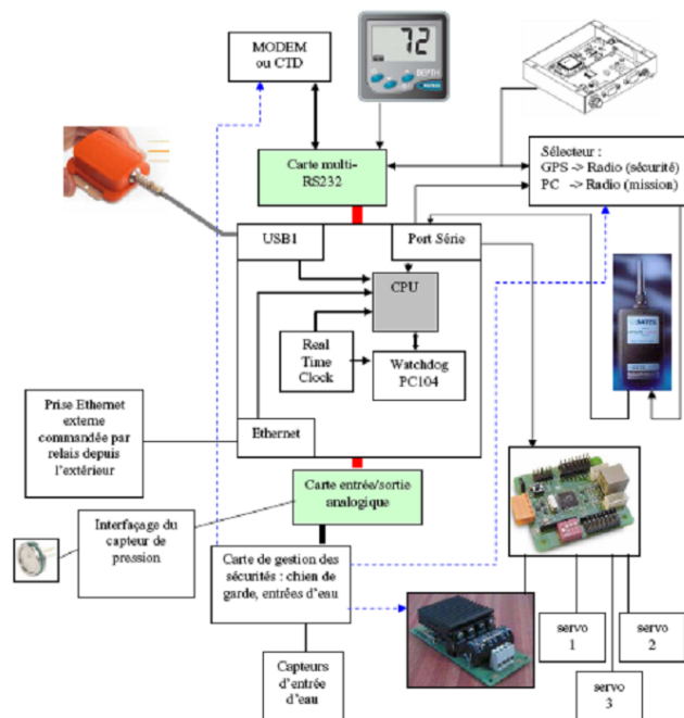
FIG. 8.5 – Architecture matérielle informatique de taipan 300 et connexions avec l'instrumentation
