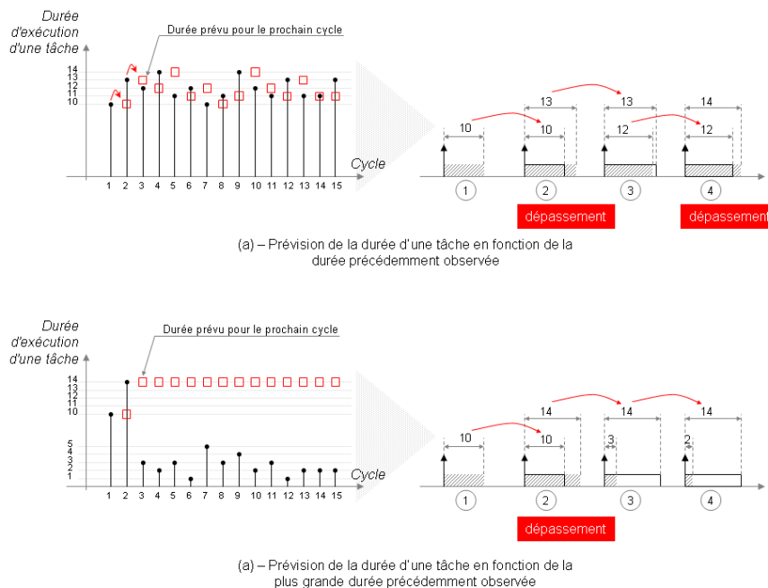
FIG. 7.12 – Prédiction des durées des tâches à chaque cycle
