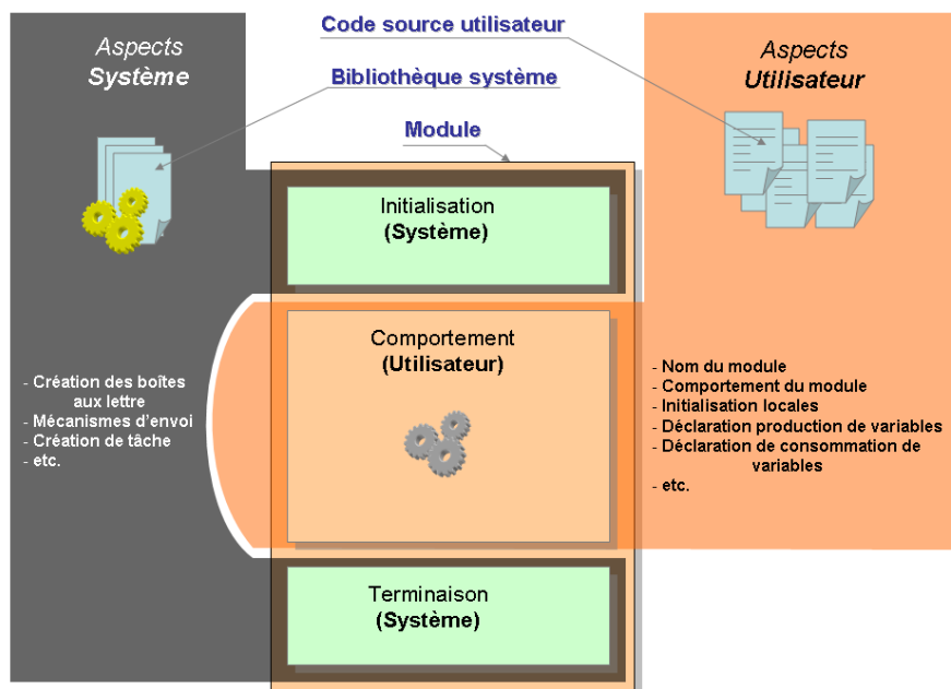
FIG. 9.3 – Structure d'un module
