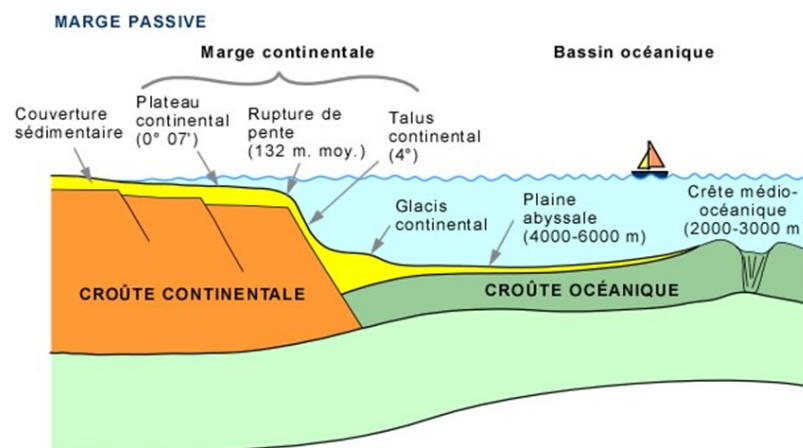
FIG. 1.1 – Coupe de la zone côtière
