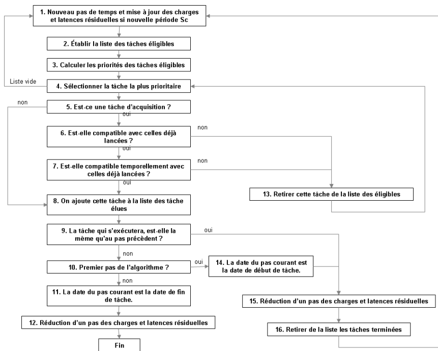
FIG. 10.5 – Organigramme simplifié de l'algorithme de calcul d'ordonnancement
