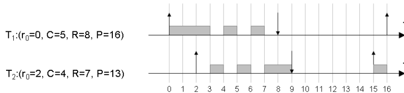
FIG. 3.3 – Ordonnement Least Laxity
