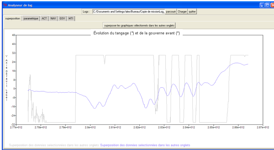
FIG. 11.5 – Evolution du tangage (degrés) et de la gouverne avant (degrés)
