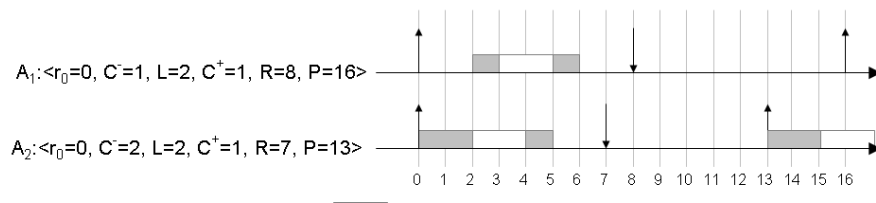
FIG. 7.8 – Ordonnement Earliest Deadline pour les tâches d'acquisition
