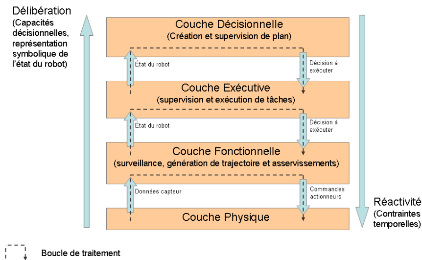
FIG. 2.6 – Modèle d'organisation des architectures délibératives
