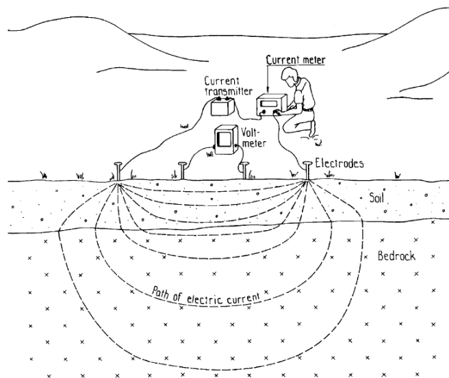
Figure 6 : Principe de la mesure de résistivité électrique DC sur le terrain, représentant la disposition des deux électrodes d'injection et des deux électrodes de mesures [tiré de Dahlin, 2001, d'après Robinson & Coruh, 1988].
