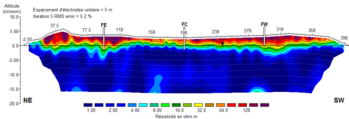
Figure 54 : Section de résistivité inversée avec la contrainte L_2 -normée pour le profil 2 (profil transversal passant par le centre de l'îlot) après troncature des données de résistivités apparentes de profondeur supérieure à 20 m. La topographie est prise en compte dans le calcul inverse et représentée sur la section calculée, avec positionnement des forages (barres verticales blanches) et indication de la surface piézométrique (trait fin noir horizontal).
