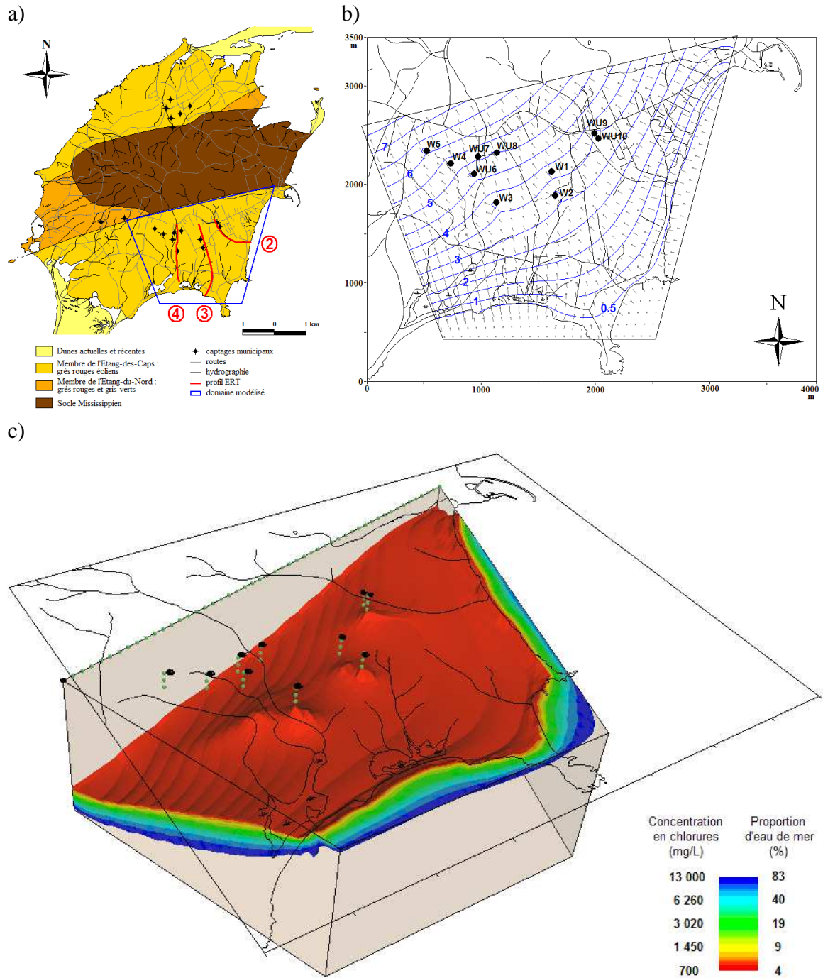
Figure 27 : Résultats du modèle d'écoulement densitaire : a) localisation du domaine modélisé sur l'Île-du-Cap-aux-Meules avec positionnement des captages et des profils ERT (2), (3) et (4) de la Figure 21 ; b) vue en plan de la piézométrie et des vitesses d'écoulement simulées ; c) vue 3D de la zone de transition entre l'eau douce et l'eau salée simulée, montrant les cônes de remontées salines à l'aplomb des captages.
