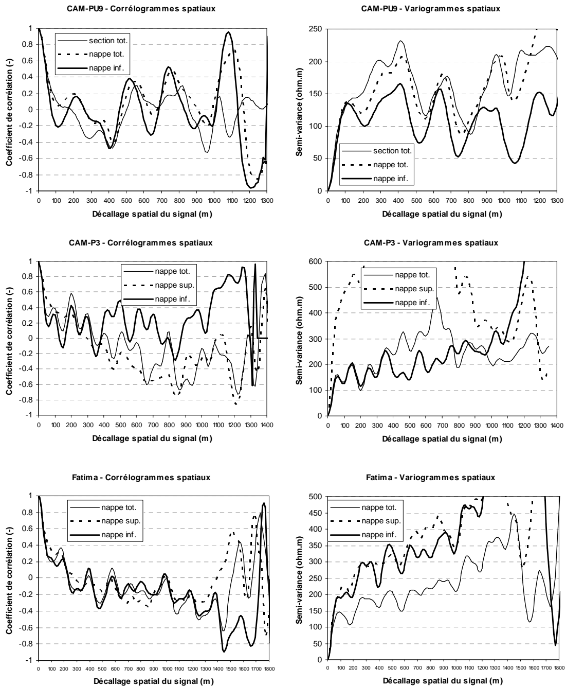
Figure 25 : Auto-correlogrammes et auto-variogrammes des variations de résistivité dans le sens d'écoulement de la nappe, pour les sections montrant les dérives de cônes de remontées salines (Figure 23), et pour 3 cas d'intégration verticale des résistivités inversées.
