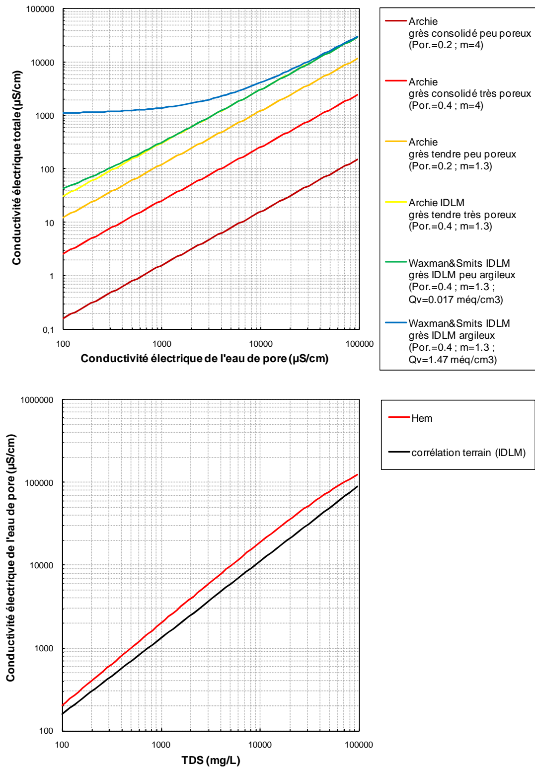
Figure 35 : Graphique du haut : comparaison des modèles pétrophysiques d'Archie [1942] correspondant à différents matériaux géologiques allant de grès consolidés à faible porosité aux grès mal consolidés et très poreux des Îles-de-la-Madeleine (IDLM), et effet de la teneur en argile sur les grès des IDLM, prise en compte par le modèle de Waxman & Smits [1968] ; Graphique du bas : comparaison du modèle physico-chimique empirique de Hem [1985] avec la corrélation puissance établie d'après les données hydrochimiques aux IDLM.
