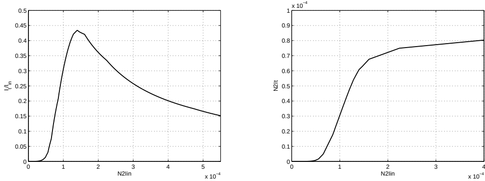
(a) Fonction de transfert non-linéaire par rapport à l'intensité en entrée : I_t/I_{in} = f(I_{in}) (b) Intensité transmise en fonction de l'intensité en entrée : I_t = f(I_{in}) .
