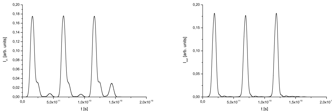
(c) ( b_4 , figure 4.6) = Port "transmis" du premier étage.
