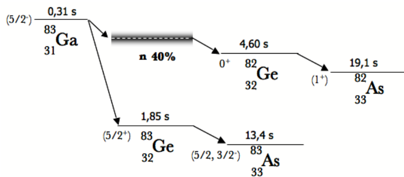
FIGURE 3.14: Schéma de la décroissance \beta^- et \beta^-n du ^{83}_{31}\text{Ga}_{52} . Les valeurs des périodes et des rapport d'embranchements sont tirées de [Bag].
