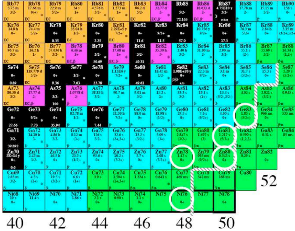
FIGURE 1.1: Agrandissement de la charte des noyaux autour du ^{78}_{28}\text{Ni}_{50} [Bag]. La ligne en pointillée représente la limite expérimentale de la connaissance sur la structure dans la région. Les noyaux entourés sont les plus exotiques étudiés dans la région.
