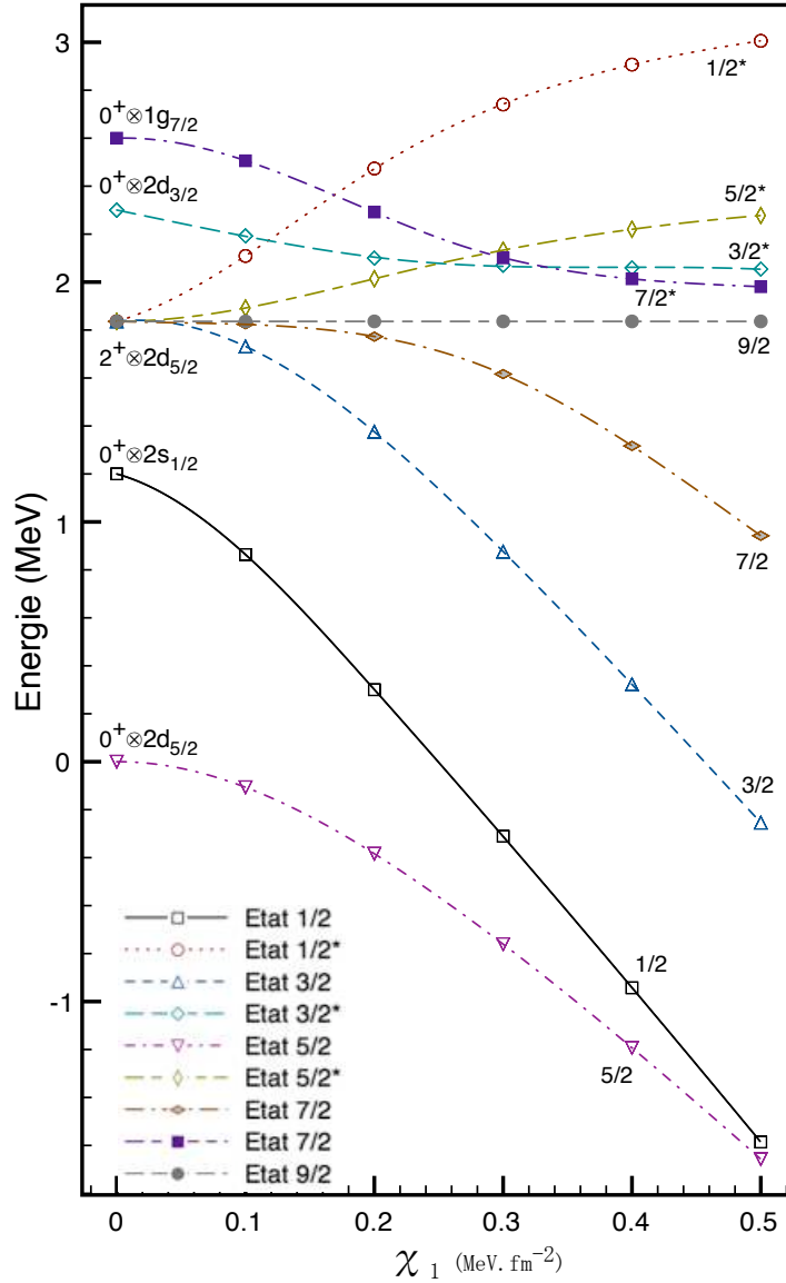
FIGURE 5.2: Variation des valeurs propres en fonction de \chi_1 avec \xi = 0 \text{ MeV} et \chi_2 = 0 \text{ MeV} \cdot \text{fm}^{-2} pour le ^{89}\text{Sr} .
