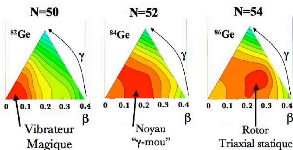
FIGURE 4.12: Cartographie des potentiels de {}^{82-84-86}\text{Ge} , en fonction de la déformation \beta pour 0 \leq \gamma \leq 60 . Chaque ligne correspond à une équipotentielle distante de 1 MeV ; les plus petites valeurs de potentiel sont en gris clair et augmentent jusqu’au gris foncé. Le nom du noyau est indiqué au dessus du potentiel.
