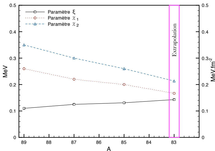
FIGURE 5.14: Courbe de l'évolution des paramètres \xi , \chi_1 , et \chi_2 . Sur cette courbe, les points correspondants à {}^{83}_{32}\text{Ge}_{51} ont été extrapolés à partir des valeurs obtenues pour les autres isotones.
