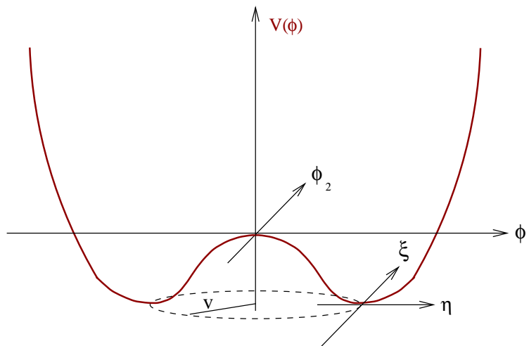
FIG. 1.2 – Potentiel de Higgs dans le cas d'une théorie de jauge reposant sur le groupe U(1) .
