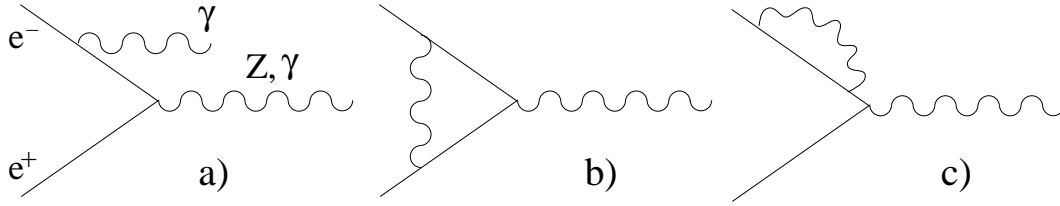
FIG. 1.9 – Diagrammes de Feynman correspondant aux radiations dans l'état initial d'un photon réel (a), ou d'un photon virtuel (b et c).
