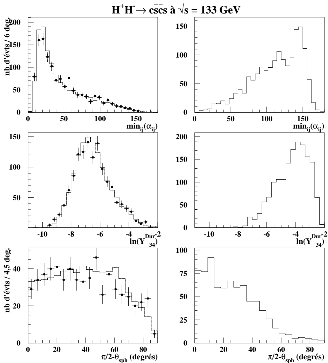
FIG. 4.19 – Distributions des variables composant la fonction discriminante multidimensionnelle F_{cscs} pour les processus standards simulés (histogrammes) superposés aux événements réels (points), à gauche, et pour le signal constitué de 1600 événements engendrés avec m_{H^\pm} = 44 et 46 GeV/ c^2 , à droite. Tous les événements utilisés vérifient le critère de présélection hadronique.
