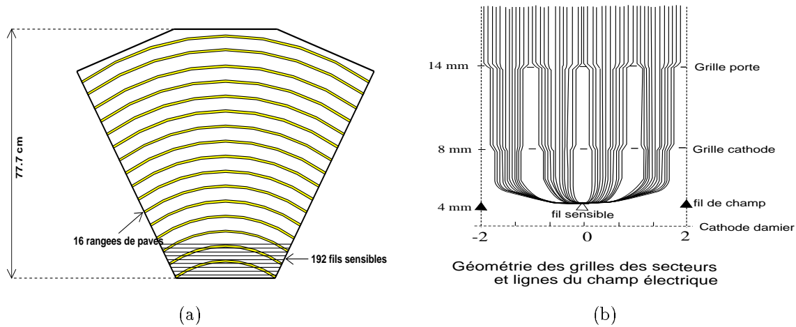
FIG. 2.11 – (a) Vue de face schématique de l'un des six secteurs d'un côté de la TPC . Une partie seulement des fils sensibles est représentée.
