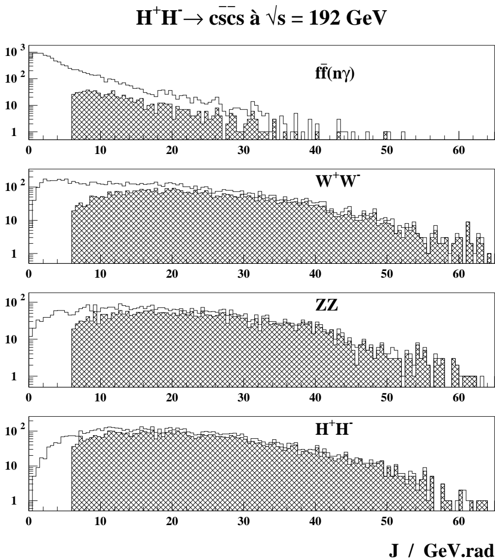
FIG. 8.5 – Distribution de la variable \mathcal{J}_{c\bar{c}s\bar{s}} , produit de l'énergie du jet le moins énergétique et de l'angle minimal entre deux jets quelconques, une fois les particules de l'événement regroupées en quatre jets à l'aide de l'algorithme de JADE. Les commentaires de la figure 8.3 sont valables ici aussi.
