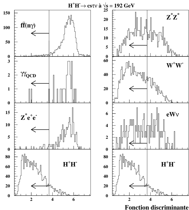
FIG. 8.15 – Distributions de la fonction discriminante multidimensionnelle F_{c\tau\nu} , obtenues à partir d'un lot d'événements du signal engendrés avec plusieurs masses et à partir des lots d'événements des processus standards. Tous les événements utilisés vérifient les critères C1 à C4.
