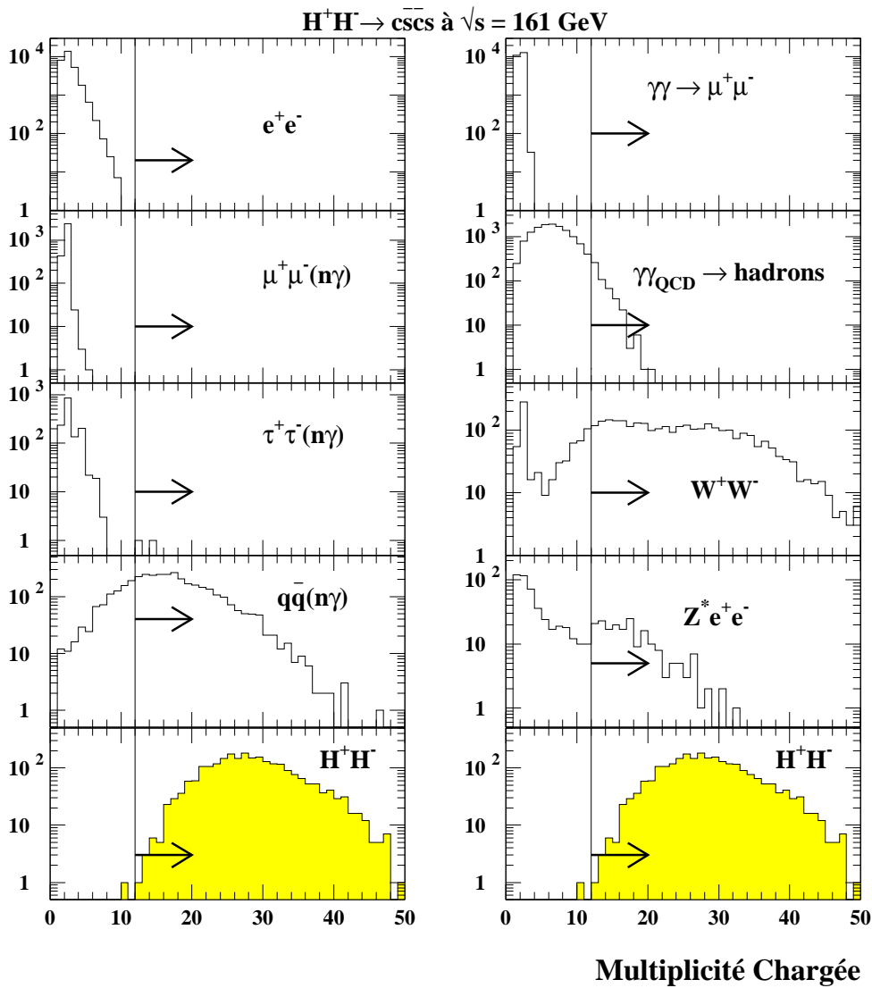
FIG. 4.14 – Distribution du nombre de particules chargées, pour quelques processus de bruit de fond et le signal. Aucune sélection n'est appliquée sur les événements utilisés. Les flèches indiquent les valeurs autorisées par la présélection hadronique.
