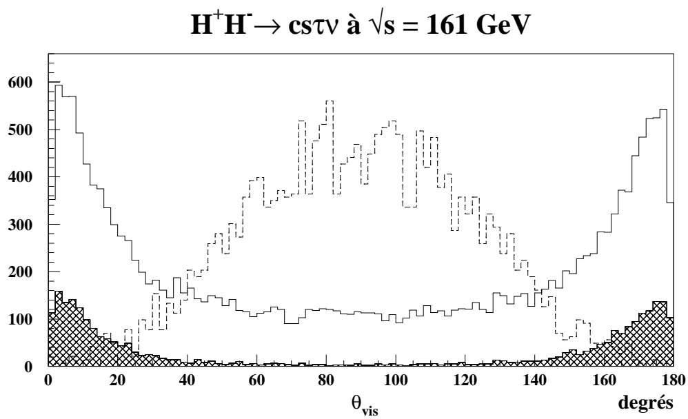
FIG. 5.6 – Distribution de l'angle polaire du vecteur quantité de mouvement totale. L'histogramme au trait continu est obtenu avec les événements du processus e^+e^- \rightarrow q\bar{q}(n\gamma) qui vérifient les critères de la présélection hadronique. L'histogramme hachuré est obtenu avec les événements du processus e^+e^- \rightarrow q\bar{q}(n\gamma) sélectionnés avec les critères C1 à C4. L'histogramme au trait discontinu est obtenu avec des événements du signal, engendrés avec plusieurs valeurs de m_{H^\pm} , et sélectionnés avec les critères C1 à C4.
