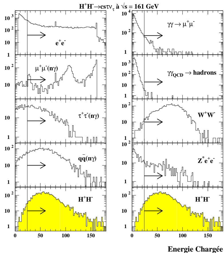
FIG. 5.14 – Energie des particules chargées des événements de quelques processus de bruit de fond et du signal. Aucune sélection n'est appliquée sur les événements utilisés. Les flèches indiquent la présélection hadronique.
