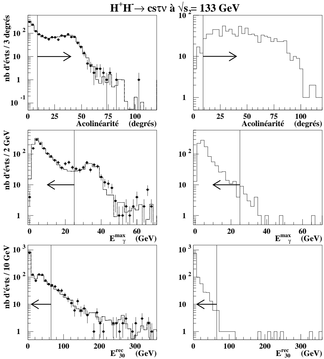
FIG. 5.18 – Distributions de l'acolinéarité, des variables E_{\gamma}^{\max} et E_{30}^{\text{rec}} , pour les processus standards simulés (histogrammes) superposés aux événements réels (points), à gauche, et pour le signal de référence ( m_{H^{\pm}} = 45 GeV/c 2 ), à droite. Tous les événements utilisés vérifient le critère de présélection hadronique. Les coupures appliquées sont indiquées par les flèches.
