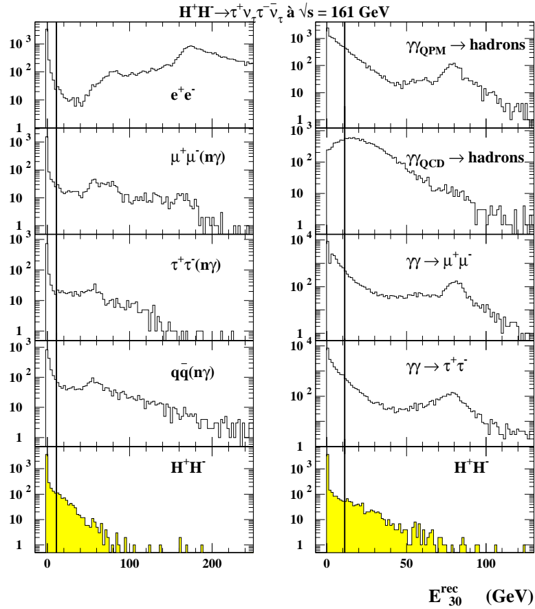
FIG. 6.10 – Energie visible à l'avant E_{30}^{rec} , pour quelques processus de bruit de fond et pour le signal. Aucune sélection n'est appliquée sur les événements utilisés. Les lignes indiquent la valeur maximale autorisée par la présélection leptonique.
