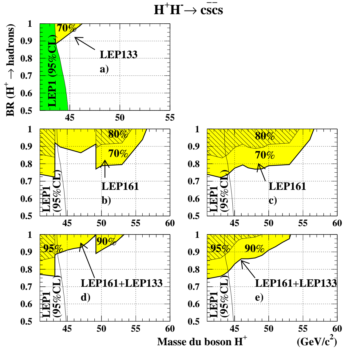
FIG. 7.1 – Régions du plan [m_{H^\pm}, Br(H^+ \rightarrow \text{hadrons})] exclues avec différents niveau de confiance par les analyses des données de LEP133 et de LEP161, pour la topologie hadronique, utilisées séparément ou de manière combinée. ( cf texte pour une description plus précise)
