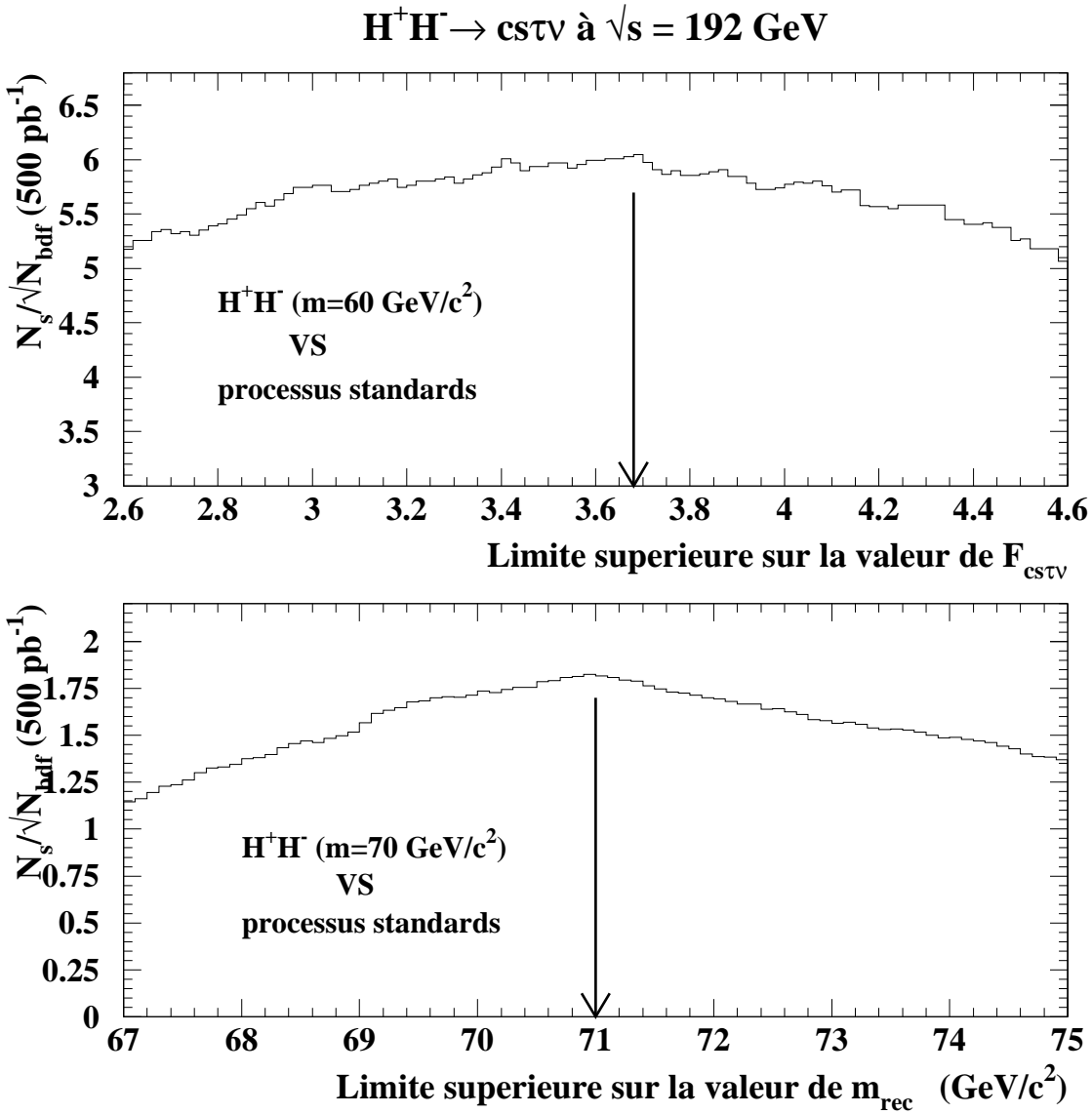
FIG. 8.17 – Rapport N_s/\sqrt{N_{bdf}} , pour une luminosité intégrée de 500 \text{ pb}^{-1} , en fonction de la coupure sur la variable F_{cst\nu} (en haut), et en fonction de la limite supérieure imposée à la masse reconstruite (en bas) dans le cas où je teste une masse du boson H^\pm égale à 70 \text{ GeV}/c^2 .
