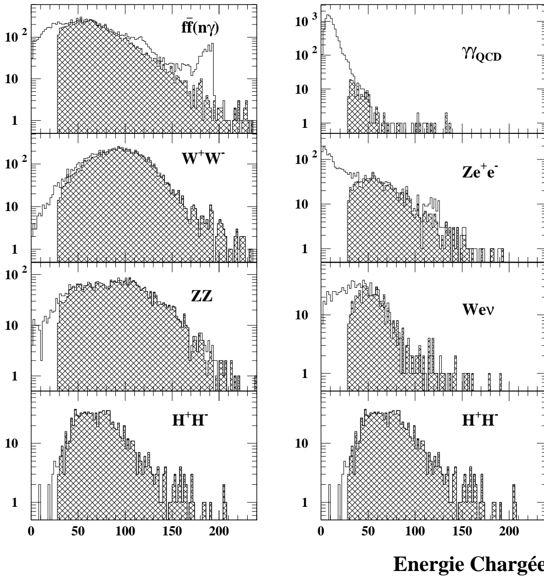
FIG. 8.12 – Distribution de l'énergie des particules chargées. Les histogrammes vides sont obtenus sans aucune sélection sur les événements ; les histogrammes hachurés sont obtenus à partir des événements sélectionnés à l'aide du critère C1. Pour le signal, les événements ont été engendrés avec une masse de 60 \text{ GeV}/c^2 .
