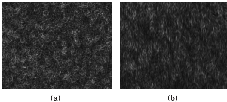
Figure II.8 : Images du speckle créé par un échantillon lambertien métallique observé avec deux différents angles de diffusion. Pour un angle de diffusion de 20°, le speckle a une taille de 42,3 \mu\text{m} (a) et pour un angle de diffusion de 65°, le speckle a une taille de 105,3 \mu\text{m} (b).
