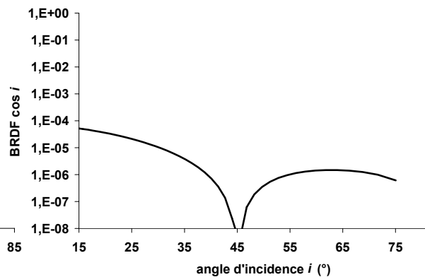
Figure 154 : Indiatrice théorique d'une impureté de dimensions r = 848 nm et h = 100 nm
