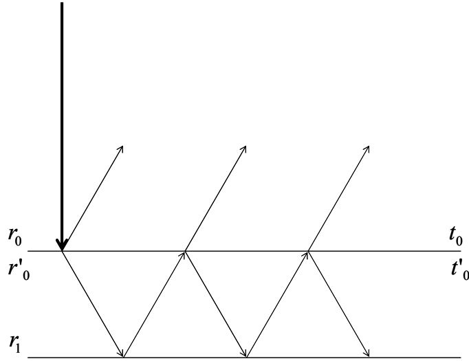
Figure 38 : Réflexions multiples à l'intérieur du dioptre
