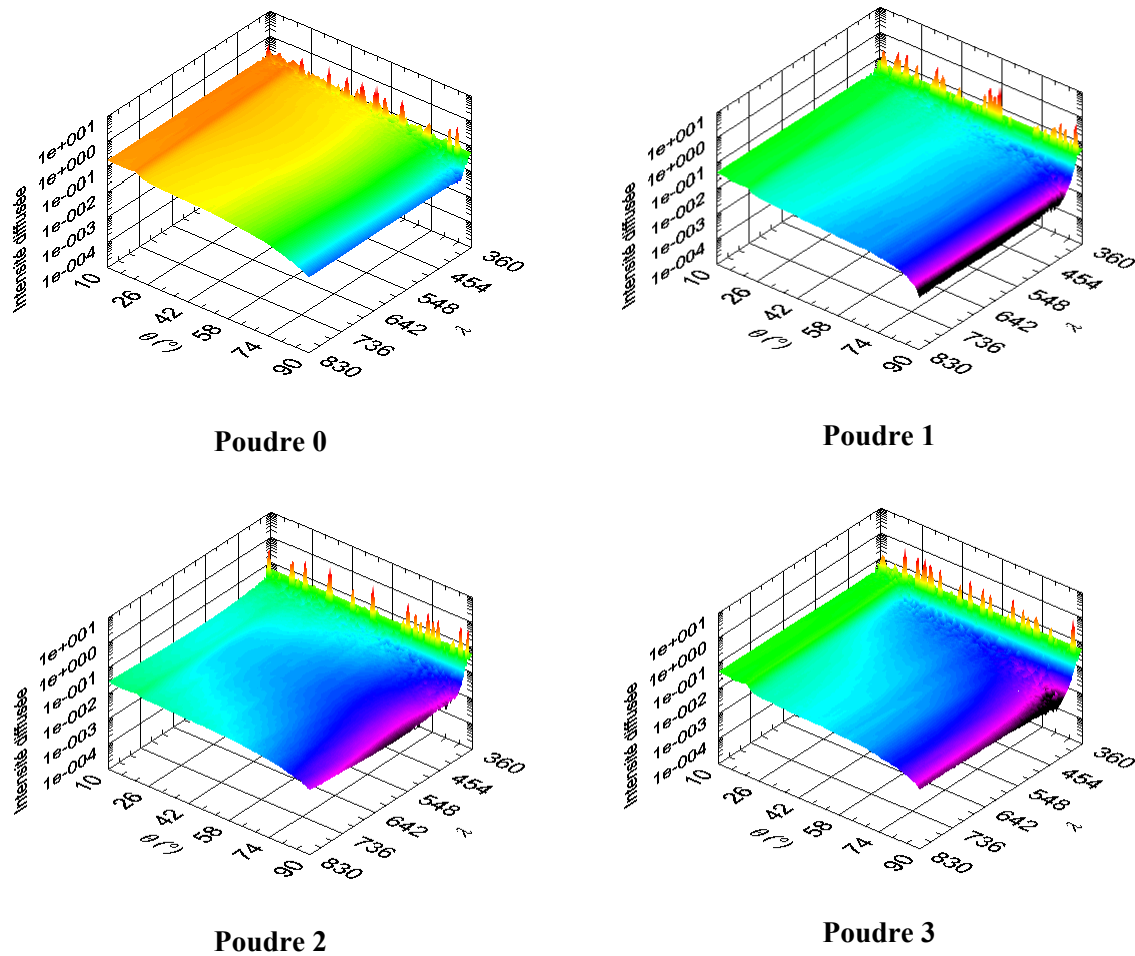
Figure 180 : Indicatrices de diffusion spectrales et angulaires des poudres présentées Figure 179
