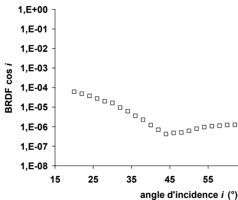
Figure 153 : Indiatrice mesurée pour une impureté
