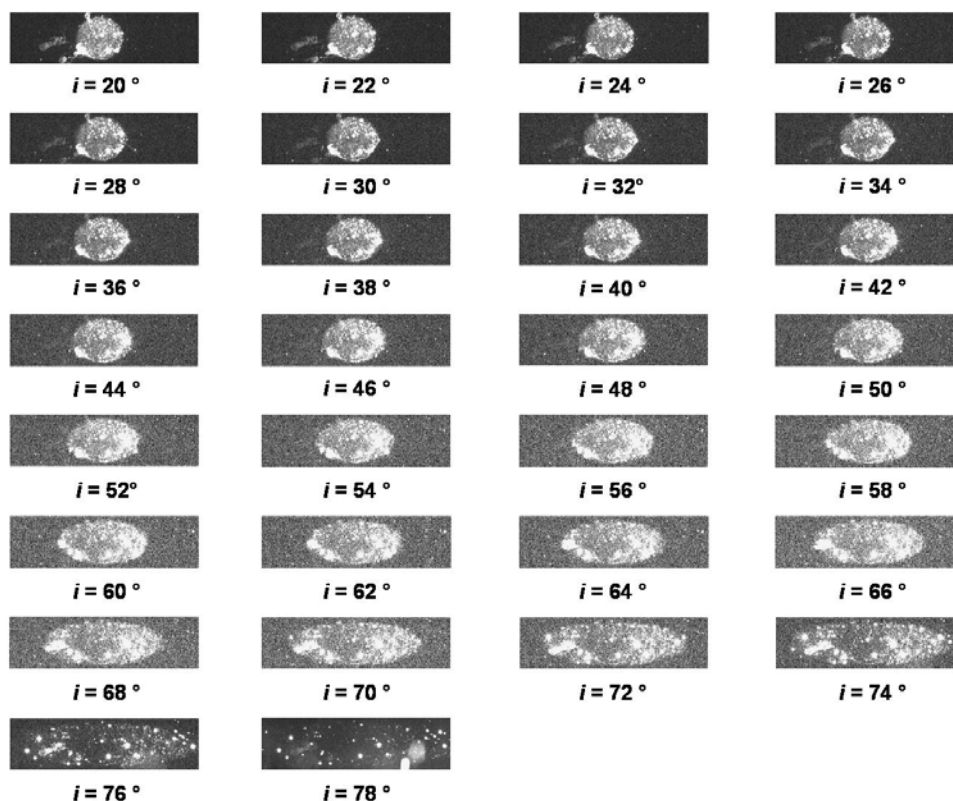
Figure 141 : Images obtenues lors de la mesure d'un verre noir (temps d'intégration : 200 ms)
