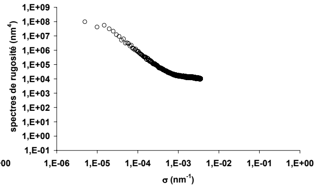
Figure 71 : Spectre de rugosité de la face 1
