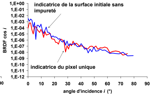
Figure 112 : Indicatrices de diffusion du pixel (6-6) et de la surface initiale (sans impureté) (même pas angulaire)
