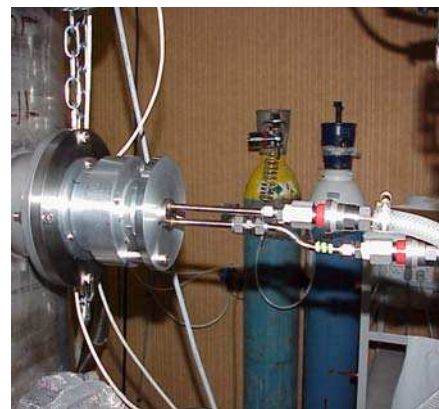
Figure 162 : Porte cibles et système de refroidissement
