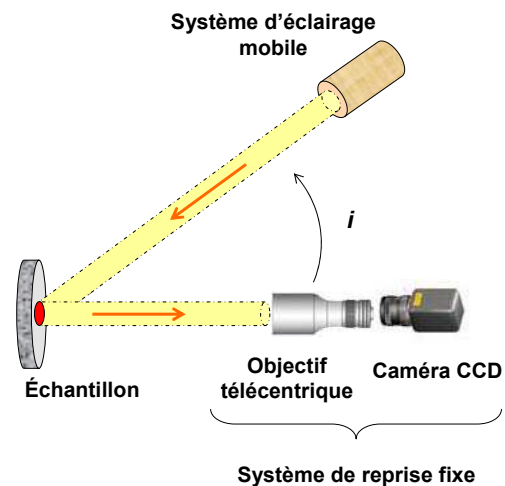
Figure 86 : Schéma de principe du montage proposé
