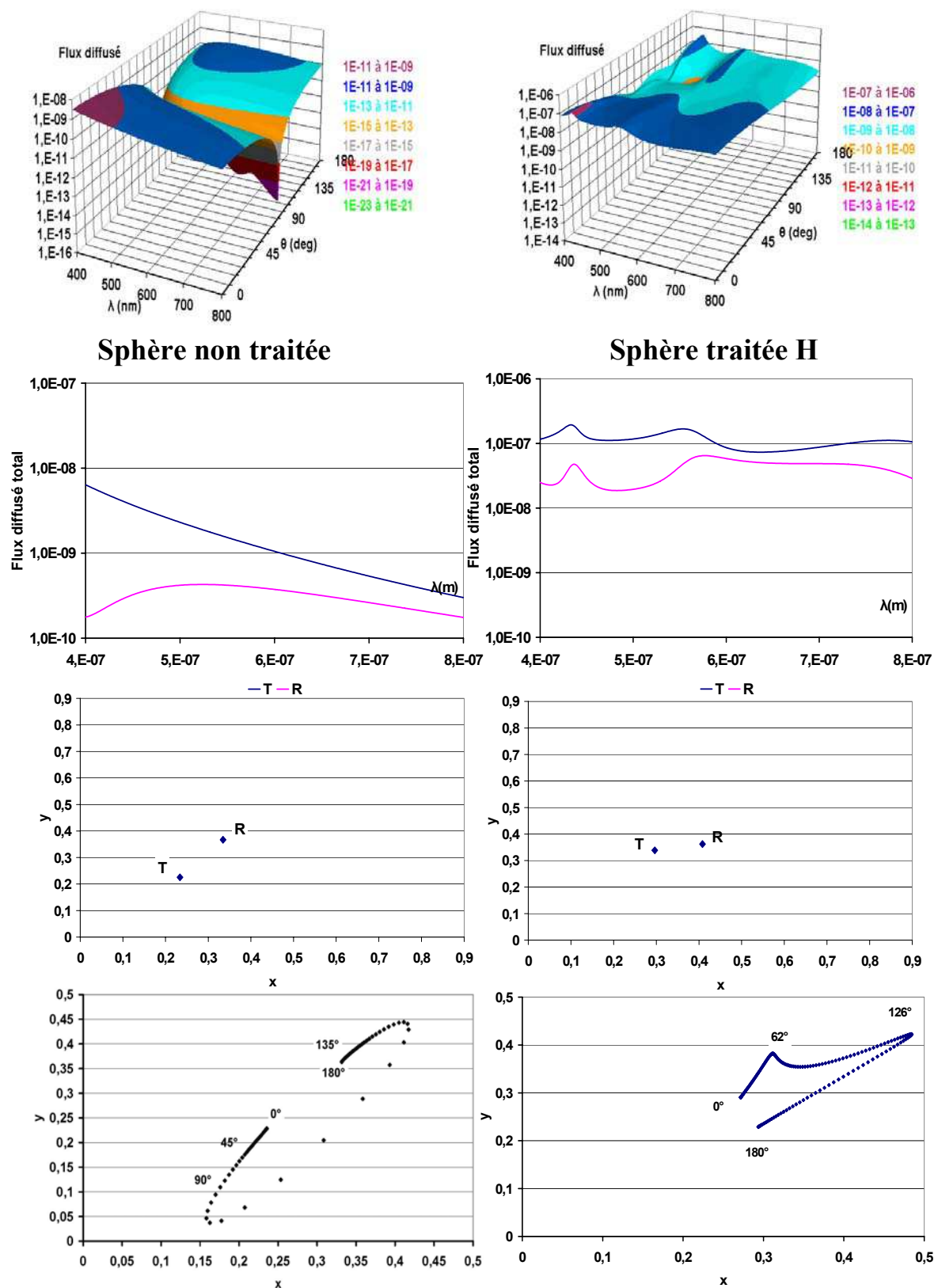
Figure 158 : Influence du dépôt d'une couche haut indice (50 nm) sur une sphère de silice de diamètre 100 \text{ nm}^{24}
