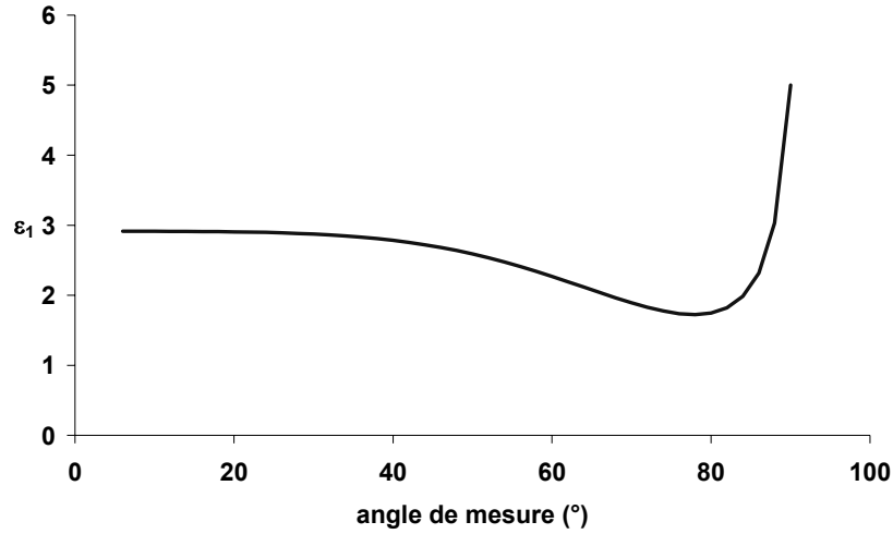
Figure 44 : Évolution angulaire du coefficient \varepsilon_1 en fonction de l'angle
