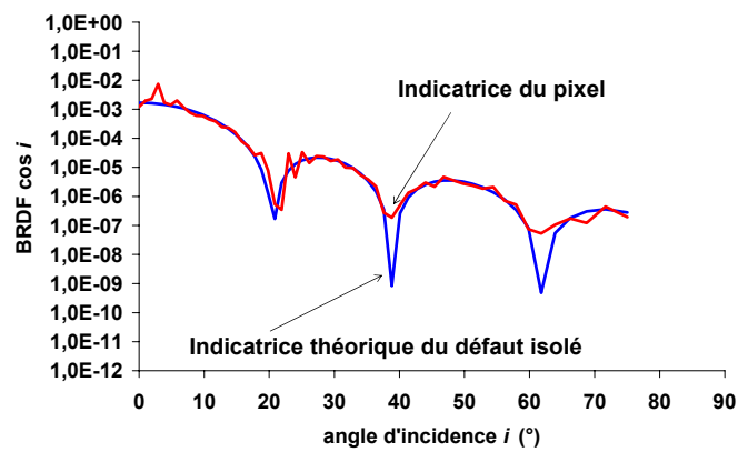
Figure 116 : Indiatrice de diffusion du pixel (4-8) et indiatrice théorique du défaut isolé
