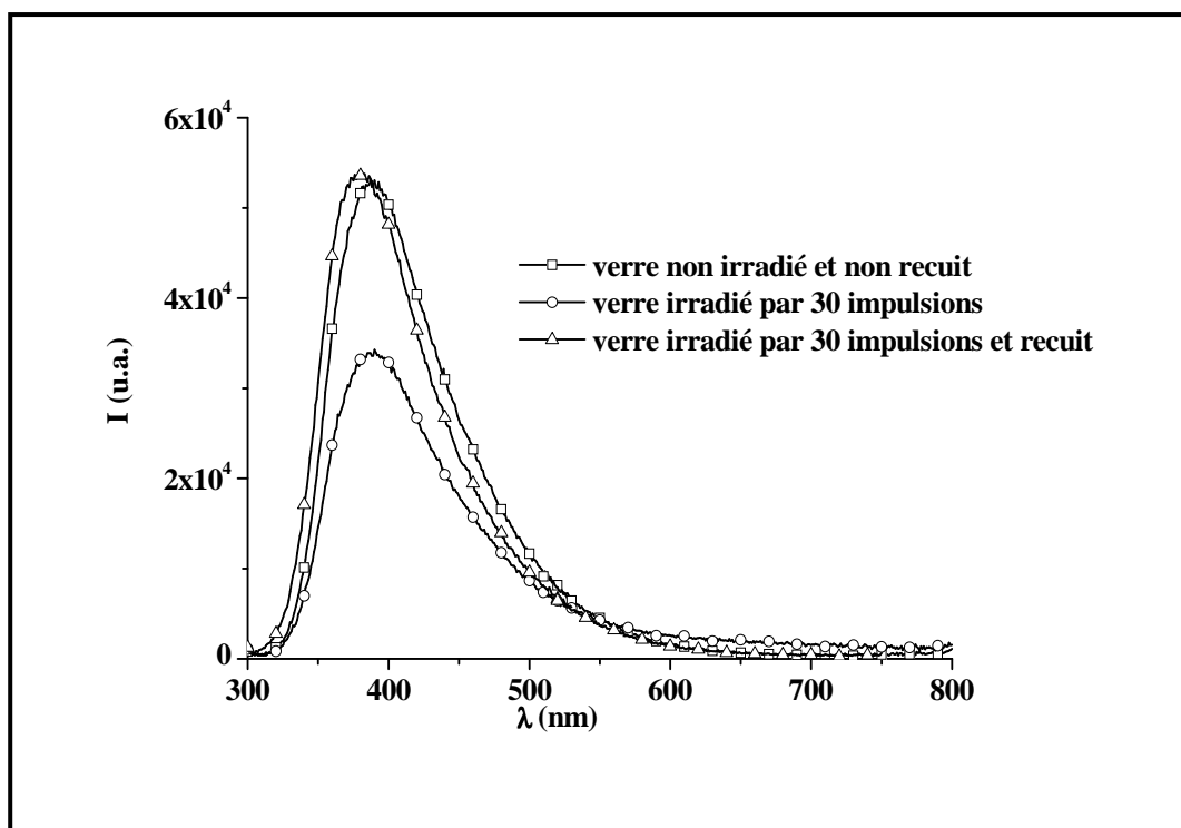
Figure IV.C11 : Spectres d'émission du verre de composition \text{Na}_{0,25}\text{Ag}_{0,75}\text{La}(\text{PO}_3)_4 , non irradié, irradié et irradié recuit, \lambda_{\text{exc.}} = 280 nm à T = 300 K. et \text{Na}_{0,9}\text{Ag}_{0,1}\text{La}(\text{PO}_3)_4
