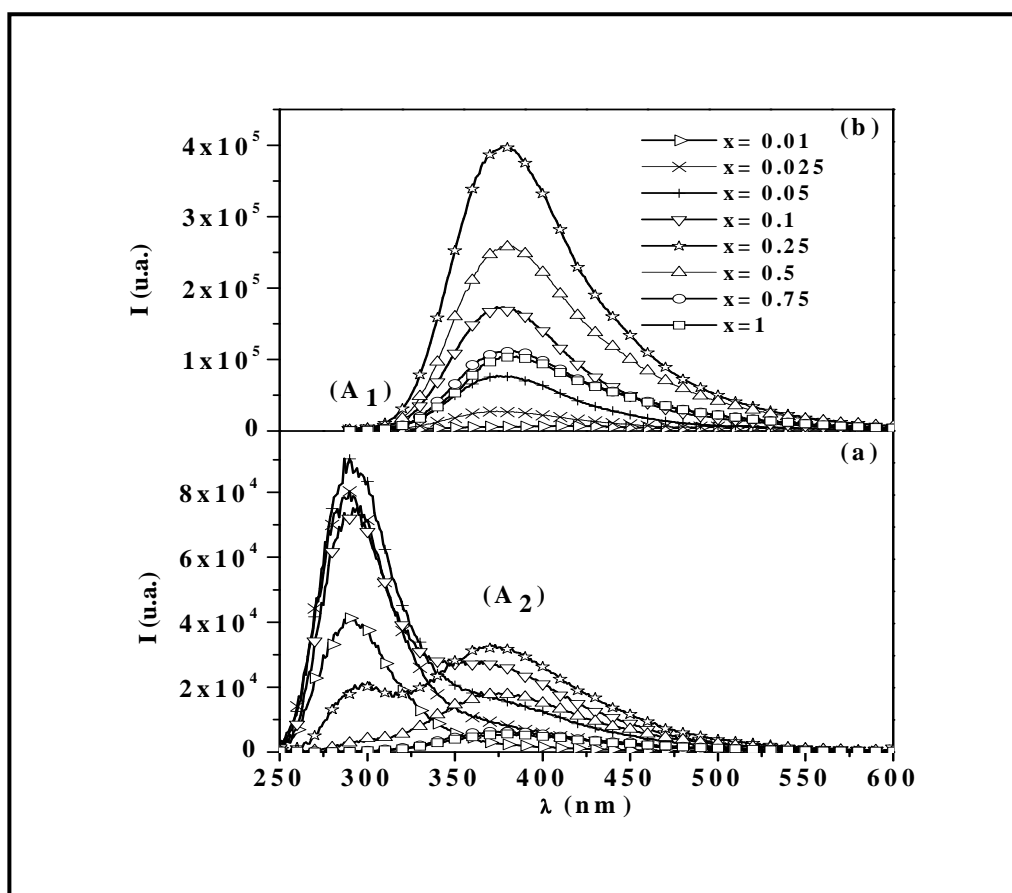
Figure IV-A12 : Evolutions des deux émissions ( A_1 ) et ( A_2 ) dans \text{Na}_{1-x}\text{Ag}_x\text{La}(\text{PO}_3)_4 en fonction du taux en argent, \lambda_{\text{exc.}} = 230 \text{ nm} (a), \lambda_{\text{exc.}} = 270 \text{ nm} (b)
