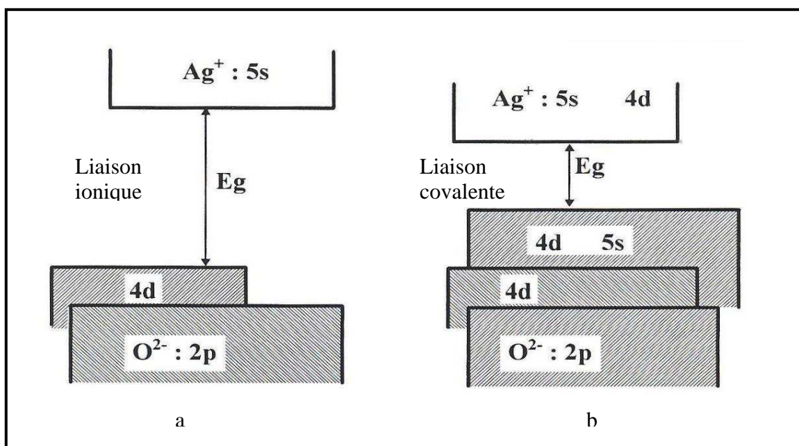
Figure I.16 : Diagrammes d'énergie schématisés pour les oxydes à base d'argent (63).
