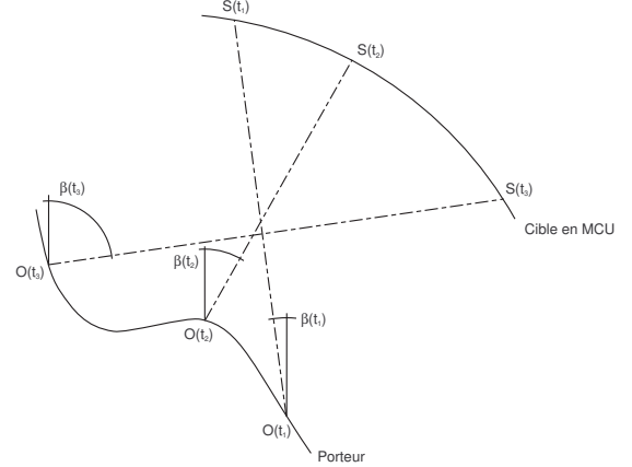
FIG. 2.2 – Cible en MCU
