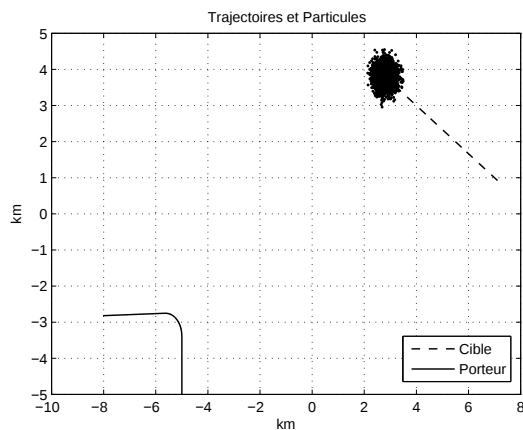
FIG. 14.3 – Cible en MRU, initialisation gaussienne centrée en S(0)
