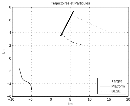
FIG. 14.8 – Cible en MRU, initialisation uniforme sur l'axe (S(0), O(0))
