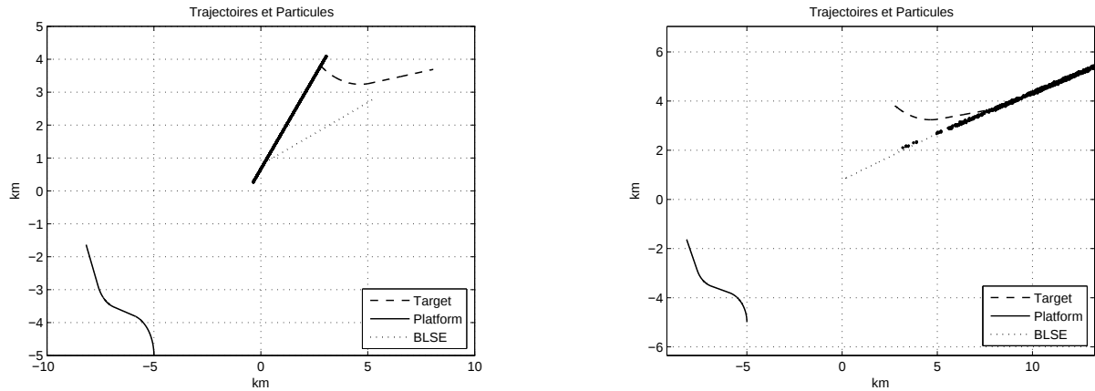
FIG. 14.10 – Cible en MRU, initialisation uniforme sur l'axe (S(0), O(0))
