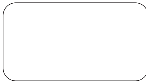
FIG. 2.5 – Trajectoire en hippodrome
