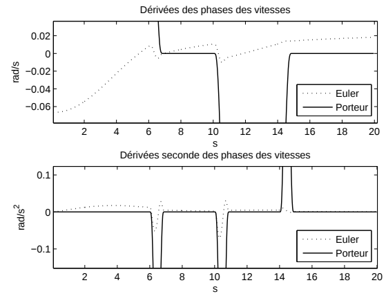
FIG. 7.16 – Dérivées première et seconde des phases des vitesses
