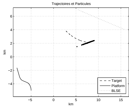
FIG. 14.7 – Cible en MRU, initialisation gaussienne centrée en S(0)
