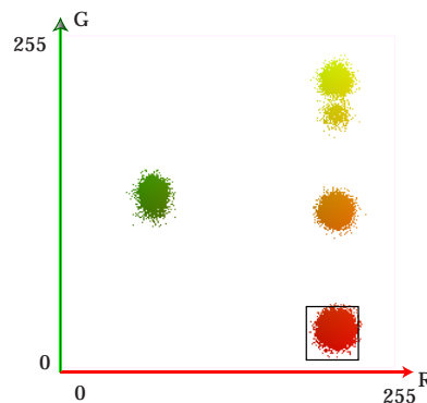
(b) Domaine-couleur \underline{D}(\text{rouge}, [41, 41, 1]^T) du plan couleur (R, G) .
