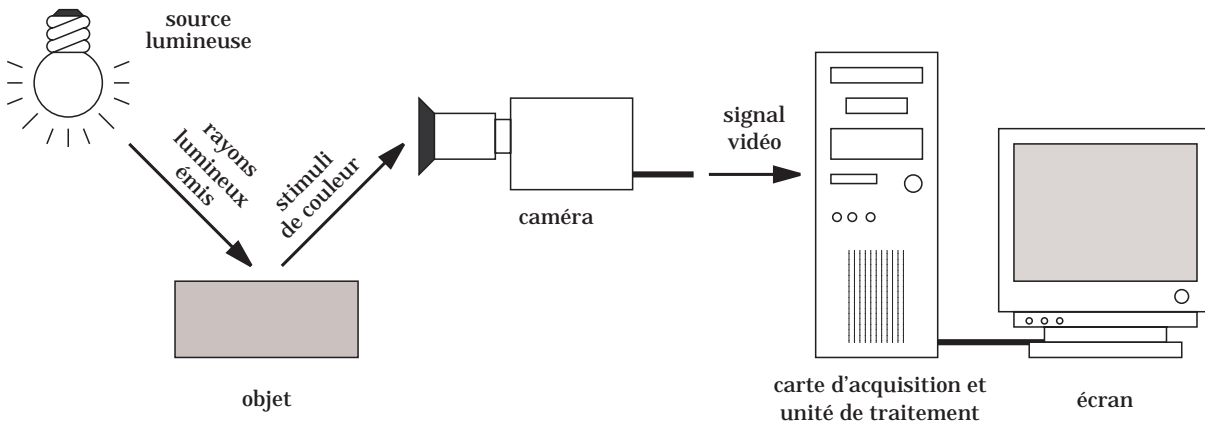
FIG. 1.7 – Vision artificielle.
