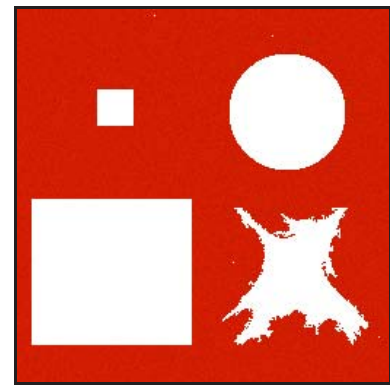
(c) Pixels de l'image de la figure 3.6(a) qui appartiennent au sous-ensemble-couleur S(\text{rouge}, [41, 41, 1]^T) . Les pixels étiquetés en blanc n'appartiennent pas à S(\text{rouge}, [41, 41, 1]^T) .
