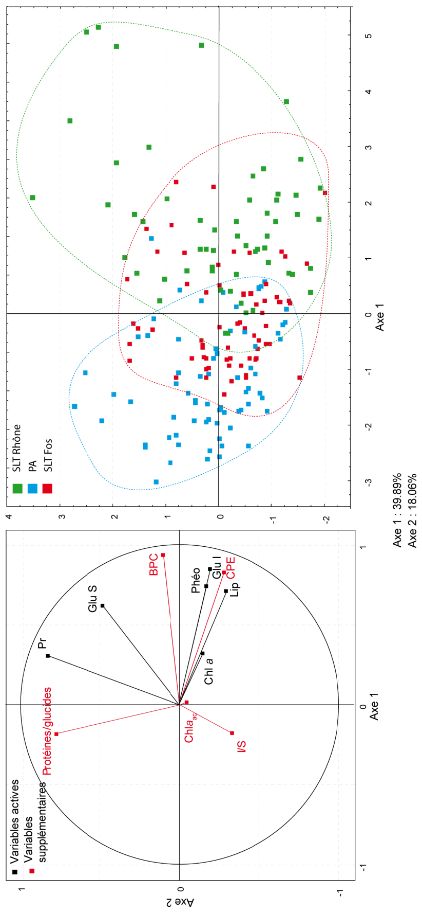
Figure III 22 : ACP normée réalisée avec 6 variables actives (Pr, Glu, Glu S , Lip, Chl a , Phéo) et 5 variables supplémentaires : ( \frac{I}{S} , Pr, Glu, Chl ac , BPC et CPE). N = 198 : SLT Fos, PA et SLT Rhône – 2 centimètres superficiels.
