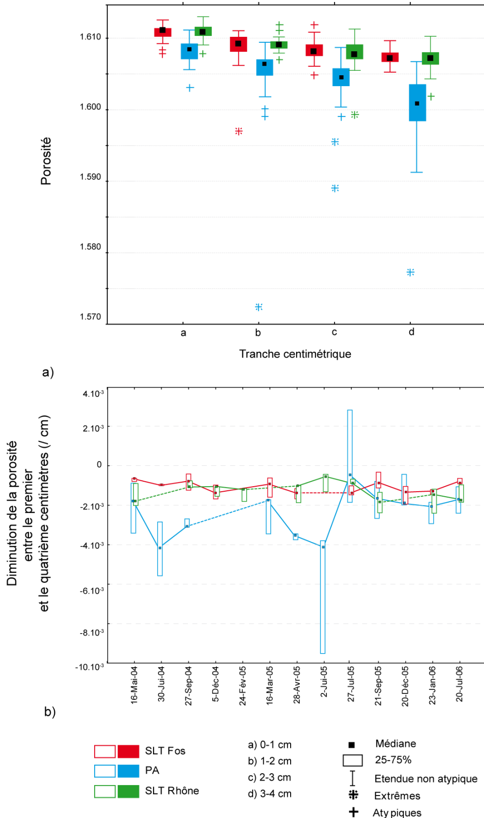
Figure III 11 : Distribution de la porosité totale des sédiments à SLT Fos, PA et SLT Rhône (a) en fonction de la profondeur sous l'interface eau-sédiment et Variation au cours du temps de la pente de diminution de la porosité dans la couche de sédiment (/ cm) (b). Période couverte : mars 2004 à juillet 2006.
