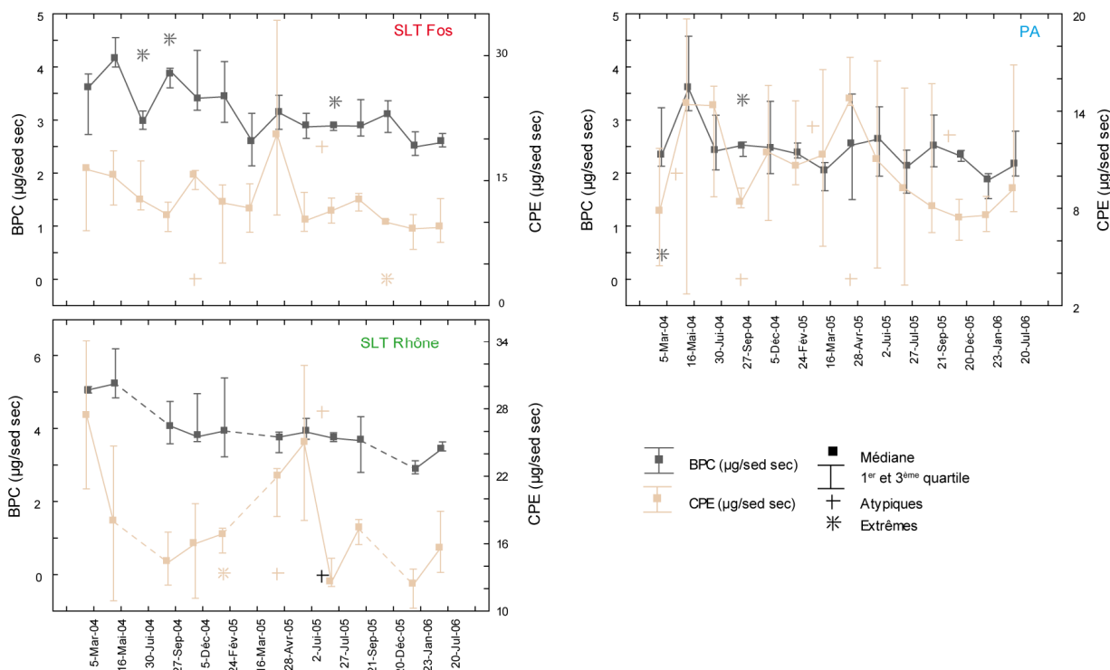
Figure III 20 : Comparaison des variations temporelles des teneurs en BPC ( \mu\text{g/g sed sec} ) et CPE ( \mu\text{g/g sed. sec} ) à SLT Fos, PA et SLT Rhône entre mars 2004 et juillet 2006.
