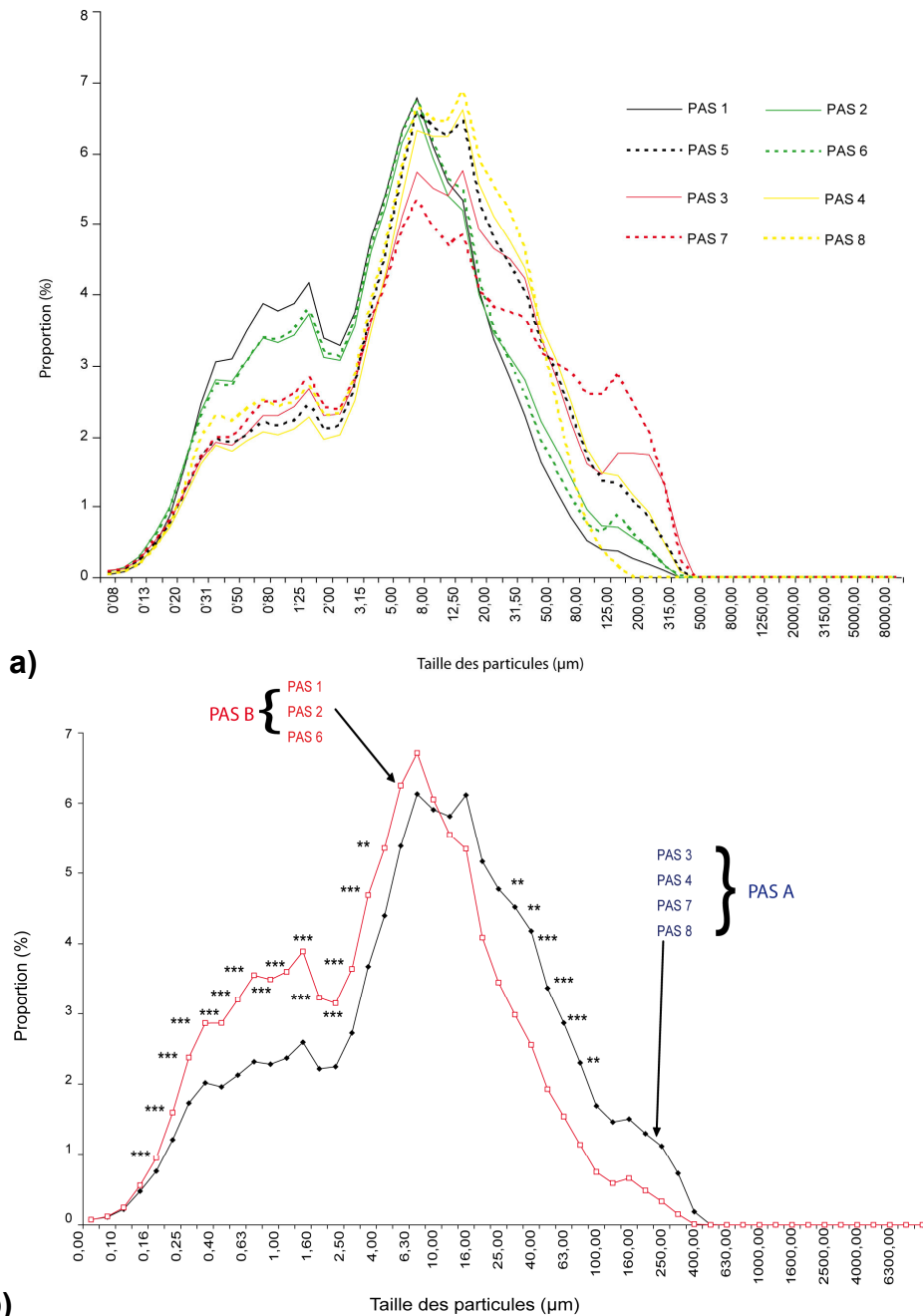
Figure III 3 : Comparaison des courbes granulométriques \mathcal{L}_2 des 8 stations de la zone de clapages PAS 1 à 8 en mai 2004. a) 8 courbes de PAS; b) Courbes moyennes des 2 classes déterminées par l'algorithme de classification par les k-moyennes.
