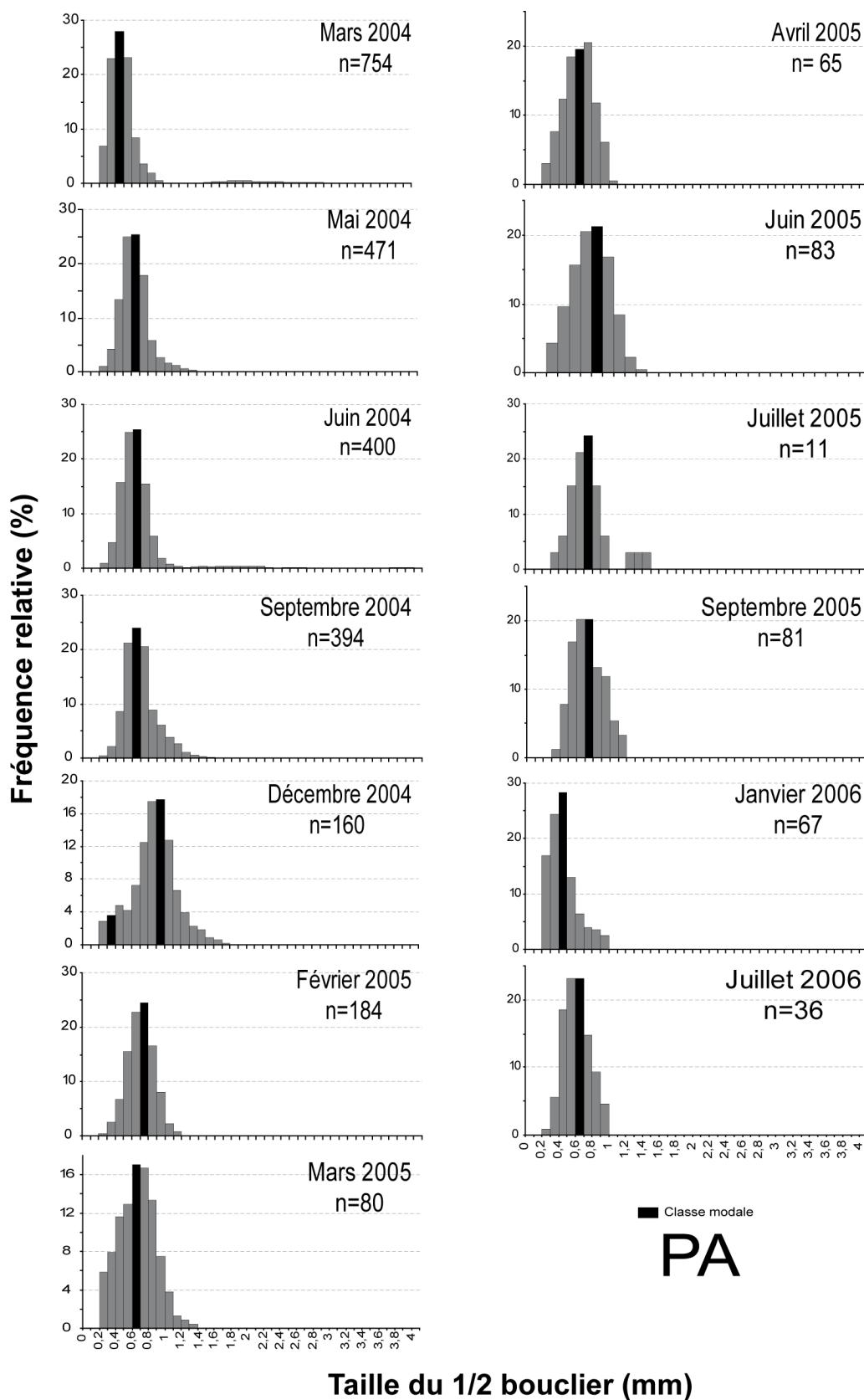
Figure IV 16 b: Histogramme de classe de taille du 1/2 bouclier ( L_{1/2} ) (mm) de Sternaspis scutata à PA. Chaque histogramme représente la distribution lissée de la fréquence relative de la largeur du demi-bouclier droit ( L_{1/2} ) (mm) dans l'ensemble des individus de chacune des campagnes (3 réplicats mélangés). L'identification des cohortes a été réalisée à l'aide de la méthode de Bhattacharya.
