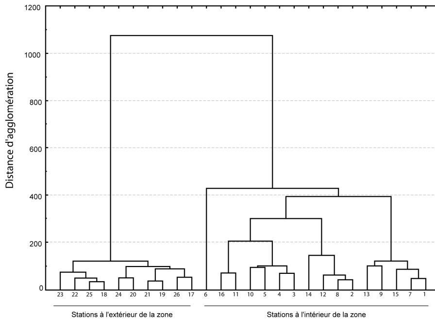
Figure II 6 : Classification hiérarchique ascendante réalisée d'après les données de Safefe Cetiis, 2005. Méthode d'agrégation : Ward basée sur la distance euclidienne. En fonction de l'ensemble des espèces présentes dans le peuplement en données brutes (densité ind / 0,3 m 2 ).
