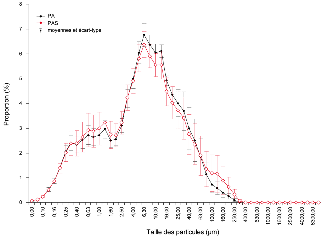
Figure III 4 : Comparaison des courbes \mathcal{L} moyennes \pm écart-type des prélèvements de PAS 1 à 8 et de l'ensemble des prélèvements de PA.
