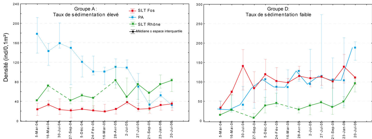
Figure IV 26 : Variations de l'abondance (ind / 0,1 m 2 ) des taxa à SLT Fos, PA et SLT Rhône, sur l'ensemble de la période d'étude, en fonction de leur résistance à la sédimentation selon Hermand et al. (2008). Le groupe A rassemble les espèces plus abondantes à proximité du Rhône (sédimentation élevée). D regroupe celles qui sont abondantes à plus de 10 km de l'embouchure (sédimentation faible).
