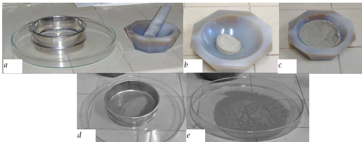
Figure II 11 (a à e) : étapes successives de la préparation des prélèvements de sédiment avant toute analyse. a) matériel nécessaire, un tamis (250 \mu\text{m} ) et un mortier; b) aspect du sédiment lyophilisé avant broyage; c) sédiment en cours de broyage; d) l'homogénéisation du sédiment par tamisage; e) le sédiment est prêt.
