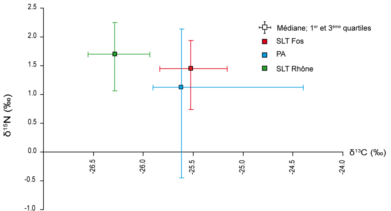
Figure III 12 :(a) Graphe des valeurs médianes et 1 er et 3 ème quartiles sur les deux premiers centimètres du sédiment des \delta^{13}\text{C} et \delta^{15}\text{N} à SLT Fos, PA et SLT Rhône
