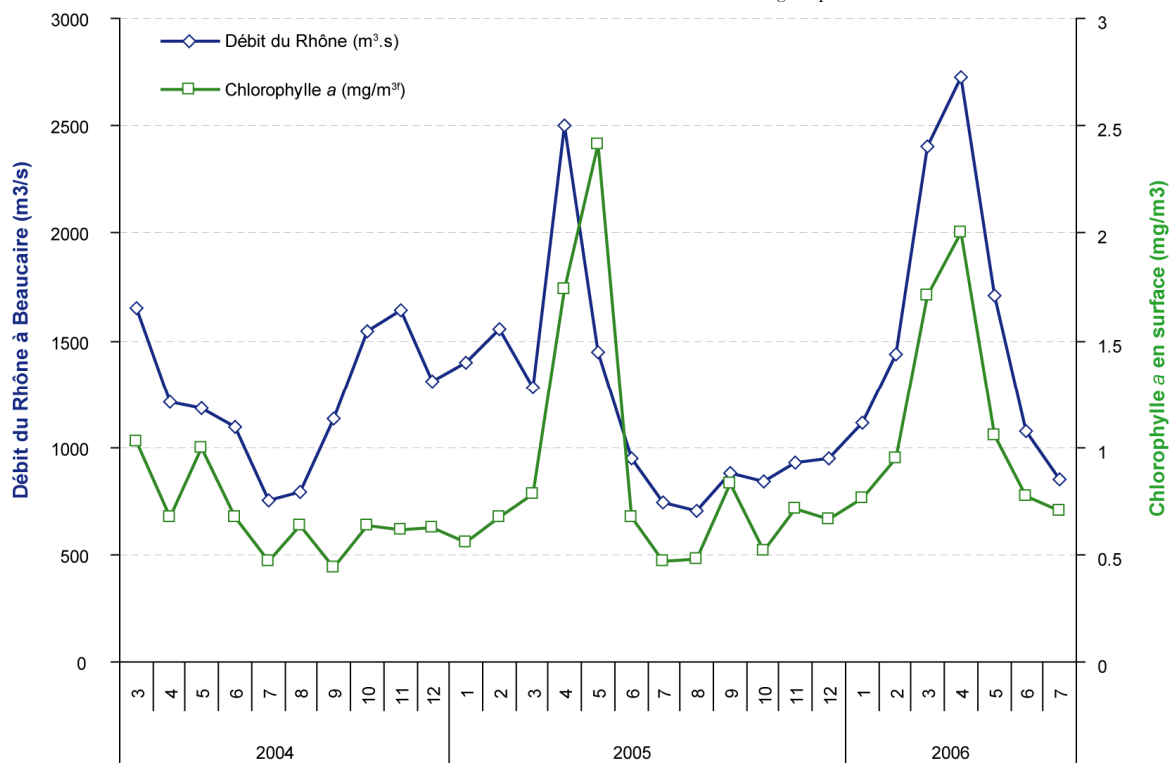
Figure III 25 : relation entre le débit moyen mensuel du Rhône et les mesures des concentrations en chlorophylle a en surface. Sources : (1) débit du Rhône : Compagnie Nationale du Rhône; (2) Chlorophylle a : Données du satellite SEA-WIFS : www.giovanni.gsfc.nasa.gov = moyennes sur la zone [Latitude = [43.0N,45.0N], Longitude = [4.0E,6.0E]].
