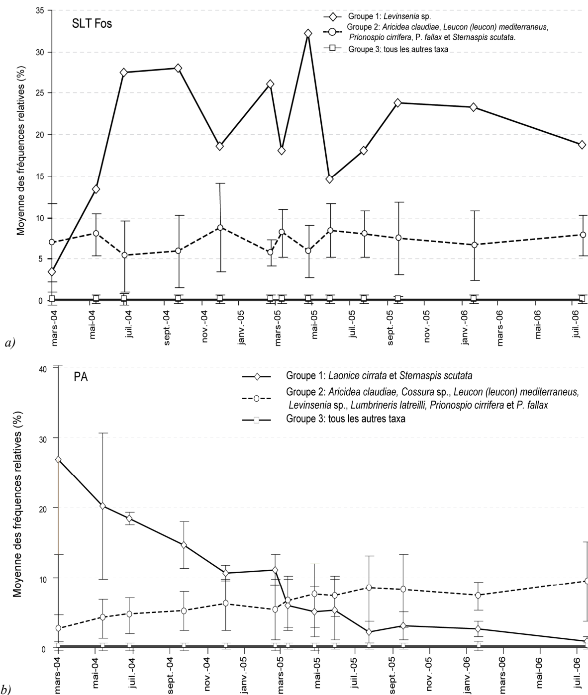
Figure IV 10 a et b : Variations temporelles de la moyenne des fréquences relatives des trois groupes d'espèces issus de l'algorithme de classification des k-moyennes à SLT Fos (a), PA (b). Moyenne ± écart-type.
