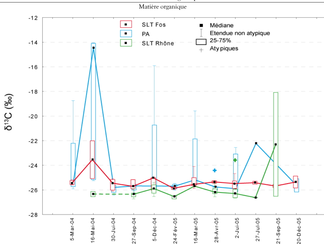
Figure III 12 b) Variation temporelle de \delta^{13}\text{C}(\text{‰}) à SLT Fos, PA et SLT Rhône.
