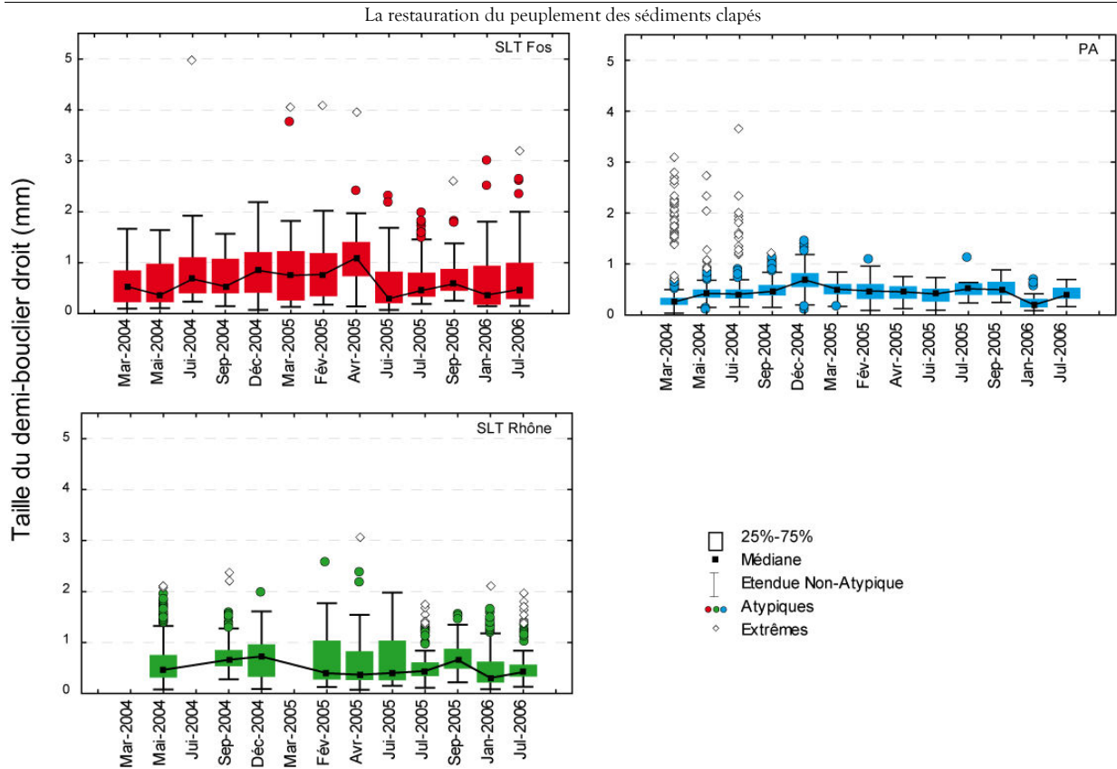
Figure IV 14 : Distribution des largeurs du demi-bouclier droit L_{1/2} (mm) à SLT Fos, PA et SLT Rhône au cours de la période d'étude.
