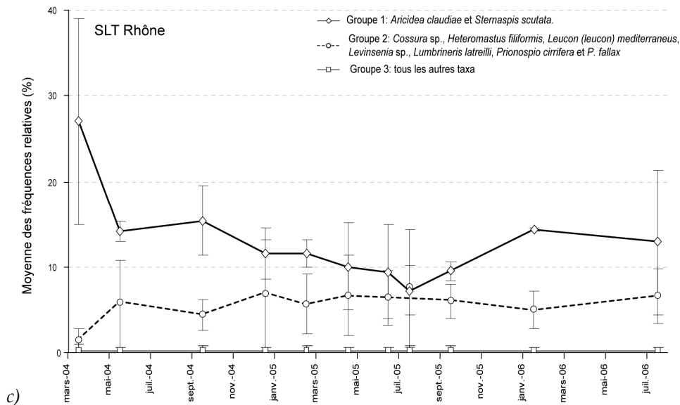
Figure IV 10 c : Variations temporelles de la moyenne des fréquences relatives des trois groupes d'espèces issues de l'algorithme de classification des k-moyennes à SLT Rhône (c). Moyenne \pm écart-type.
