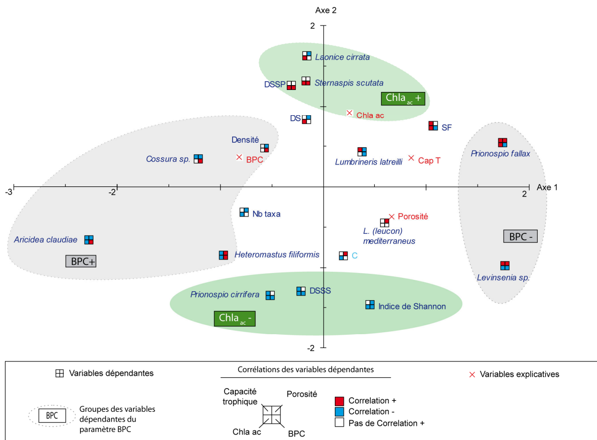
Figure IV 21 : Analyse Factorielle des Correspondances réalisées à partir des valeurs de \beta obtenues lors de l'analyse des régressions multiples. CapT : Capacité trophique; Chla ac : Chlorophylle active; DSSS : Dépositivores de sub-surface superficiels; DSSP : Dépositivores de sub-surface Profonds; DS : dépositivores de surface; SF : Suspensivores-Filtreurs, C : Carnivores. Variabilité expliquée par les axes : Axe 1 : 47 %; Axe 2 : 31 %.
