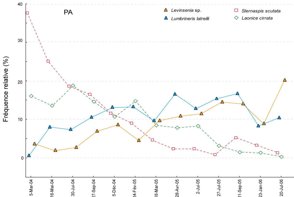
Figure IV 9 : Succession des espèces à PA de mars 2004 à juillet 2006. Fréquence relative de Levinsenia sp. , Lumbrineris latreilli , Laonice cirrata et Sternaspis scutata . Valeur médiane, l'espace interquartile n'a pas été figuré pour la clarté du graphe.
