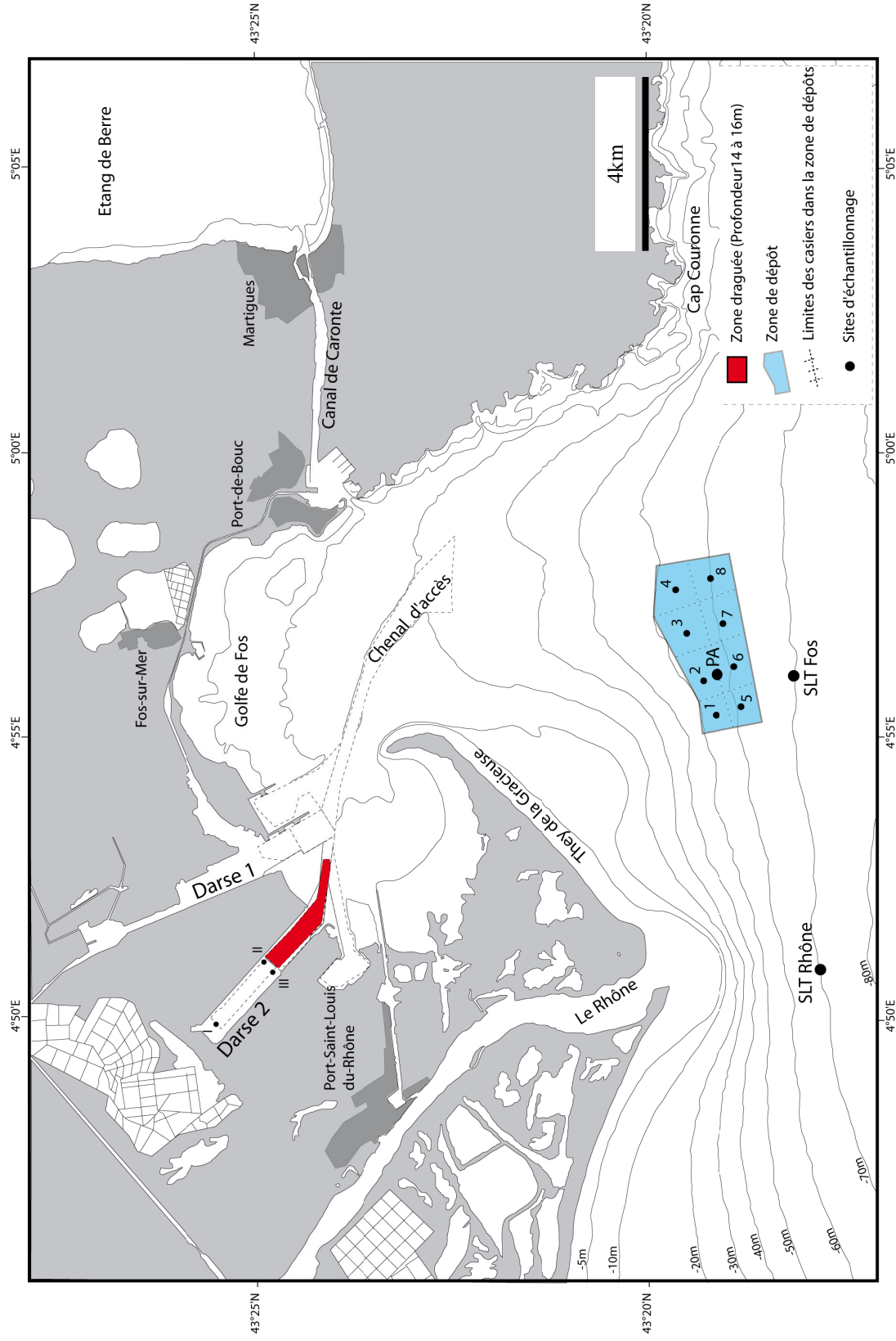
Figure II 4 : Carte de situation des points d'échantillonnage. SLT Fos, PA et SLT Rhone sont les trois stations échantillonnées régulièrement de mars 2004 à juillet 2006. I à III = Stations "Darse 2-1 à 3" échantillonnées en mars 2006. 1 à 8 = stations "PAS, 1 à 8" échantillonnées en mai 2004.
