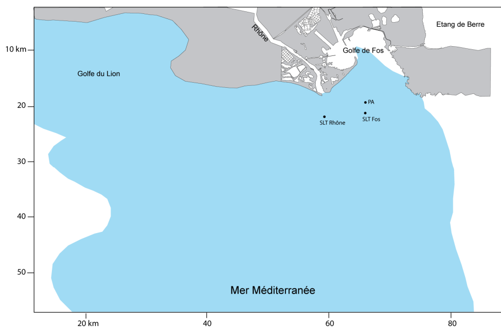
Figure II 2 : Extension maximale du panache de dilution du Rhône d'après Estournel et al. (1997; 2001). Les sites d'échantillonnage (SLT Fos, PA et SLT Rhône) sont positionnés sur cette carte afin de montrer qu'ils sont soumis à l'influence des eaux du Rhône. Les explications concernant l'échantillonnage sont présentées dans le paragraphe II.2 p30.
