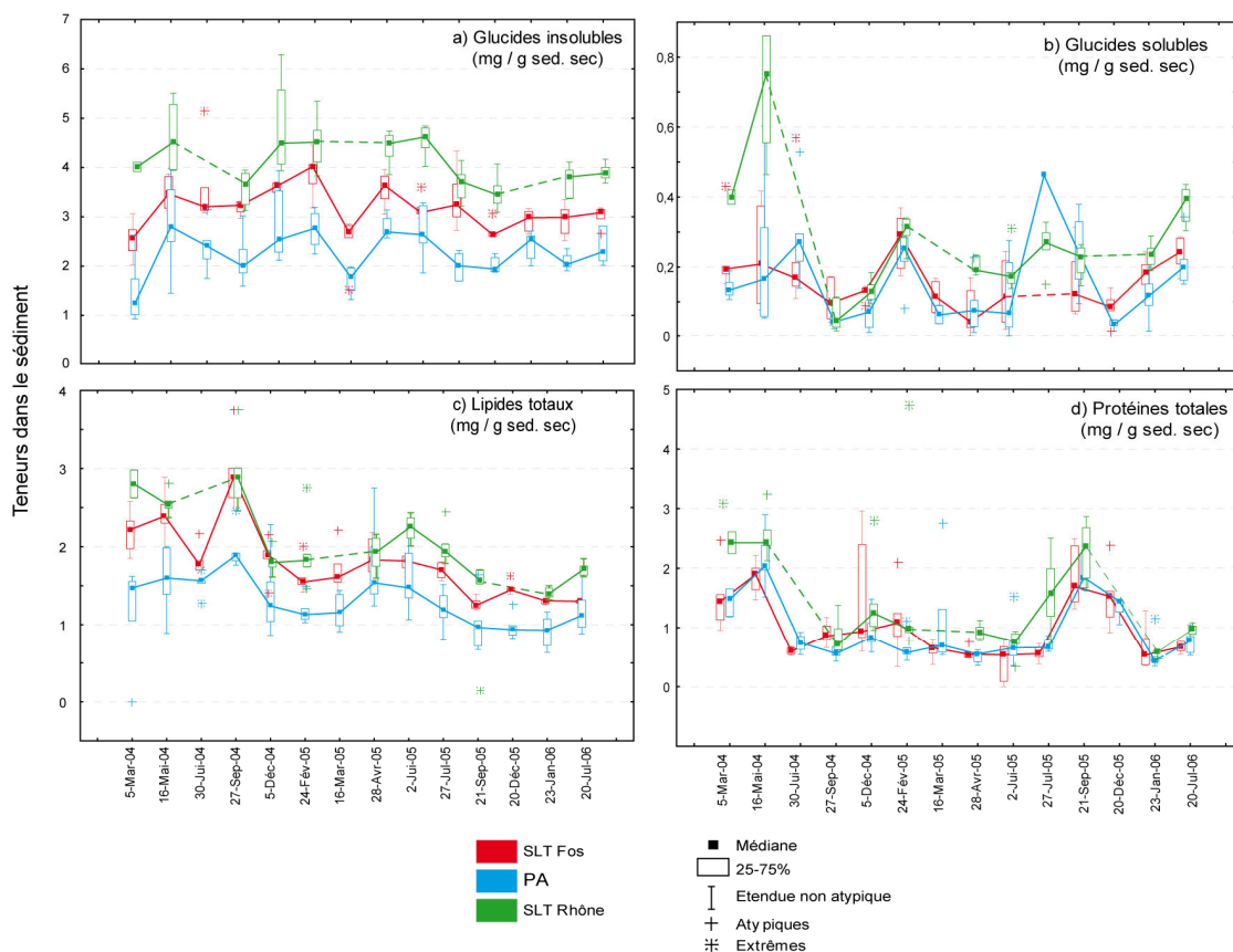
Figure III 19 : Variations temporelles des teneurs en glucides insolubles (a) et solubles (b), lipides (c) et protéines (d) à SLT Fos, PA et SLT Rhône entre mars 2004 et juillet 2006.
