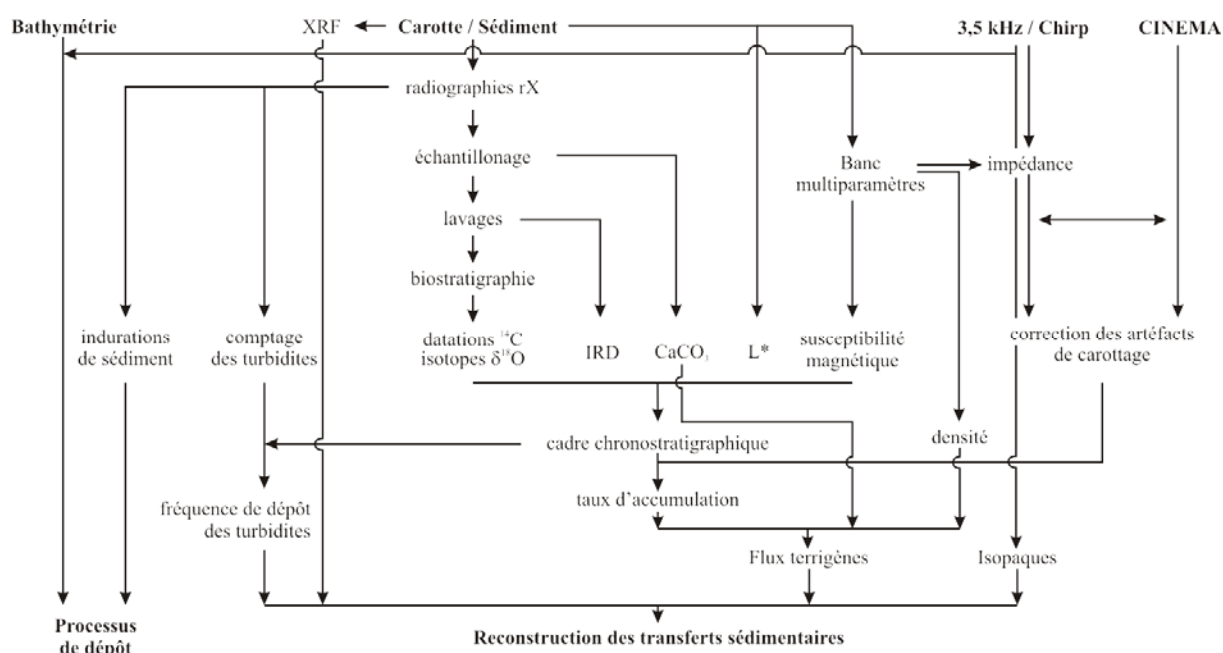
Figure IV-7. Schéma récapitulatif des outils et méthodes utilisées pour reconstruire les processus de dépôt et quantifier les transferts sédimentaires sur la Marge Nord Gascogne.
