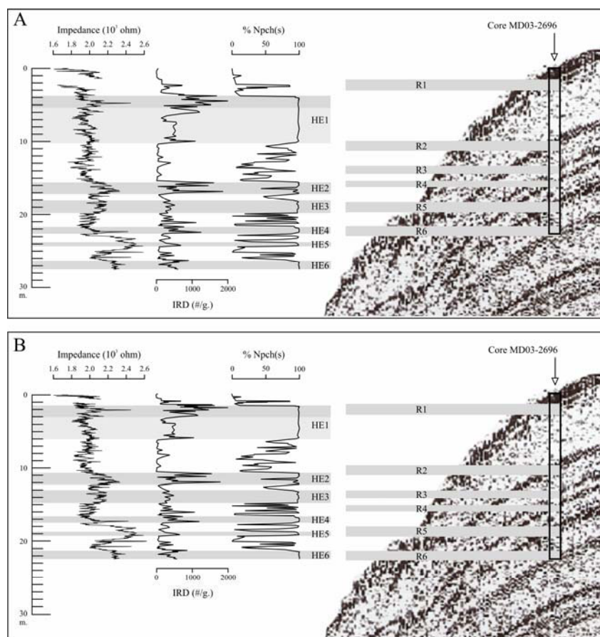
Figure IV-5. Confrontation des données de la carotte MD03-2696 avec le profil 3,5 kHz acquis sur zone, (A) avant correction des artéfacts et (B) après correction via CINEMA.
