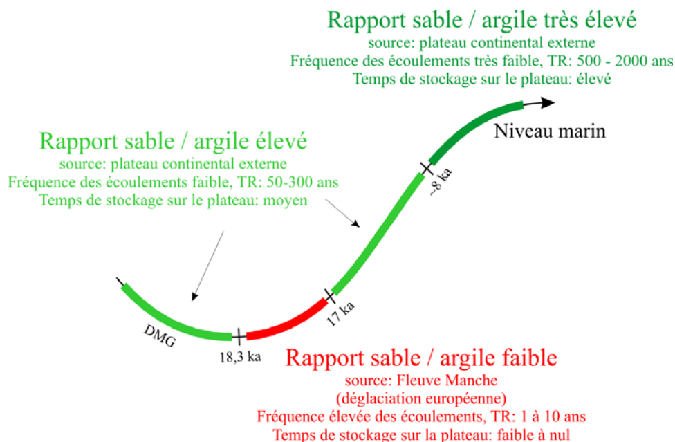
Figure V-25. Evolution des propriétés des courants de turbidité et des sources sédimentaires au cours de la transition MIS 2 – MIS 1 dans le système turbiditique Armoricaïn. TR : Temps de Réurrence des écoulements gravitaires.
