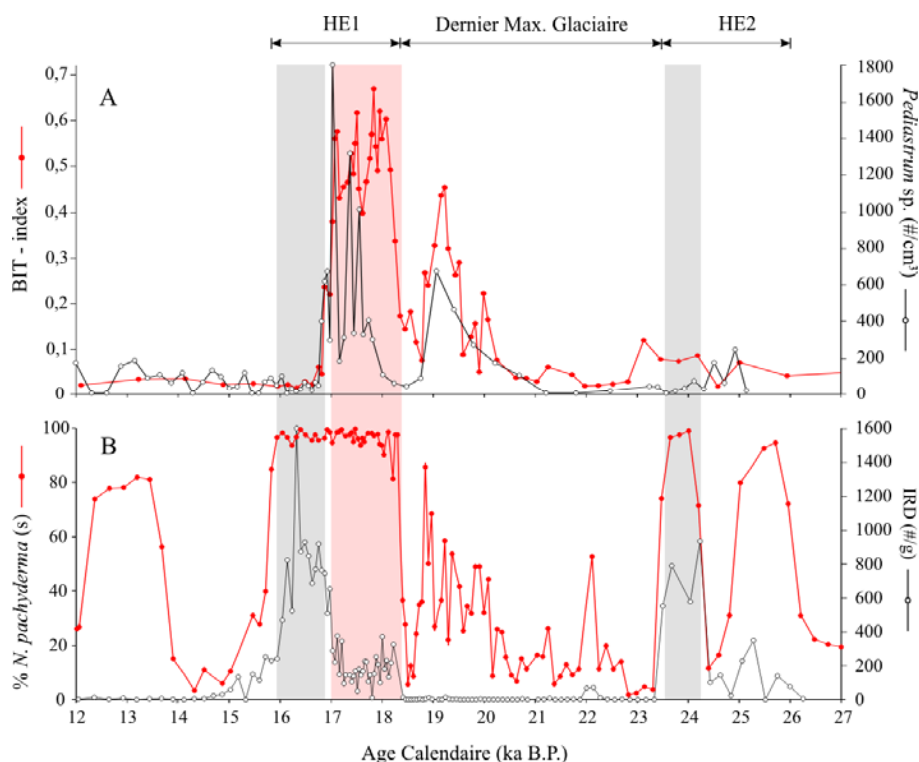
Figure V-15. Position du faciès laminé (bande rouge – 18,3-17 ka) dans la carotte MD95-2002, comparé à (A) la concentration en BIT-index (Ménot et al., 2006) et l'abondance de Pediastrum sp., et (B) la concentration en IRD et l'abondance en N. pachyderma (s) (Eynaud, 1999; Zaragosi et al., 2001b). Les bandes grises matérialisent la position du faciès à IRD.
