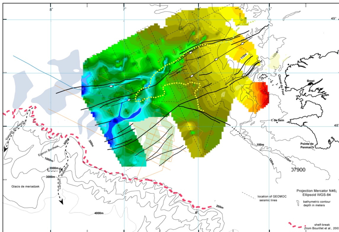
Figure I-4. Profondeur isochrone de la base de la formation de la Petite Sole et de ses paléovallées (Kervevan, 2007). La base de cette formation, érosive, affecte les formations Néogènes sous-jacentes, à savoir les formations de Jones et de Cockburn (Miocène - Pliocène) et localement le socle Crétacé. La profondeur de la base de cette formation est comprise entre 75 mstd (rouge) et 300 mstd (bleu). Le prolongement des incisions vers l'Ouest (gris) représente l'extension des paléovallées définies par Bourillet et al. (2003) et visibles dans les Figure I-1 et Figure I-8.
