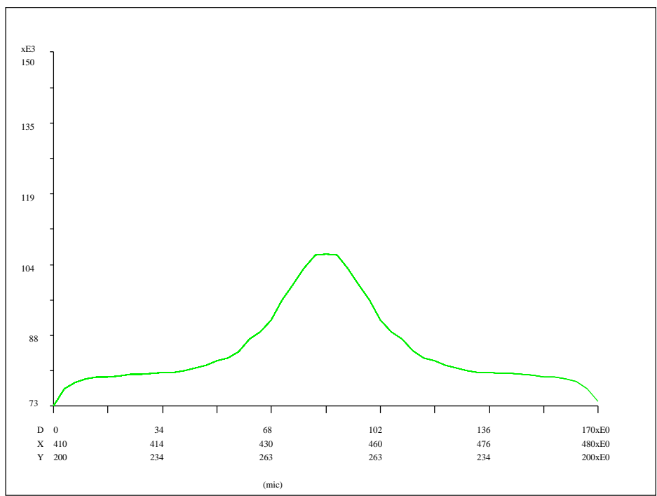
FIG. 5.10 - Simulation du champ électrostatique autour des terminaisons des cathodes pour le dessin 2.
