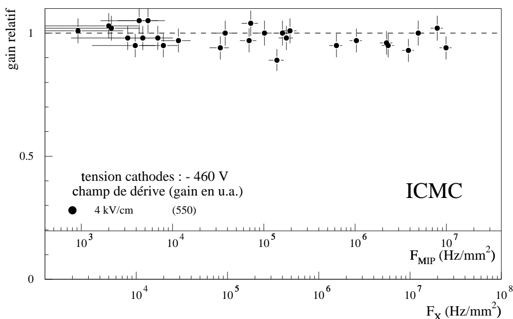
FIG. 6.20 - Couche mince ICMC (pistes Al) : variation du gain relatif en fonction du flux de rayons X ou du flux équivalent MIP. (gaz : 90% Ar + 10% DME)
