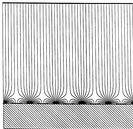
FIG. 2.4 - Lignes de champ dans une chambre gazeuse à micropistes (MSGC) [16].
