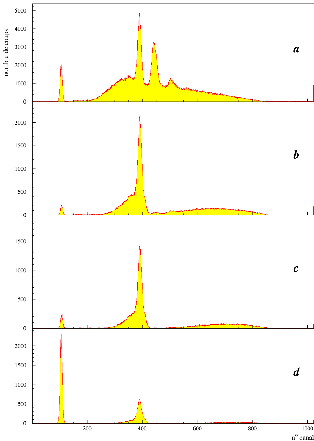
FIG. 3.12 - Spectre des rayons X émis par le canon (a), puis après avoir traversé 20 μm de cuivre (b), 30 μm de cuivre (c) et 50 μm de cuivre (d).
