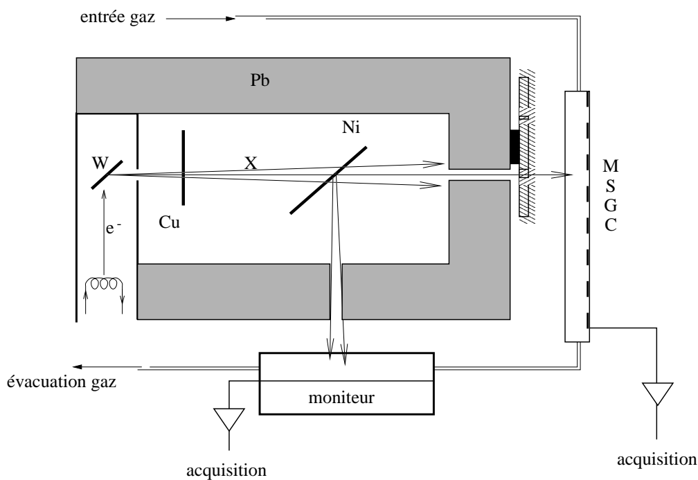
FIG. 3.11 - Banc de tests muni d'un canon à rayons X.
