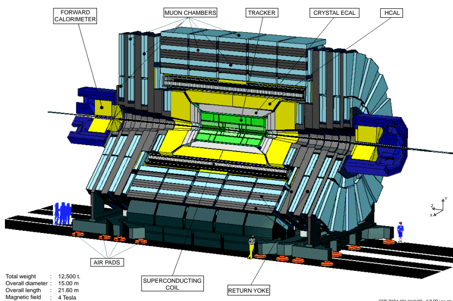
FIG. 1.7 - Détecteur CMS [10].
