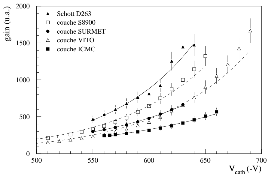
FIG. 6.12 - Gain en fonction du substrat dans les conditions de mesure : gaz 50 % Ar + 50 % DME ; tension plan de dérive -1800 V.
