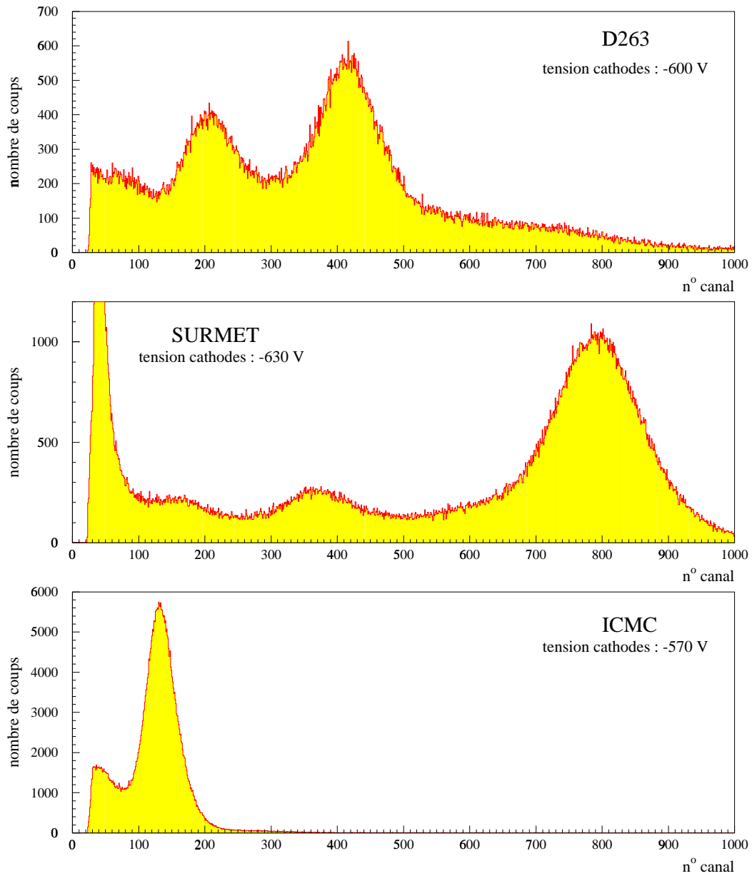
FIG. 7.7 - Spectres de la source de Fe^{55} mesurés avec les détecteurs irradiés par des neutrons, dans les conditions de mesure : gaz 50% Ar + 50% DME ; tension plan de dérive -1800 V.
