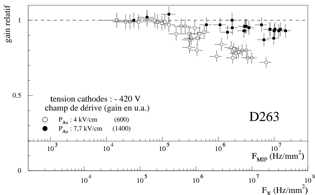
FIG. 6.16 - Verre Schott D263 (pistes Au) : variation du gain relatif en fonction du flux de rayons X pour différents champs de dérive. (gaz : 90% Ar + 10% DME)
