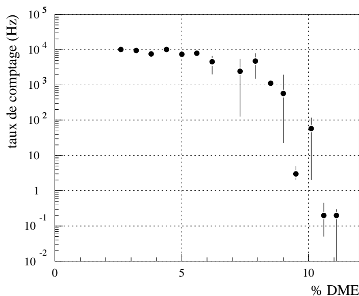
FIG. 4.1 - Taux de comptage des signaux dus à une source de Fe^{55} , dans un détecteur à micropistes en fonction du pourcentage de DME dans le mélange Ar + DME, à tensions fixées.
