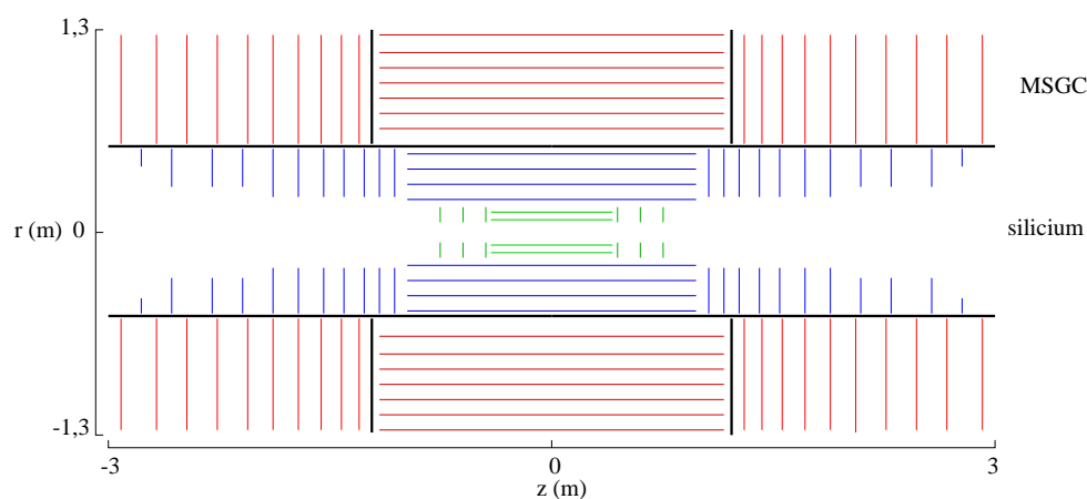
FIG. 1.8 - Ensemble de reconstruction de traces interne.
