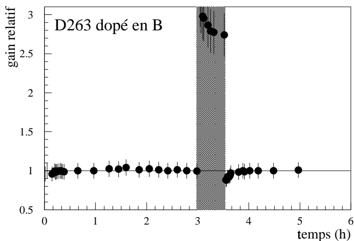
FIG. 6.5 - Conditionnement d'un détecteur réalisé sur le verre Schott D263 dopé en B par implantation.
