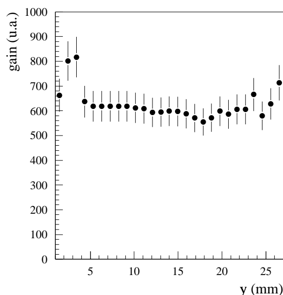
FIG. 3.17 - Mesure du gain en déplaçant la source devant le détecteur dans une direction perpendiculaire aux anodes : y .
