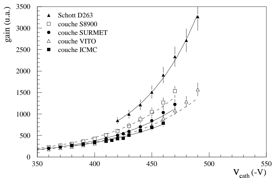
FIG. 6.13 - Gain en fonction du substrat dans les conditions de mesure : gaz 90 % Ar + 10 % DME ; tension plan de dérive -1800 V.
