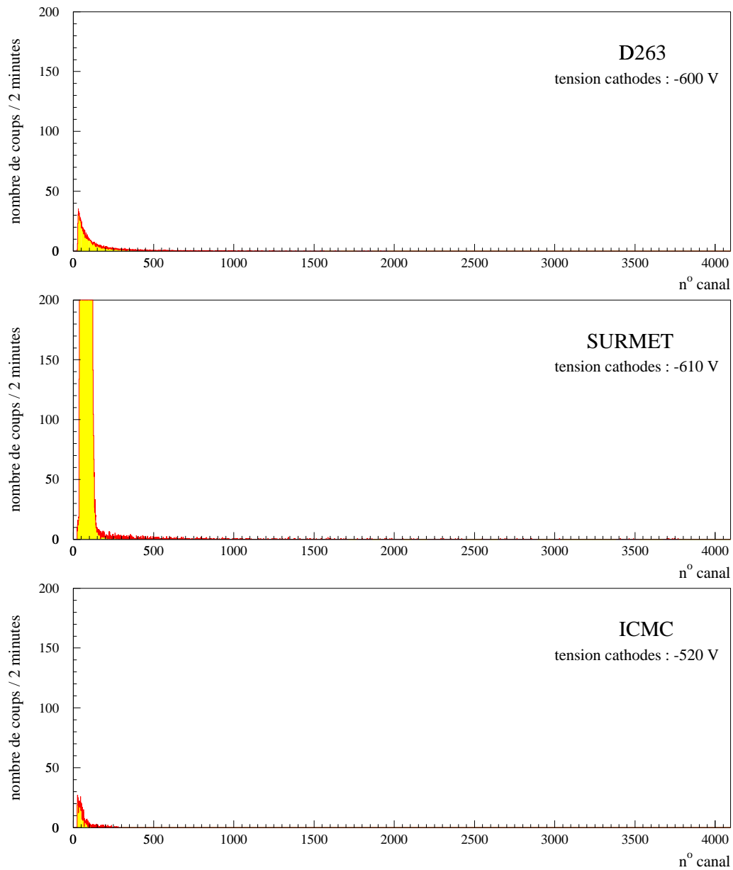
FIG. 7.9 - Spectres mesurés immédiatement après l'arrêt du réacteur, dans les conditions de mesure : gaz 50% Ar + 50% DME; tension plan de dérivation -1800 V.
