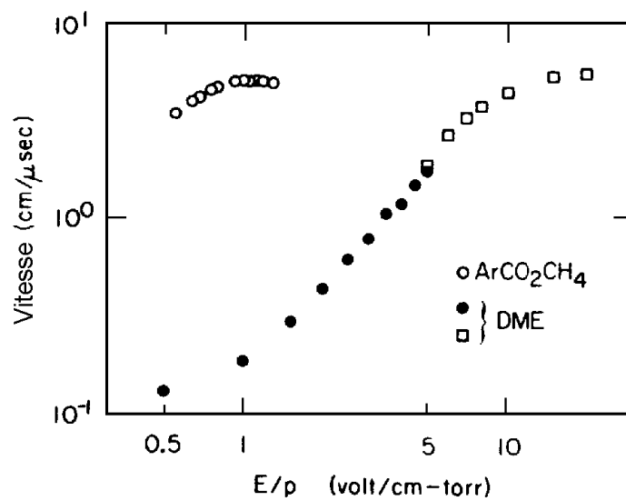
FIG. 2.9 - Vitesse de dérive des électrons dans le DME [21].
