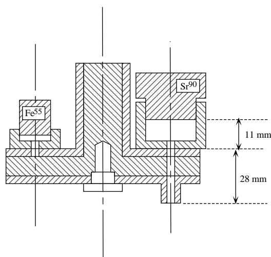
FIG. 3.9 - Système mécanique à barillets portant les deux sources de \text{Fe}^{55} et de \text{Sr}^{90} , ainsi que les différents diaphragmes de diamètre 4 mm, 1,5 mm et 0,5 mm.
