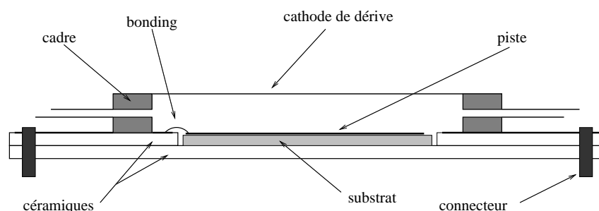
FIG. 3.5 - Détecteur monté.
