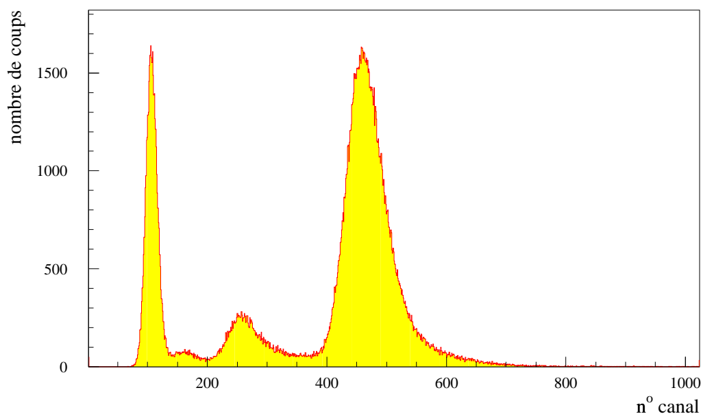
FIG. 3.18 - Spectre en énergie dû à la source de \text{Fe}^{55} mesuré avec un détecteur MSGC dans lequel circule un mélange 80 % Ar + 20 % DME. Le champ de dérive est de 4 kV/cm et la tension sur les cathodes est de -480 V.
