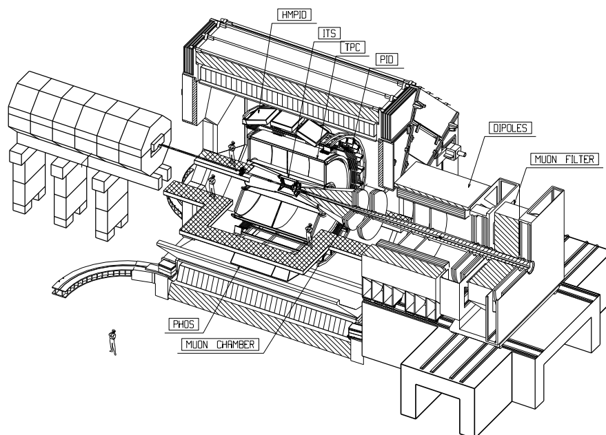
FIG. 1.4 - Détecteur ALICE [8].
