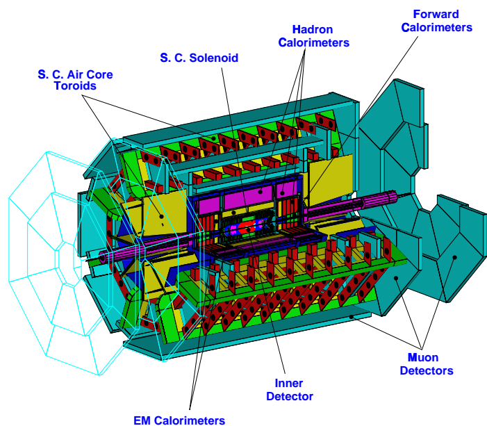
FIG. 1.5 - Détecteur ATLAS [9].
