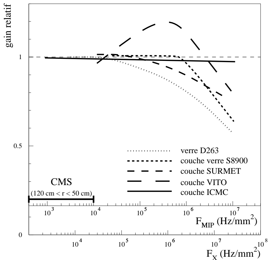
FIG. 6.21 - Gain relatif en fonction du flux de rayons X.
