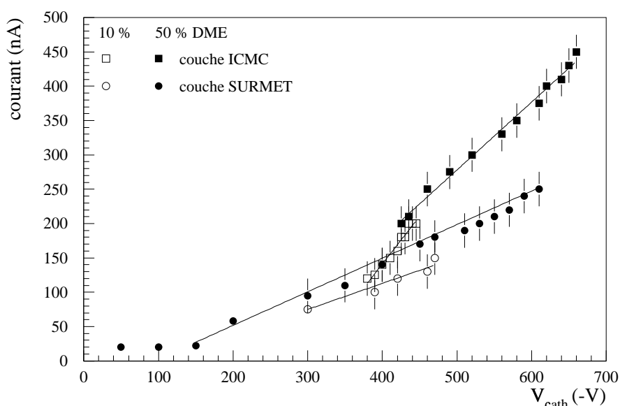
FIG. 6.14 - Courant sur les cathodes en fonction du substrat dans les conditions de mesure : gaz Ar + DME ; tension plan de dérive -1800 V.
